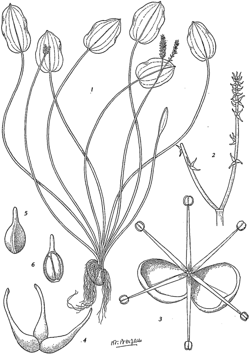
Pl. 1. — Aponogeton Decaryi Jum. emend. Bosser et van Bruggen : 1, port d'un pied femelle; 2, inflorescence femelle grossie; 3, fleur mâle (tépalés de 2 mm de long); 4, fleur femelle (carpelles de 5 mm de long environ); 5, jeune fruit; 6, coupe de ce jeune fruit montrant les 2 graines.
