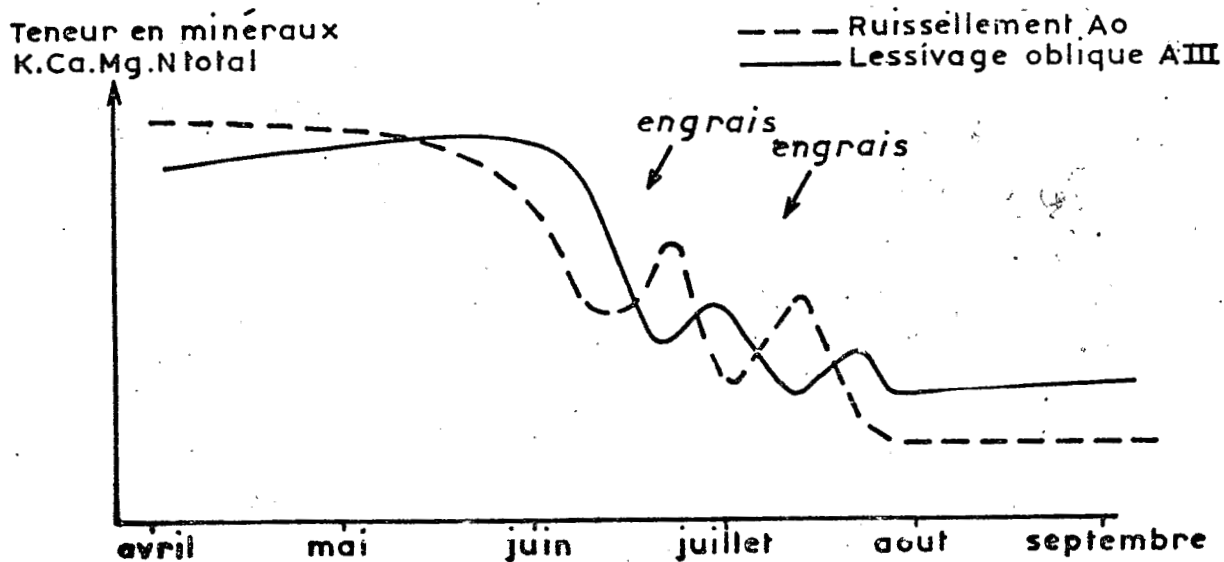
Fig. n° 2.- Schéma de l'évolution des teneurs en minéraux des eaux de ruissellement Ao et de lessivage oblique (AIII) au cours de la grande saison des pluies.
