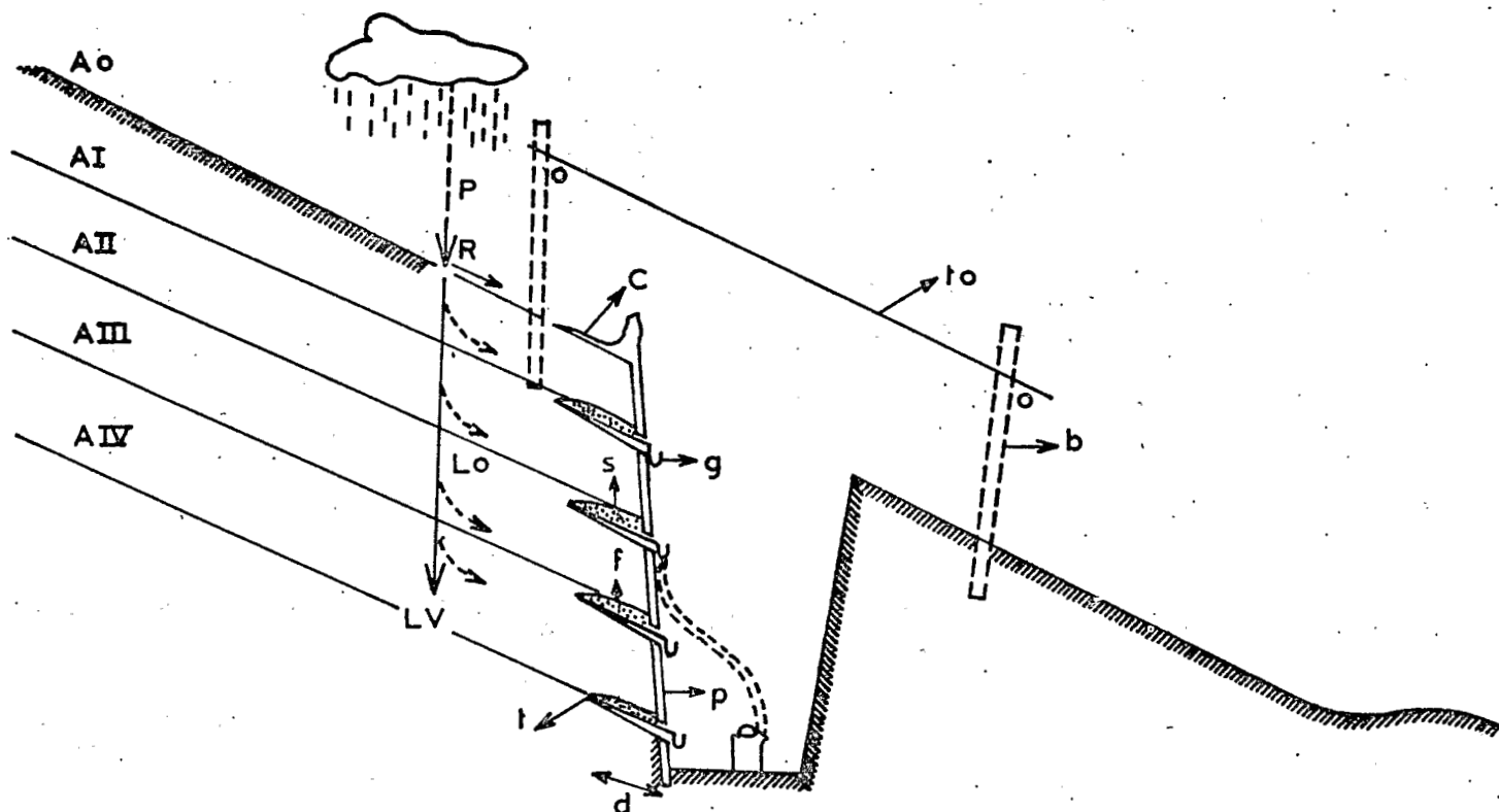
Fig. n° 1 - Schéma des mouvements de l'eau de gravité et d'une case de lessivage oblique; P = pluie; R = ruissellement; LV = lessivage vertical; Lo = lessivage oblique; AI, II, III, IV = horizon pedologique; C = canal du ruissellement; g = gouttière; t = tête; f = fente; s = sable lavé; d = tranche de sol protégée par le canal c et la tôle to; b = bâti qui soutient le toit to; p = planche.
