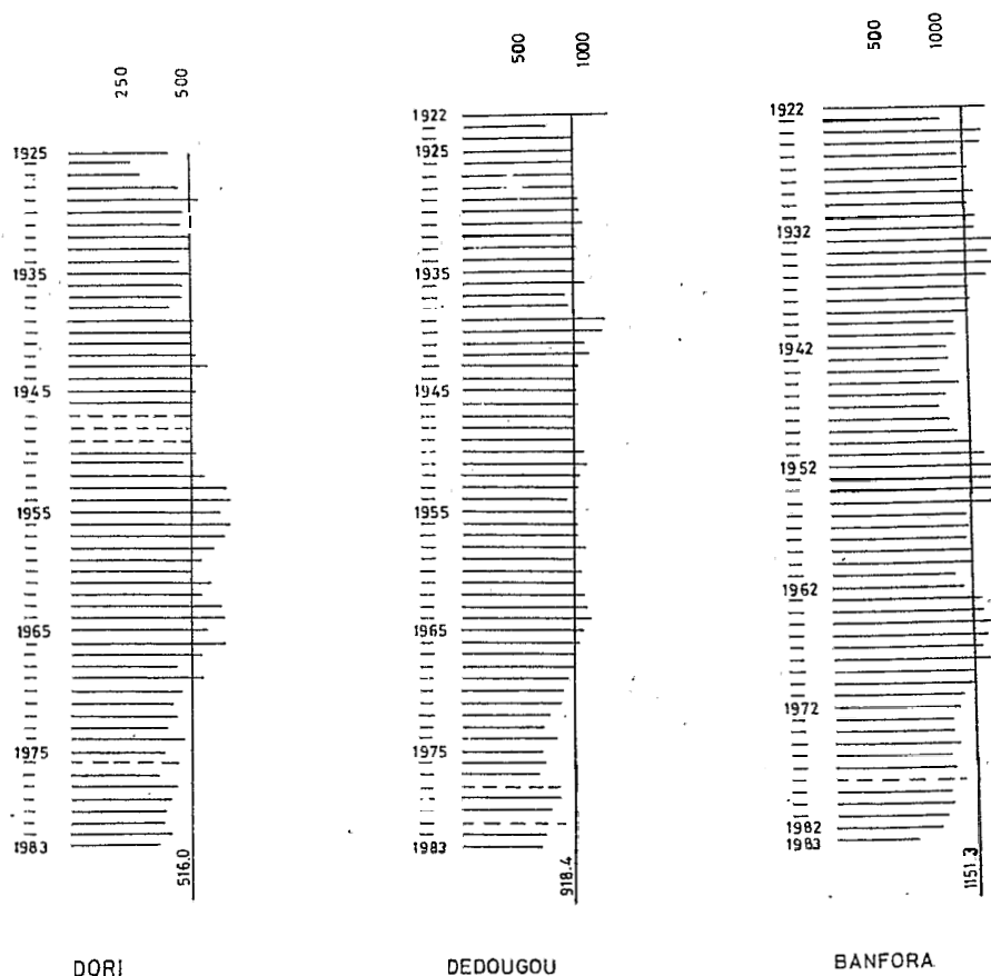
FIGURE 3 - MOYENNES MOBILES PONDEREES DES PLUVIOMETRIES ANNUELLES POUR TROIS STATIONS CLIMATOLOGIQUES.
