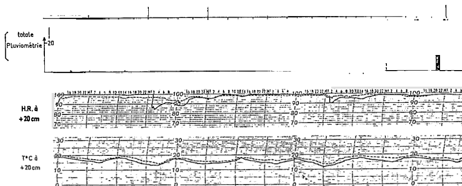
FIG. 5. — Microclimats comparés à 1 300 m (forêt humide de moyenne altitude) et 1 400 m (forêt sclérophylle de montagne), dans le massif du Marojezy.
