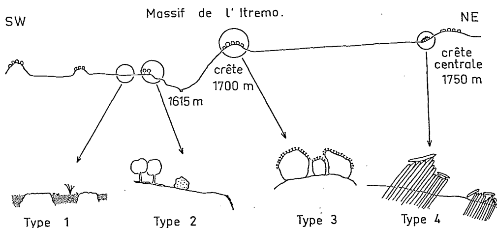
FIG. 11. — Principaux types de biotopes dans la zone rocheuse de l'Itremo.
