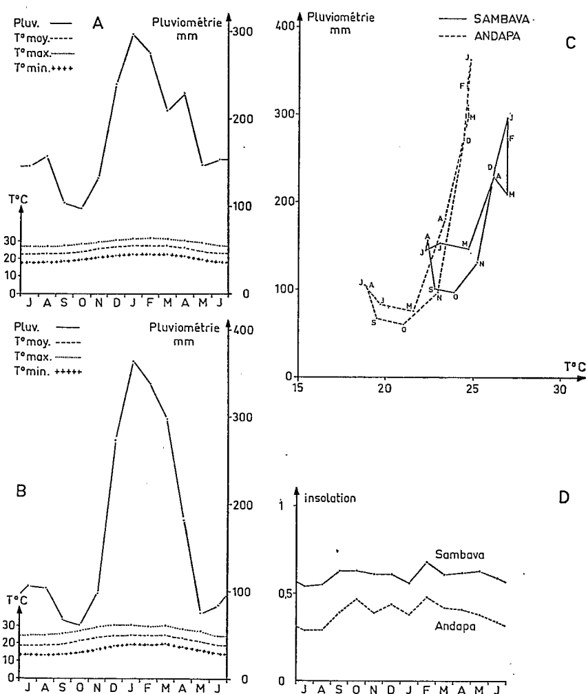
FIG. 4. — A. Diagramme ombrothermique de la station de Sambava. B. Diagramme ombrothermique de la station d'Andapa. C. Climatogramme pluviothermique de ces deux stations. D. Rapport durée d'insolation : durée du jour de ces deux stations.
