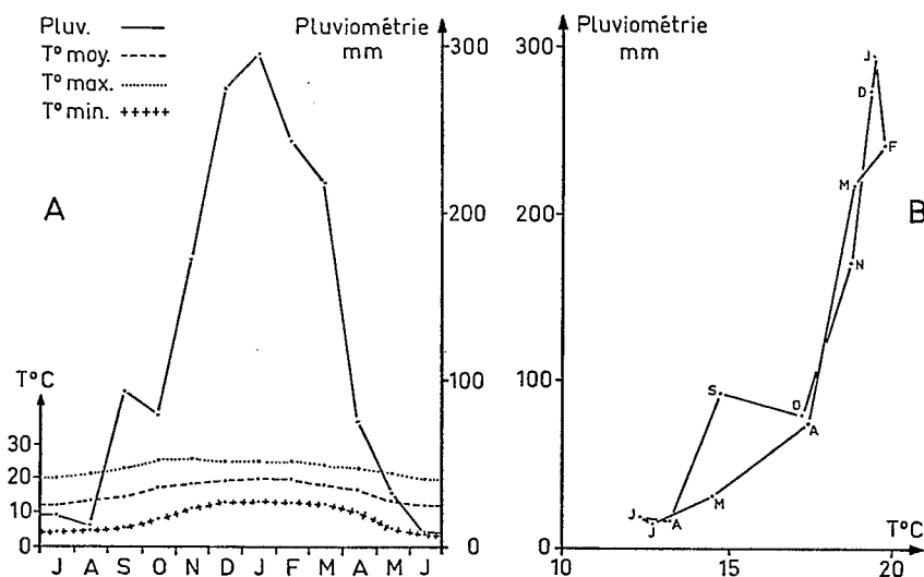
FIG. 9. — Diagramme ombrothermique et climatogramme pluviothermique de la station d'Antsirabe, près du massif de l'Ibity.
