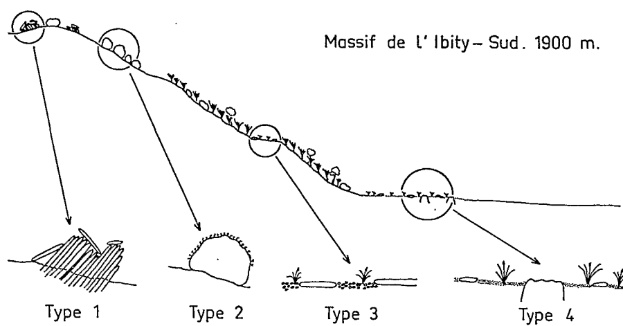
FIG. 12. — Principaux types de biotopes dans la zone rocheuse de l'Ibity-Sud. 1. Lames d'itacolumite. 2. Rochers de quartzite recouverts de lichens fruticuleux. 3. Pavage de quartzite, grains grossiers de quartzite et Graminées, au milieu de la végétation arbustive. 4. Sable grossier, pavage de quartzite, rochers affleurants et Graminées, en prairie altimontaine.
