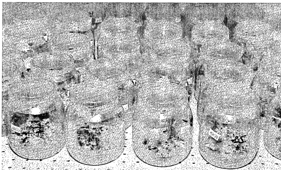
FIG. 4. — Embryogenèse adventive (Adventive embryogenesis).
