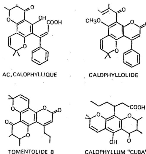
Figure 1 • Structures de l'acide calophyllique, du calophyllolide, du calophyllum "cuba" et du tomentolide B utilisés pour les tests comparatifs de toxicité in vitro .
