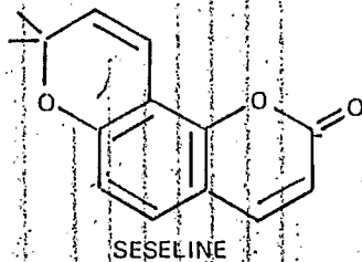
Figure 3 • Structures de la séséline (C 14 H 12 O 3 ).
