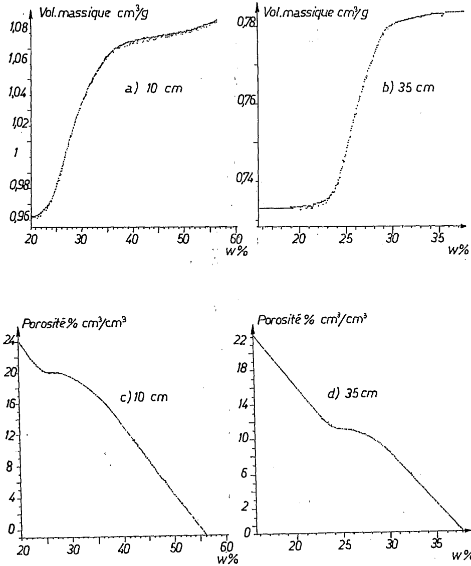
Figure 4 : Exemple de courbes de retrait (a, b) et de porosité ouverte à l'air (c, d), calculées à partir des courbes de rétraction à la figure 3.
