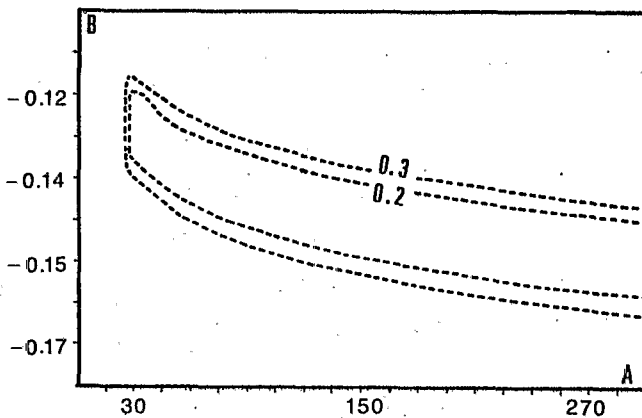
Figure 4 Représentation partielle de la région exacte de confiance des paramètres A et B aux seuils approchés de 5% (somme des carrés critiques = S.C.C. = 0,2) et de 1% (S.C.C. = 0,3). On remarquera que l'estimation de B est étroitement liée à celle de A.
