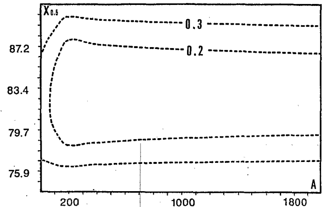
Figure 5 Représentation partielle de la région exacte de confiance des paramètres A et X_{0,5} aux seuils approchés de 5% (somme des carrés critiques = S.C.C. = 0,2) et de 1% (S.C.C. = 0,3). A la différence de ce que l'on observe dans la figure 4, X_{0,5} est pratiquement indépendant de A.
