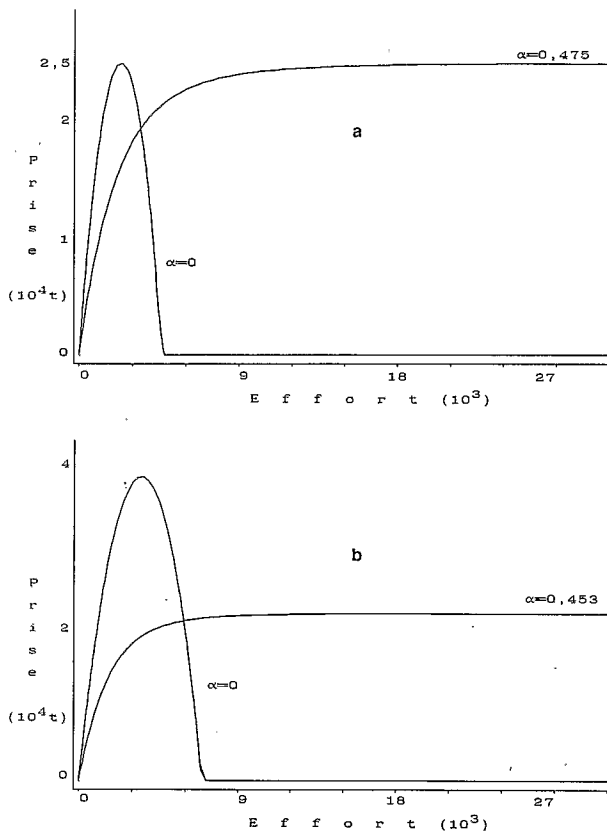
Figure 4. — Relations à l'équilibre entre prises et efforts standardisés obtenues sous l'hypothèse B_0 = B_v , selon que toute la biomasse est accessible ou non : (a) Modèle {M1}; (b) Modèle {M2}.
