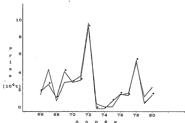
Figure 2. — Prises observées et ajustées (*) par le modèle {M1} sous l'hypothèse B_0 = B_v .
