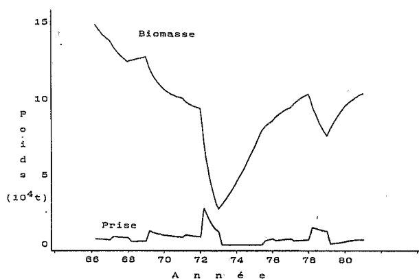
Figure 3. — Biomasse totale et captures (par cinquième d'année) de 1966 à 1980 estimées avec le modèle {M1} sous l'hypothèse B_0 = B_v .
