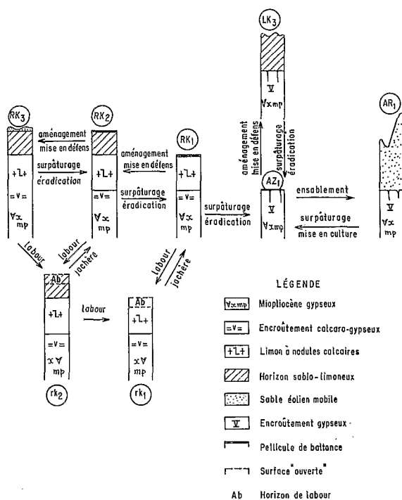
FIG. 4. — Exemples de relations entre les systèmes écologiques des steppes sableuses de la région de Zougata.
