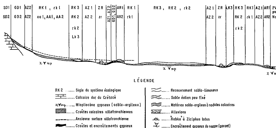
FIG. 3. — Répartition schématique des systèmes écologiques de la région de Zougrata.
