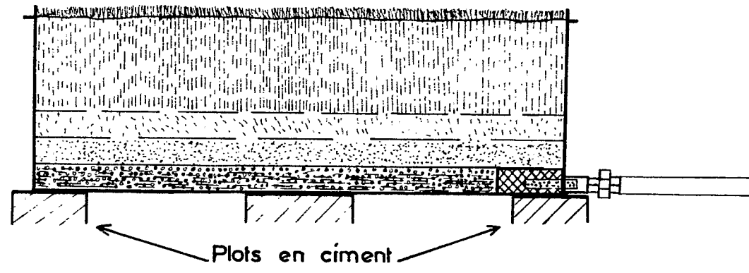
Détail de A Echelle 1/20 e
