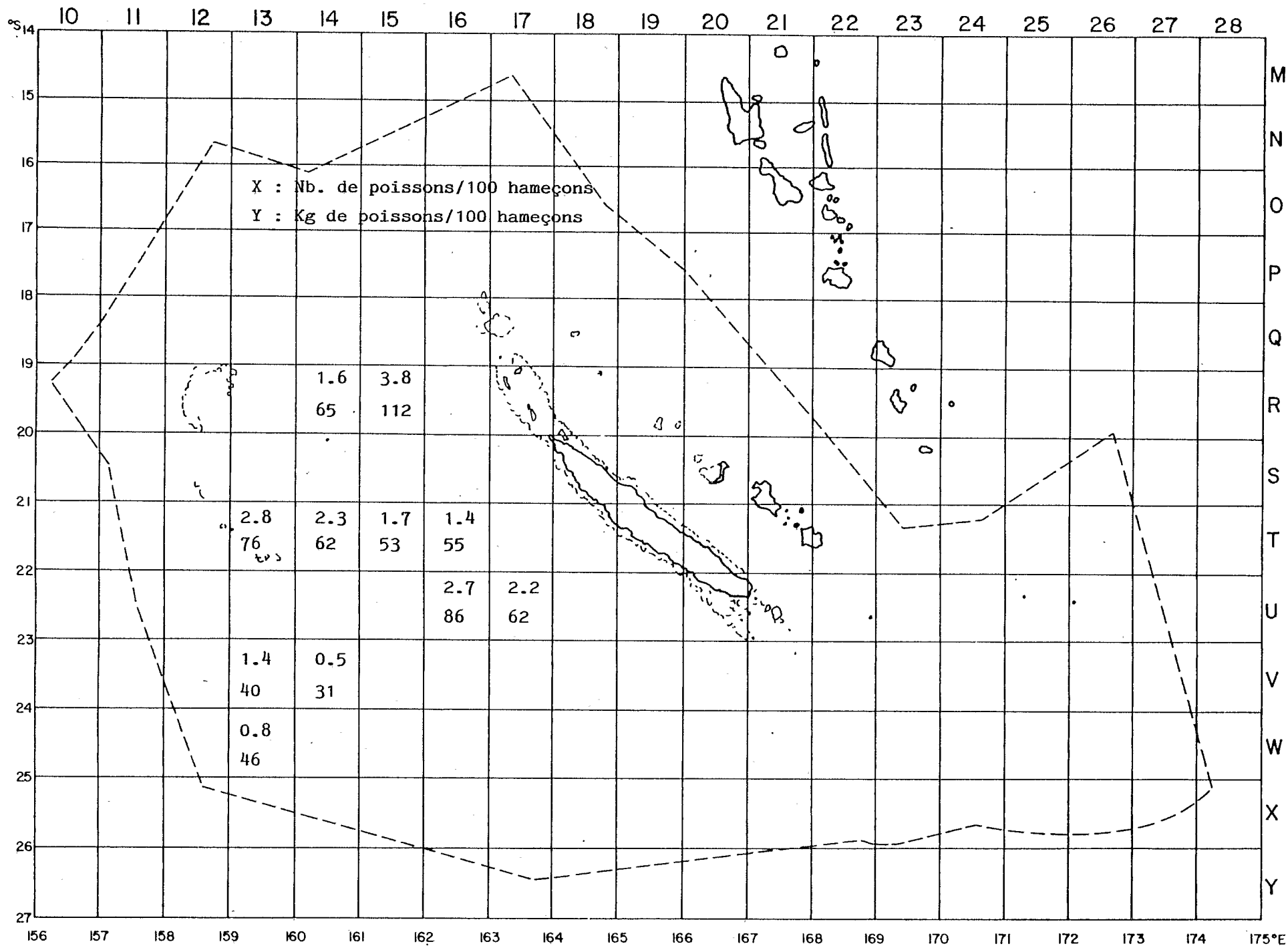
Fig. 4 - Répartition des rendements de l'OCEANIEN en novembre 1985.
