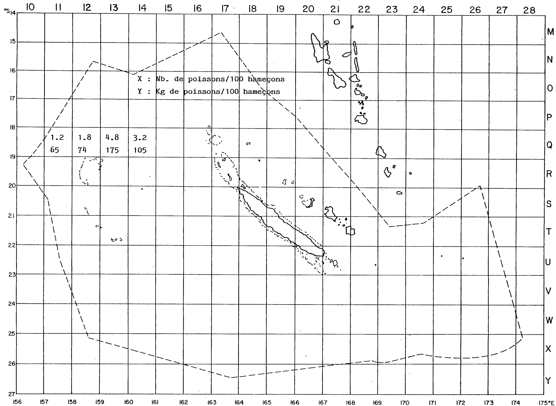
Fig. 6 - Répartition des rendements du CALEDONIE TOHO n° 1 en novembre 1985.
