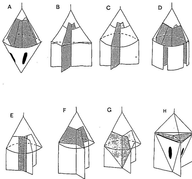
Fig. 2 : Modèles de piège : A, biconique ; B, pyramidal ; C, D, E, F, G, monoconiques (E "Vavoua", F du CRTA) ; H, bipyramidal. Partie hachurée : couleur noire ; non hachurée : couleur bleue. Le haut du piège est en tulle moustiquaire blanc.
