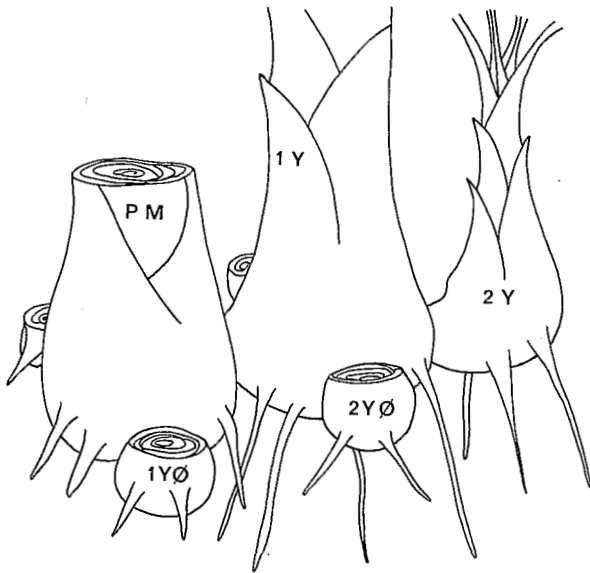
Fig. 1. Schéma de l'agencement des générations successives des rejets d'un bananier. PM = pied-mère; 1 Y = rejet de première génération; 2 Y = rejet de deuxième génération; Y Ø = rejets oeilletonnés (d'après Mateille, Cadet & Quénéhervé, 1985).
