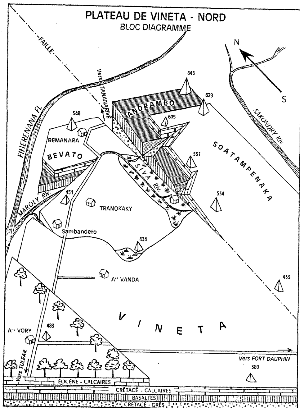
Fig. 14 — Structure du Plateau de VINETA (d'après SOURDAT, 1973)
