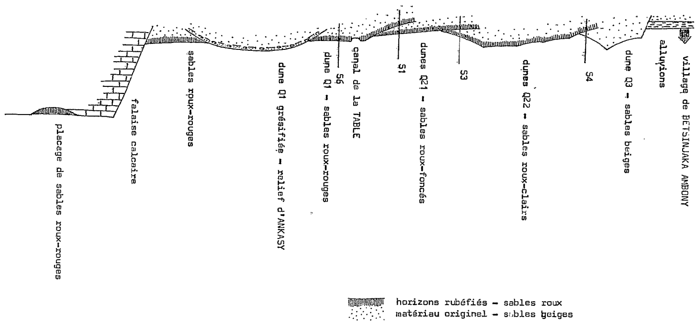
Fig. 11 - Coupe schématique E-W de la Plaine de TULEAR Emplacements des sondages
