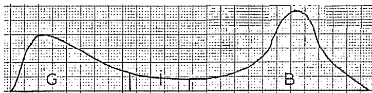
Fig. 31 — Électrophorégrammes des humus de quelques sols
