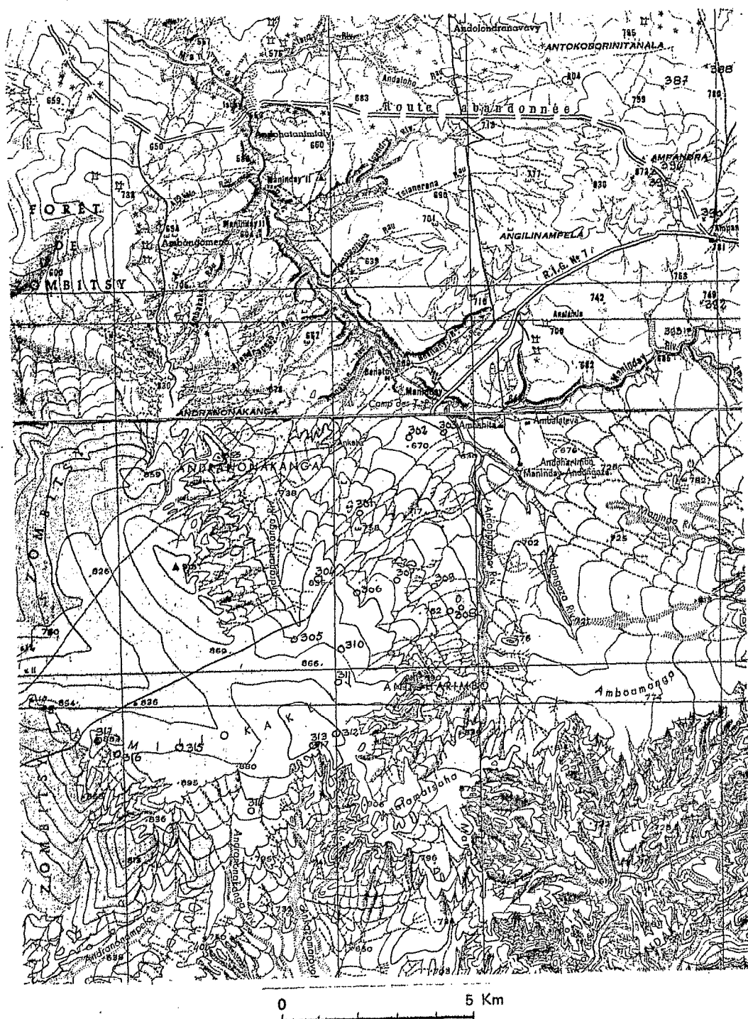
Fig. 27 — Les dômes sableux de l'ISALO, le MILIOKAKELY, l'AMPANDRA, etc. (d'après I.G.N. 1/100 000 G 56-57)
