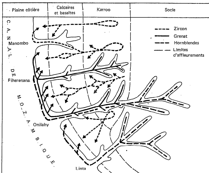
Fig. 6 - Cheminements de quelques minéraux lourds dans les bassins fluviaux et les interfluves du Sud-Ouest. (d'après SOURDAT et MAHE, 1974).
