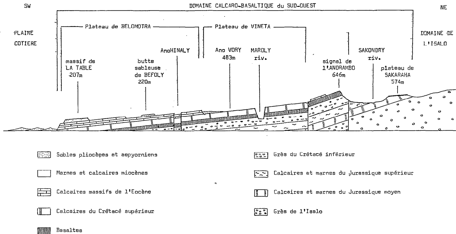
Fig. 13 - Coupe schématique du domaine calcaro-basaltique du Sud-Ouest
