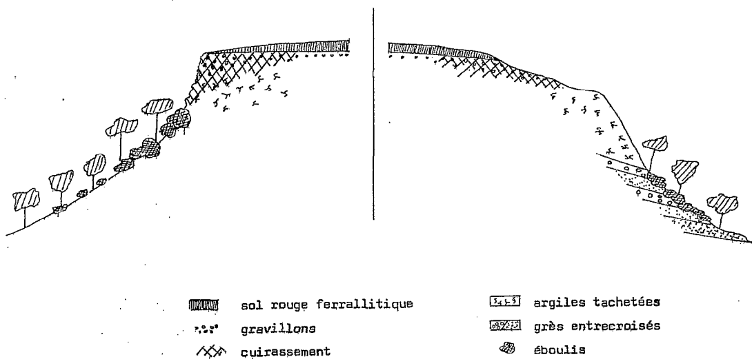
Fig. 20 - Coupe schématique de la Table de l'ANDRANOMPANGADY
