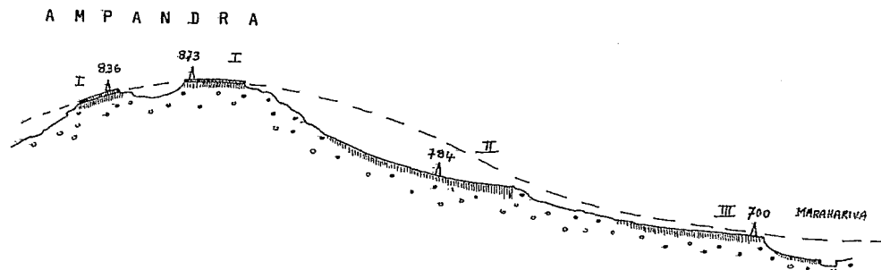
Fig. 29 - Coupe schématique du dôme d'AMPANDRA montrant la disposition des trois glacis par rapport au modelé ancien
