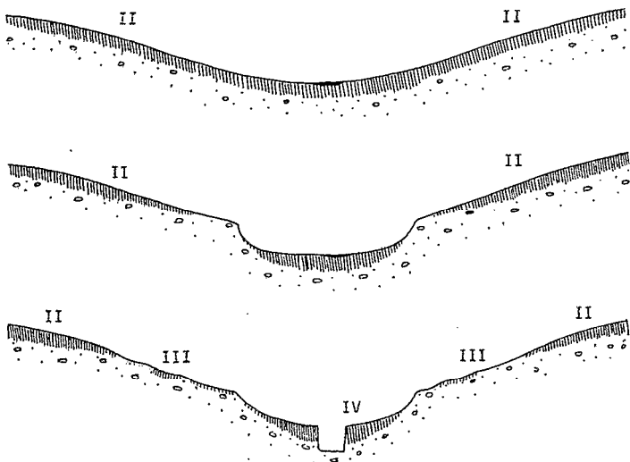
Processus d'enfoncement de la rivière AMPIO dans les glacis
