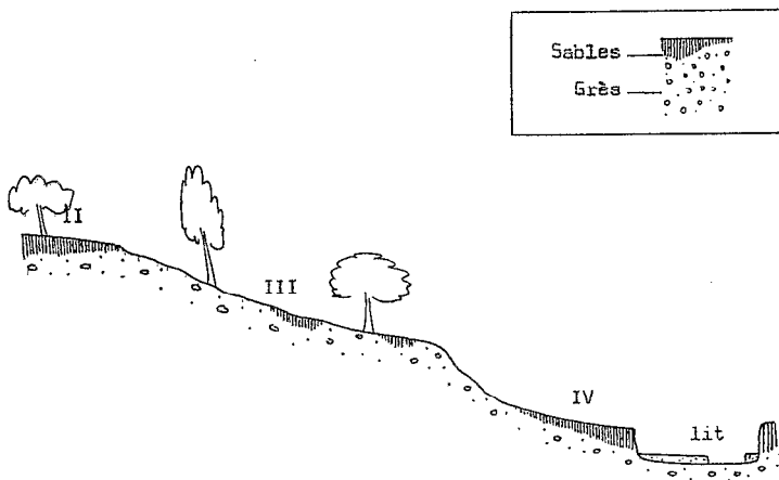
Emboitement final des glacis observé à ANDRANGLAVA en bordure du FIHENENANA.
