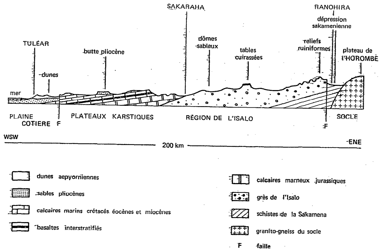
Fig. 5 - Coupe géologique schématique du bassin sédimentaire de MORONDAVA
