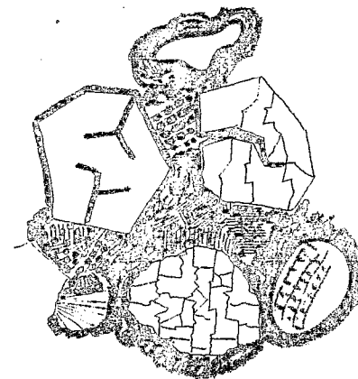
Fig. 23 - Consolidation et cuirassement des formations ferrallitiques de l'ISALO
