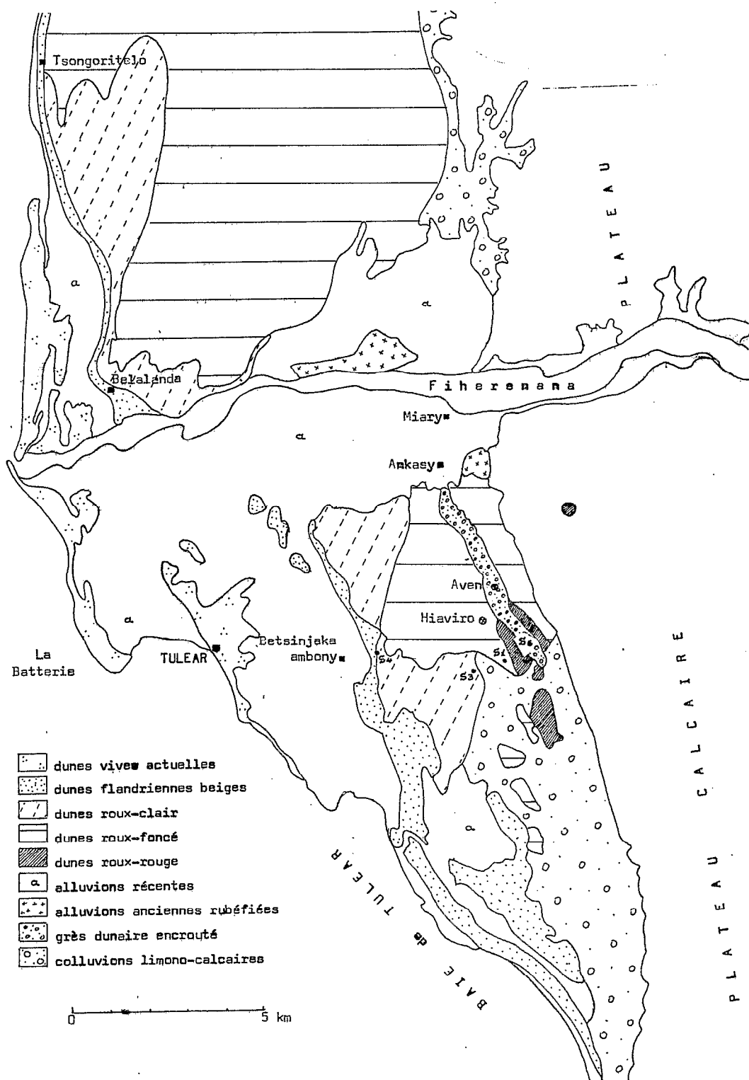
Fig. 12 - La plaine de TULEAR (d'après SOURDAT, 1970)
