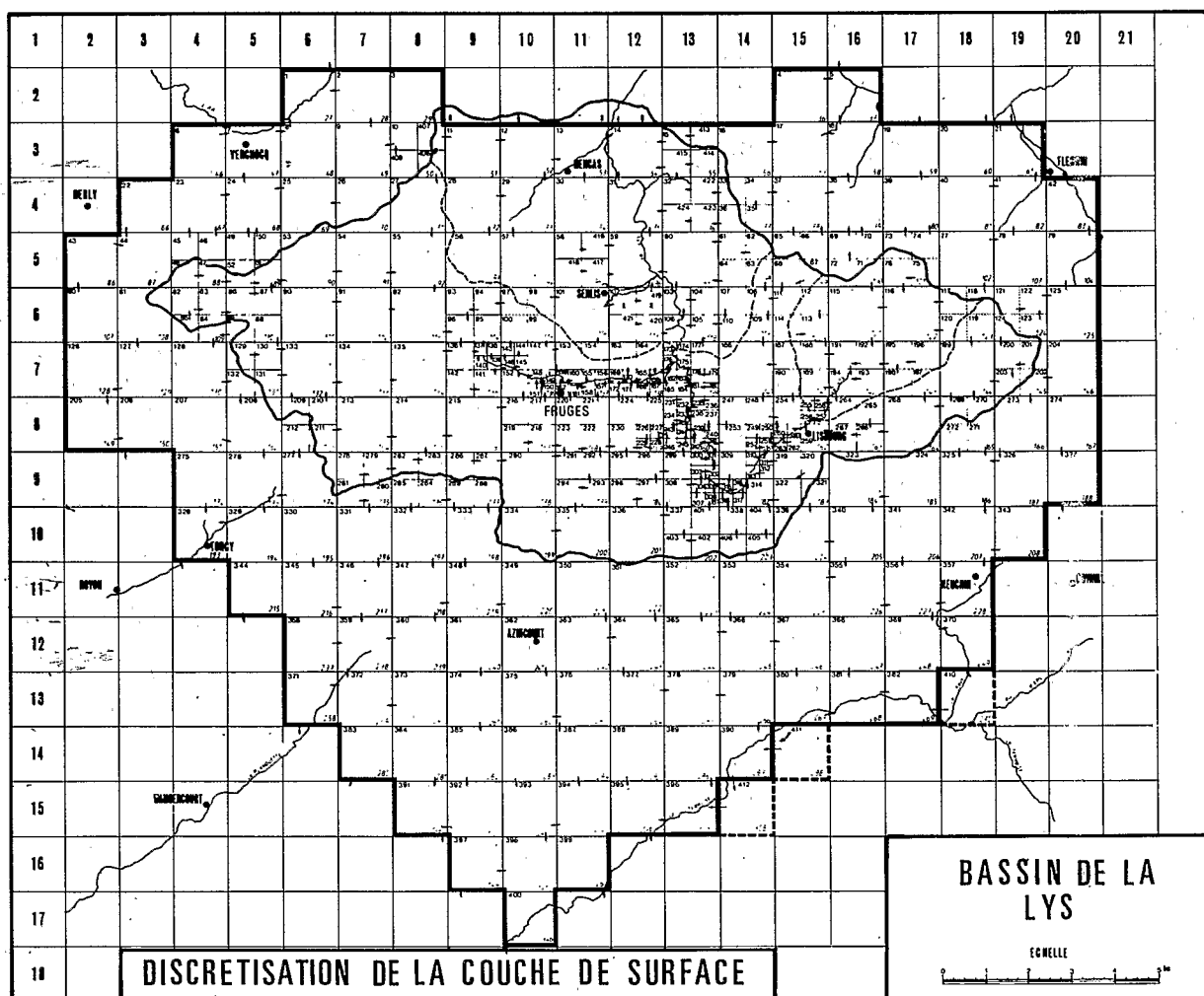
Figure 1 - Discrétisation de la couche de surface. Schéma du réseau d'écoulement.
