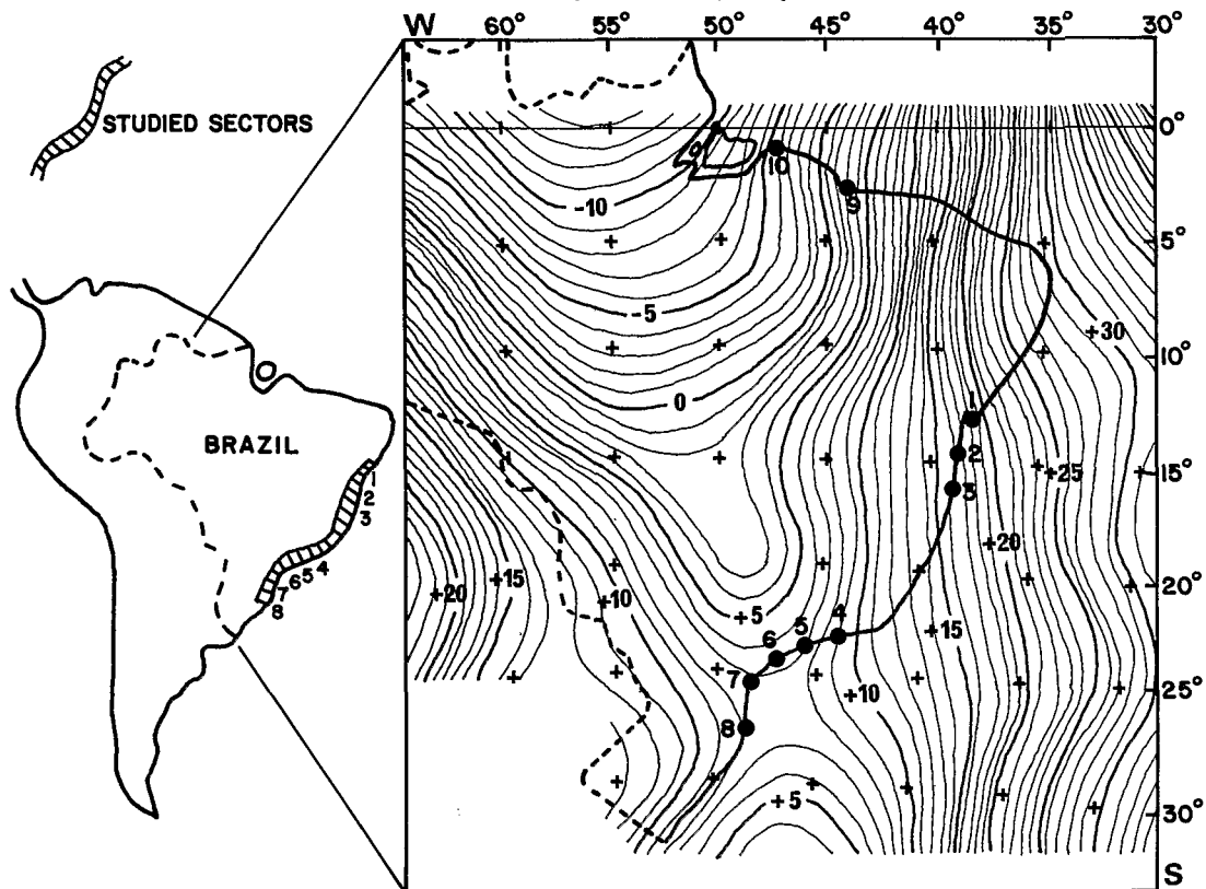
FIGURE 1 - Index map of the studies sectors of the Brazilian coast. Geoid chart of Brasil. (1) Salvador; (2) Ilhéus; (3) Caravelas; (4) Angra dos Reis; (5) Santos; (6) Cananéia; (7) Paranaguá; (8) Itajaí; (9) São Luís; (10) Belém.
