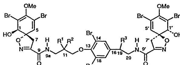
5 R^1 = R^3 = OH, R^2 = H 6 R^1 = R^2 = O, R^3 = OH 7 R^1 = R^2 = R^3 = H 8 R^1 = OH, R^2 = R^3 = H 9 R^1 = R^2 = O, R^3 = H
