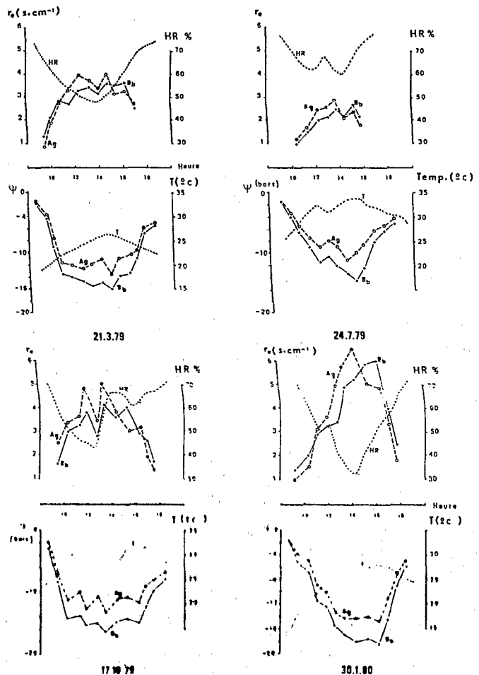
Fig. 4 - Valeurs simultanées de la résistance épidermique au flux de vapeur ( r_e ) et du potentiel de l'eau dans la vascularisation ( \psi ) chez Andropogon gayanus (Ag) et Brachiaria brizantha (Bb), au cours de quatre journées types de l'année à Sangalkam (région du Cap-Vert) T : température atmosphérique (°C) ; HR : humidité relative de l'air (%)
