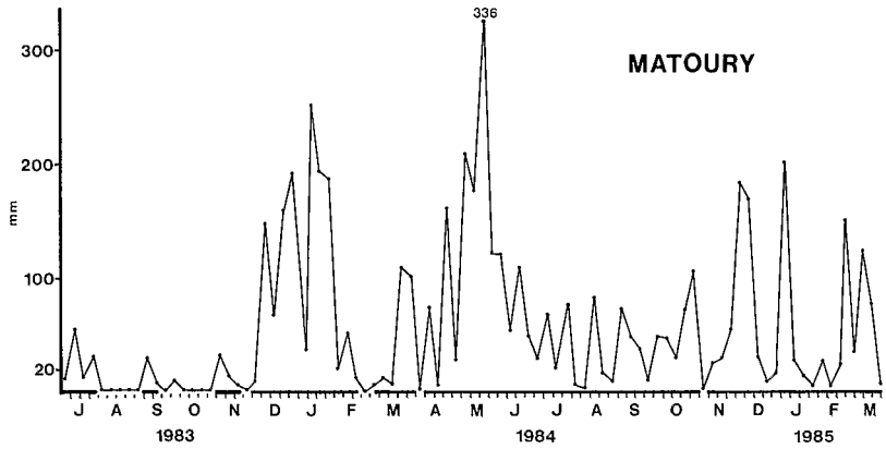
Fig. 1c. Rainfall in Matoury, F. G.
