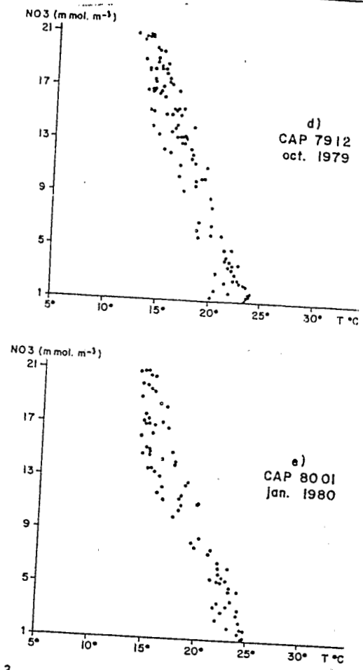
Figure 3 Les relations nitrate/température à 4°W entre 0 et 5°S pendant le programme Cipea. a : août 1978; b : avril 1979; c : juin 1979; d : octobre 1979; e : janvier 1980. Relationships nitrate/temperature along 4°W between 0 and 5°S during the Cipea programme. a : August 1978; b : April 1979; c : June 1979; d : October 1979; e : January 1980.
