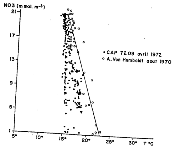
Figure 5 Relation nitrate/température dans la région mauritanienne (Cap Timiris) en août/septembre 1970 (saison chaude) et en avril 1972 (période d'upwelling). Les ronds noirs correspondent à l'upwelling (N/O Capricorne) et les cercles blancs à la saison chaude (N/O A. Von Humboldt). Relationship nitrate/temperature in the Mauritanian region (Cape Timiris) in August-September 1970 (warm season) and in April 1972 (upwelling). Black circles: upwelling season (R/V Capricorne); Open circles: typical tropical structure (R/V A. von Humboldt).
