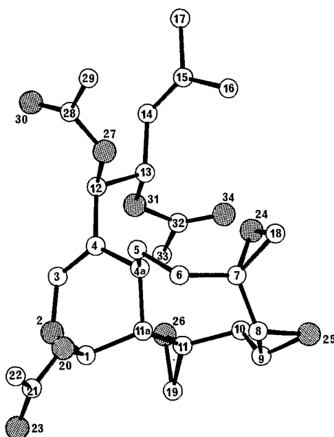
FIGURE 1. Vue en perspective de la havannahine [ 4 ]. (Les atomes d'oxygène sont en pointillé; les atomes d'hydrogène n'ont pas été dessinés pour une plus grande clarté.)
