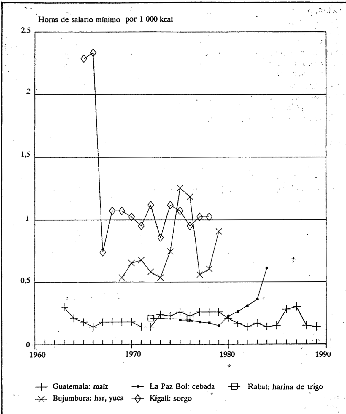
FIGURA 5. Precio de 1 000 kilocalorías, en salario mínimo por hora, del alimento energético más barato en varias ciudades del mundo.
