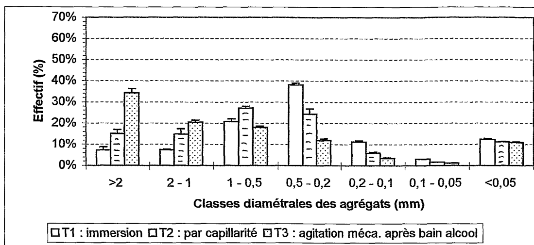
Figure 1 – Répartition des fractions d'agrégats après les 3 traitements T1, T2 et T3 du test de stabilité structurale (échantillon P4 (« banane établie »), mars 2000).
