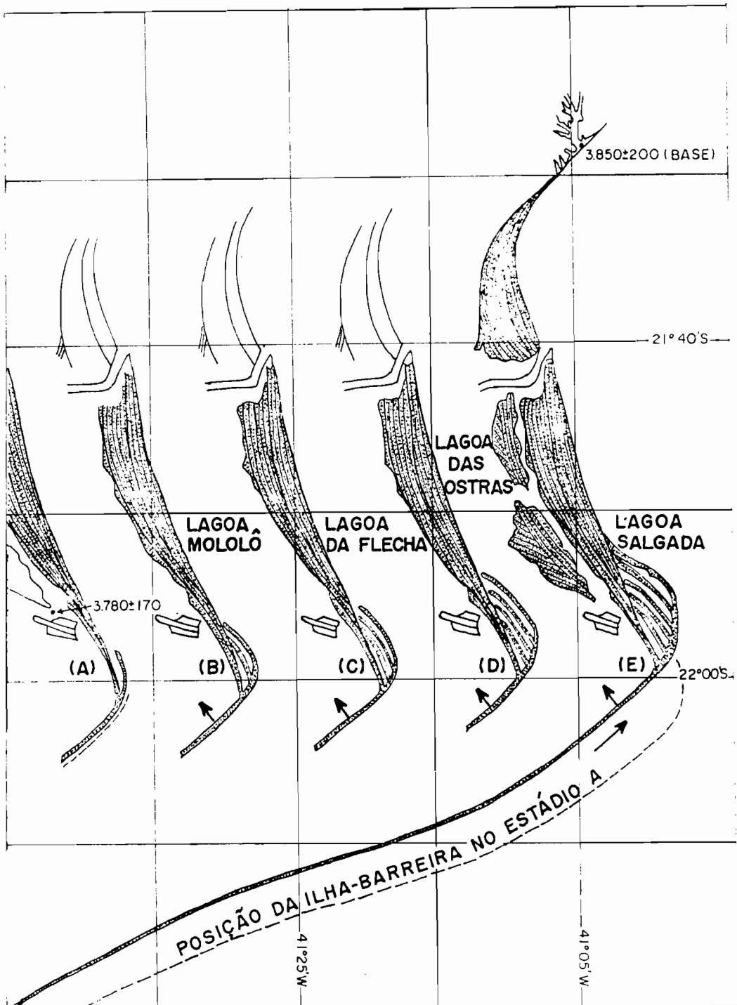
Figura 68 - Estádio C: Sequência de formação das lagoas costeiras Mololô, da Flecha, das Ostras e Salgada, ao norte do Cabo de São Tomé, entre 3.900 e 3.600 anos A.P.
