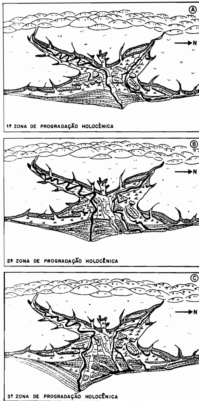
Figura 84 - Esquema evolutivos da planície costeira do Rio Jequitinhonha durante o Holoceno entre 5.100 - 0 anos A.P. (DOMINGUEZ, 1982).
