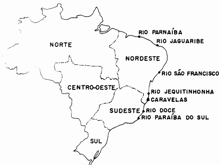
Figura 1 - Posições geográficas dos "deltas holocênicos" brasileiros (BACOCOLI, 1971) e a localização da planície costeira de Caravelas (BA).
