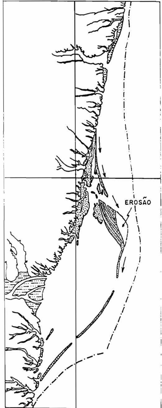
Figura 27 - Subestádio B-2: Primeira fase de erosão do intervalo de tempo correspondente a 5.100-4.200 anos A.P.
