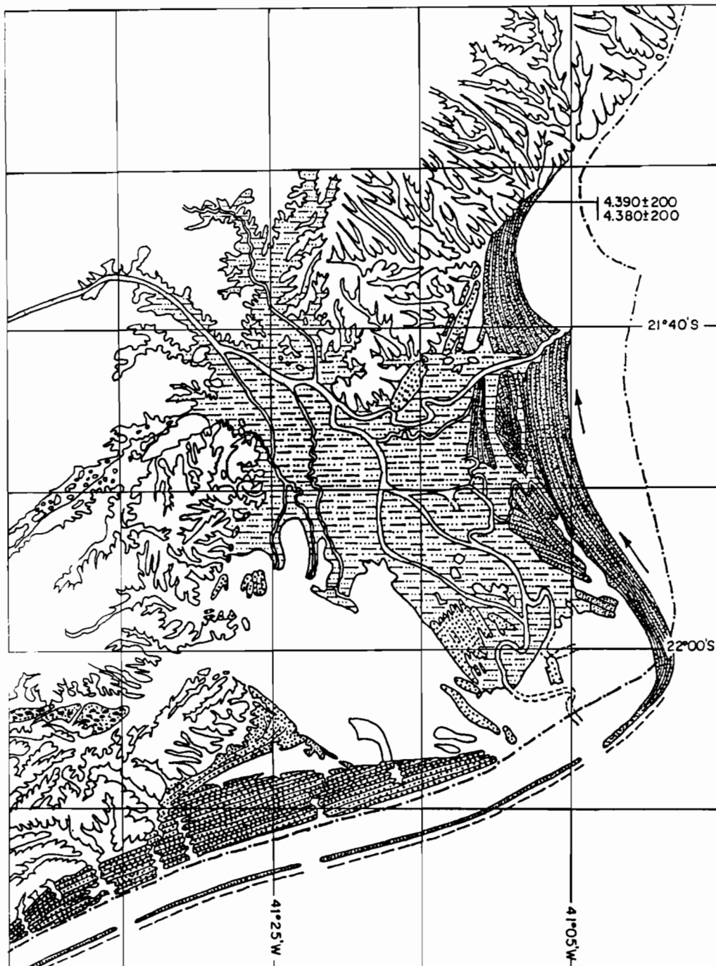
Figura 66 - Subestádio B-5: Segunda fase de construção a partir da desembocadura A no intervalo de tempo correspondente a 5.100 - 3.900 anos A.P.
