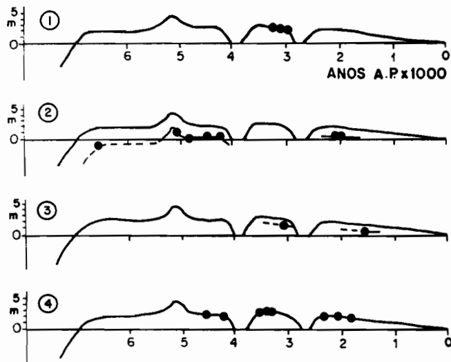
Figura 5 - Evidências de tectonismo holocênico, na região da Baía de Todos os Santos (BA) vendo-se, de cima para baixo, mapa geológico esquemático com blocos de falhas e o perfil transversal às falhas (FERNANDES FILHO et al., 1982) e, finalmente, os paleoníveis marinhos reconstruídos através de dados obtidos nos blocos 1 a 4 (MARTIN et al., 1984a).
