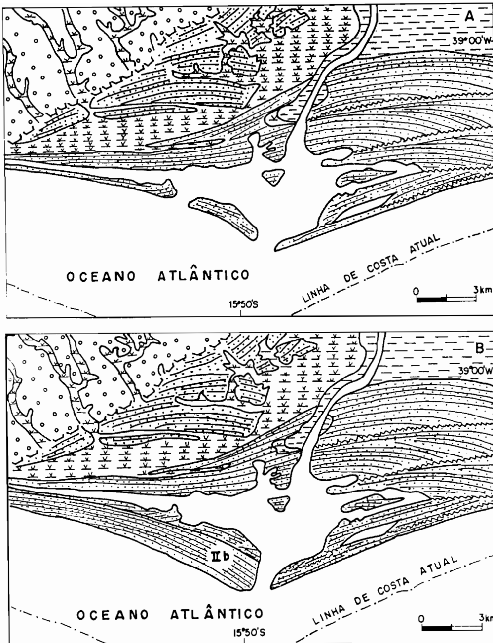
Figura 85 - (A) Paleogeografia durante o afogamento da segunda zona de progradação holocênica do Rio Jequitinhonha. (B) Após o afogamento a linha de costa ainda teve condições de progradar rumo ao mar, principalmente ao sul da desembocadura do Rio Jequitinhonha, quando então foi construído o subsistema de cristas praias IIb (DOMINGUEZ, 1982).
