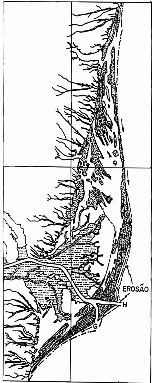
Figura 53 - Subestádio G-6: Terceira fase de erosão do intervalo de tempo correspondente a 2.500 - 0 anos A.P.
