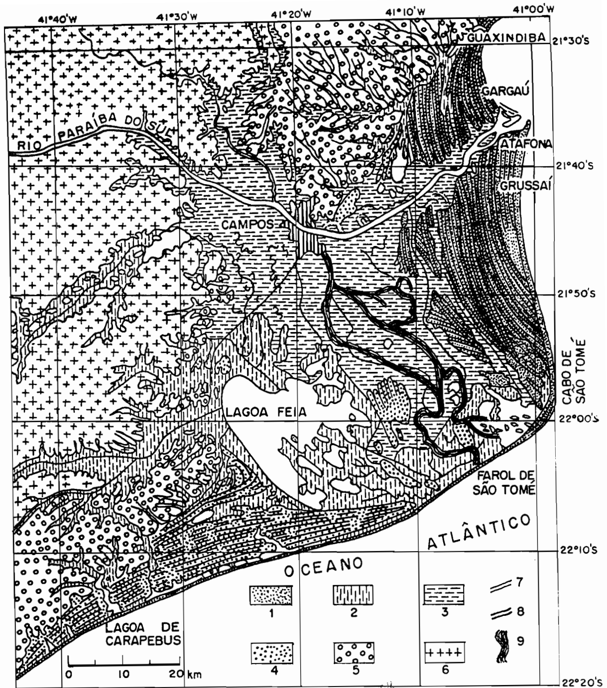
Figura 56 - Mapa geológico esquemático da planície costeira do Rio Paraíba do Sul (ES): (1) terraço marinho holocênico, (2) sedimentos lagunares, (3) sedimentos fluviais (delta intralagunar), (4) terraço pleistocênico, (5) sedimentos continentais terciários (Formação Barreiras), (6) embasamento cristalino pré-cambriano, (7) alinhamentos de cristas praias holocênicas; (8) alinhamentos de cristas praias pleistocênicas e (9) paleocanais fluviais.
