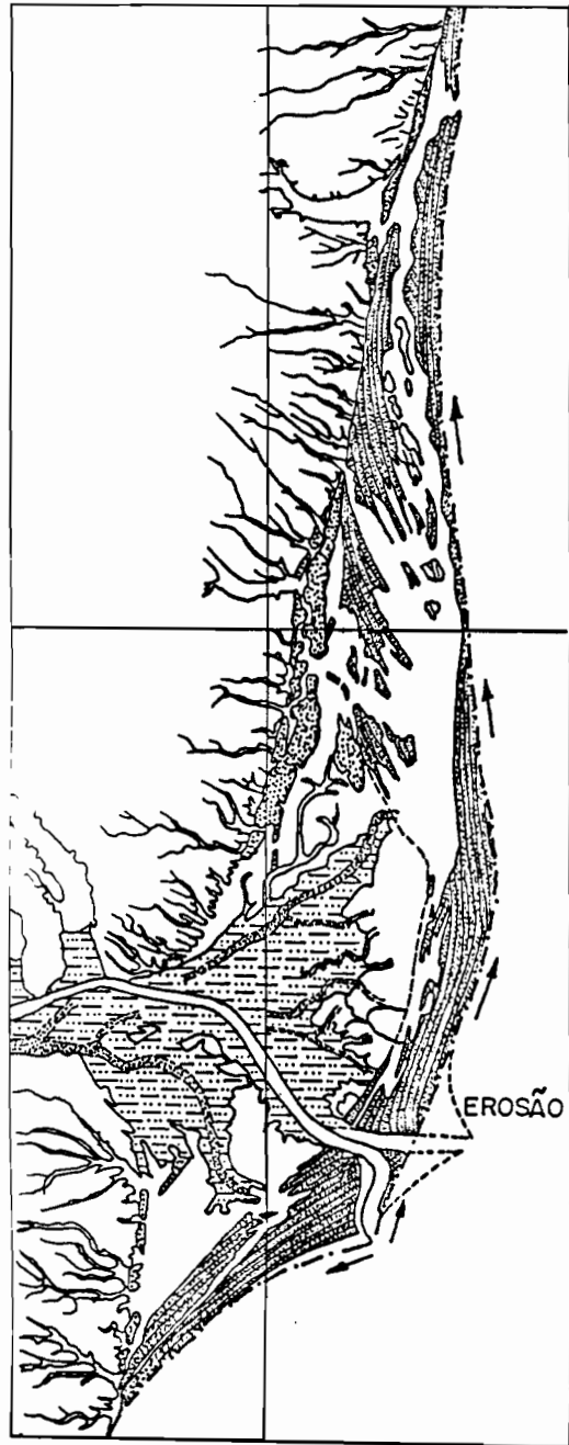
Figura 55 - Subestádio G-8 e G-9: Abandono da desembocadura norte (H) e erosão das zonas em desequilíbrio hidrodinâmico.
