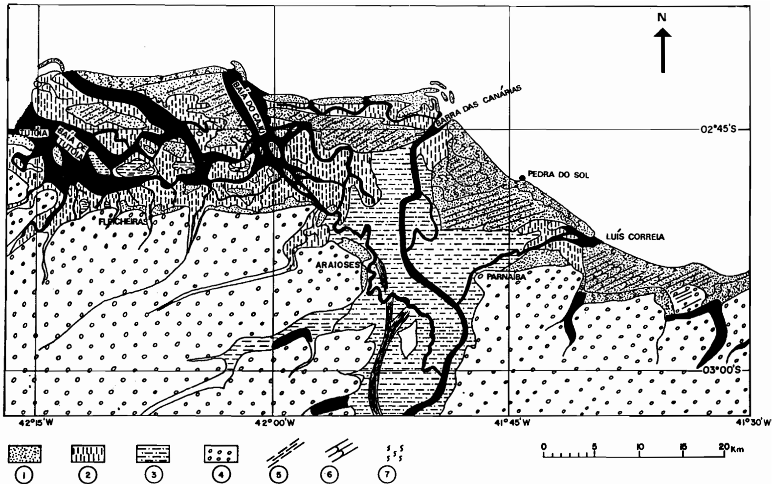
Figura 90 - Mapa geológico esquemático da planície costeira do Rio Parnaíba (PI/MA): (1) areias holocênicas, (2) depósitos de manguezal, (3) sedimentos fluviais, (4) Formação Barreiras com dunas pleistocênicas, (5) cicatrizes de deslocamento de dunas barcanas, (6) dunas barcanas e (7) areias retrabalhadas pelo vento.
