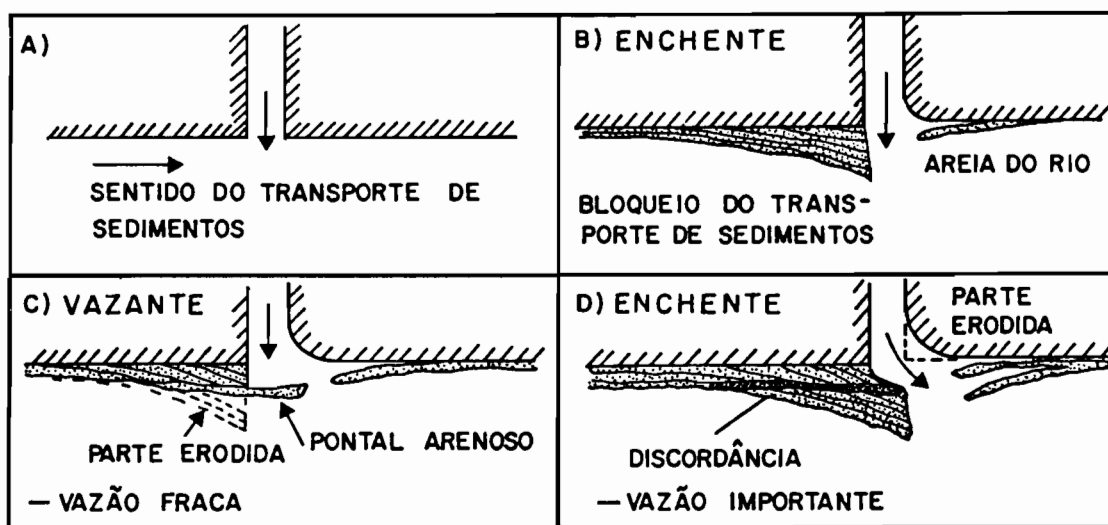
Figura 10 - Mecanismo de bloqueio do transporte litorâneo de areias, paralelamente à costa, por efeito de fluxo ligado a uma desembocadura fluvial em regiões costeiras, exibindo alternância de fases de débitos fluviais.
