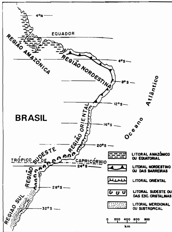
Figura 12 - Classificação do litoral brasileiro por SILVEIRA (1964), baseada em elementos oceanográficos, climáticos e continentais.
