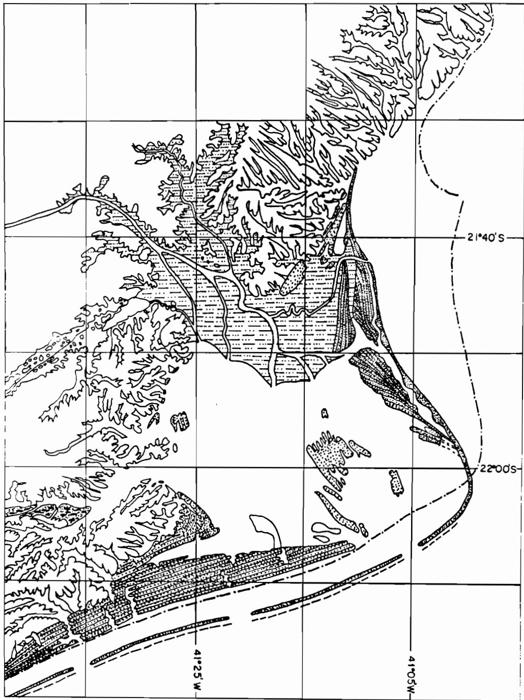
Figura 63 - Subestádio B-2: Saída direta para o mar de um distributário do delta intralagunar no intervalo de tempo correspondente a 5.100 - 3.900 anos A.P.
