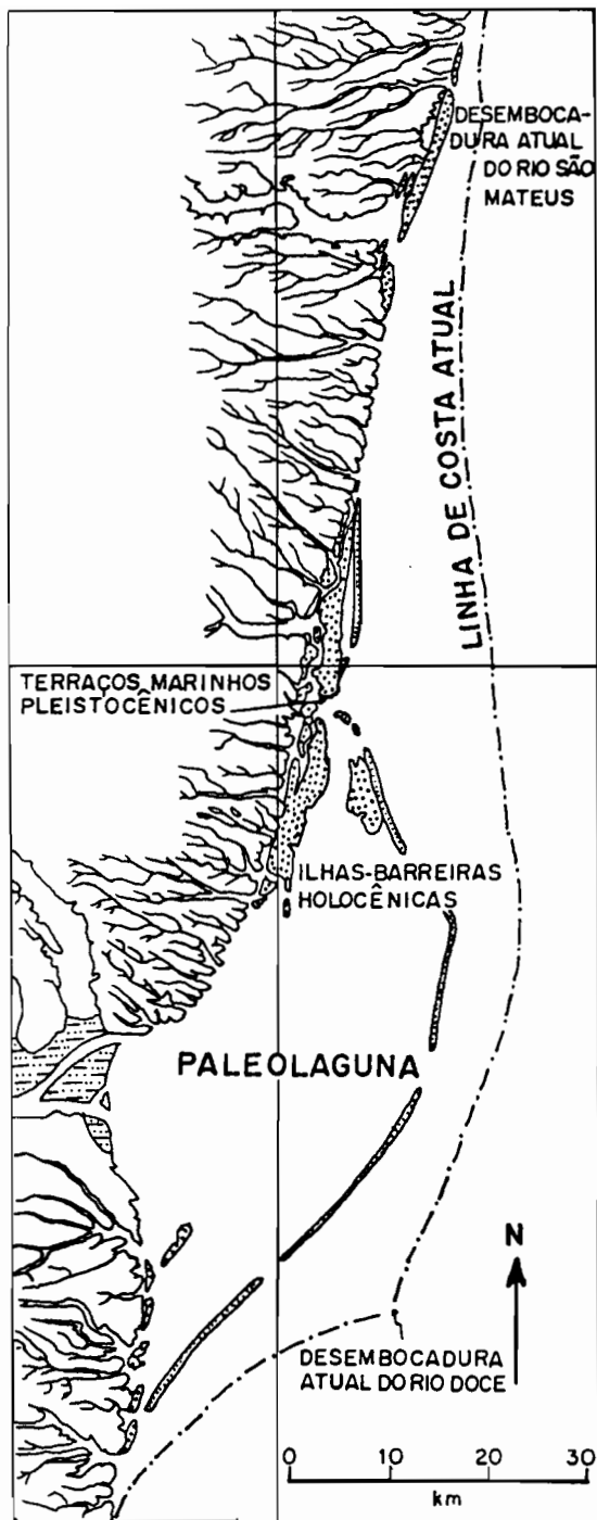
Figura 25 - Estádio A: Fase anterior a 5.100 anos A.P. - Situação do sistema ilhas-barreiras/laguna ao redor de 5.100 anos A.P., correspondente ao nível máximo holocênico. Podem ser vistos testemunhos de terraços marinhos pleistocênicos, situação da linha de costa atual e as posições atuais das desembocaduras dos rios Doce e São Mateus.
