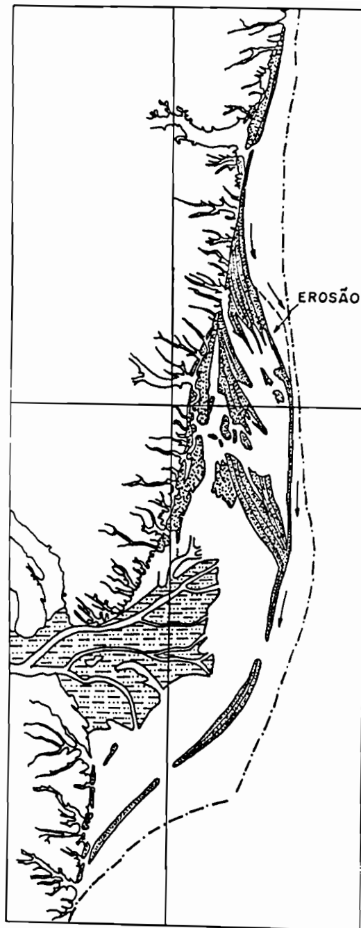
Figura 35 - Subestádio B-10: Quinta fase de erosão do intervalo de tempo correspondente a 5.100-4.200 anos A.P.
