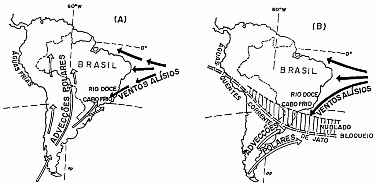
Figura 19 - Esquemas de circulação atmosférica sobre a América do Sul sob: (A) condições normais e (B) durante fenômenos do tipo "EL Niño", como em 1983, regida por ventos alísios e adveções polares.
