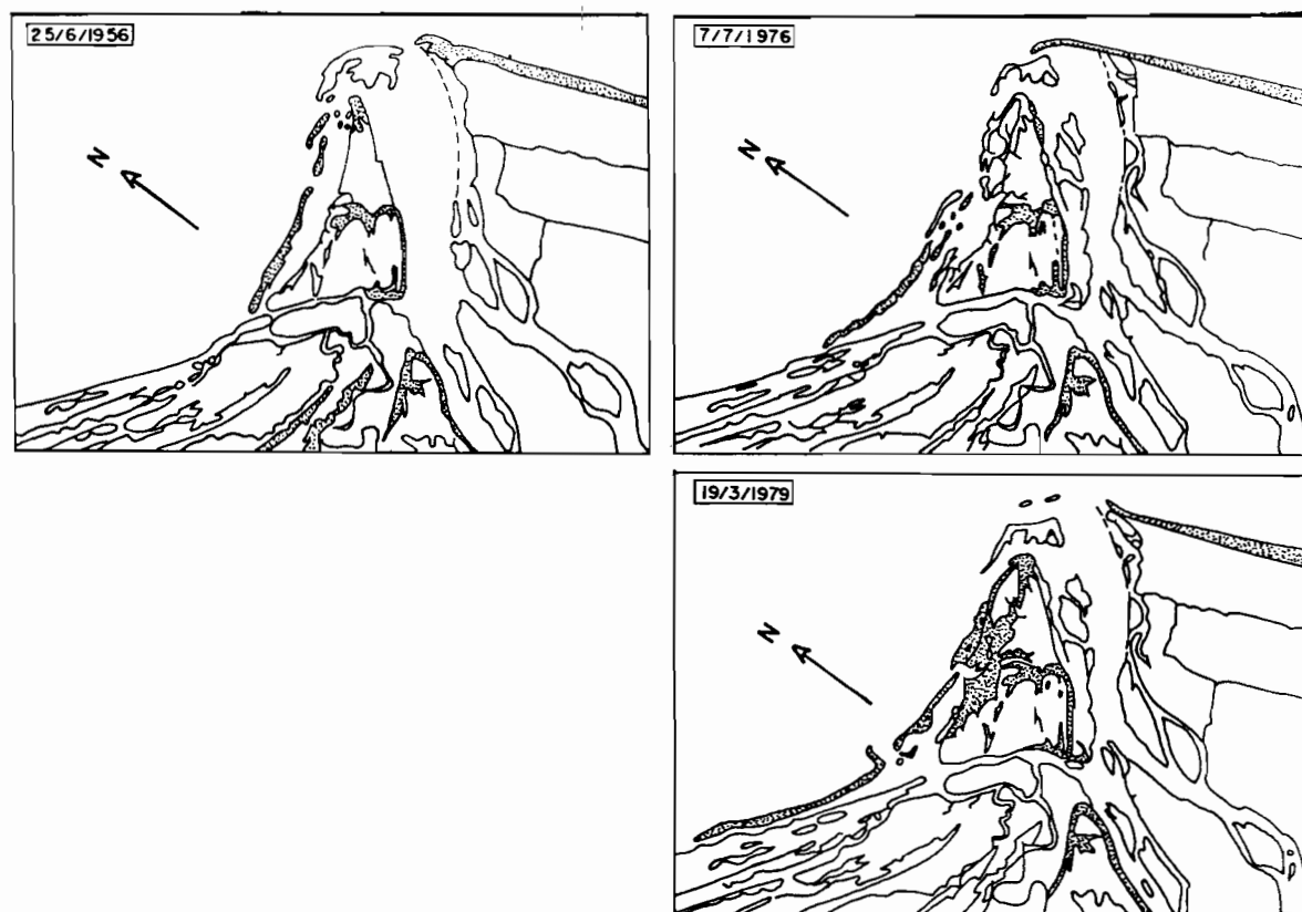
Figura 78 - Modificações nas características morfológicas da foz atual do Rio Paraíba do Sul entre os anos de 1956 e 1979 (DIAS, 1981).
