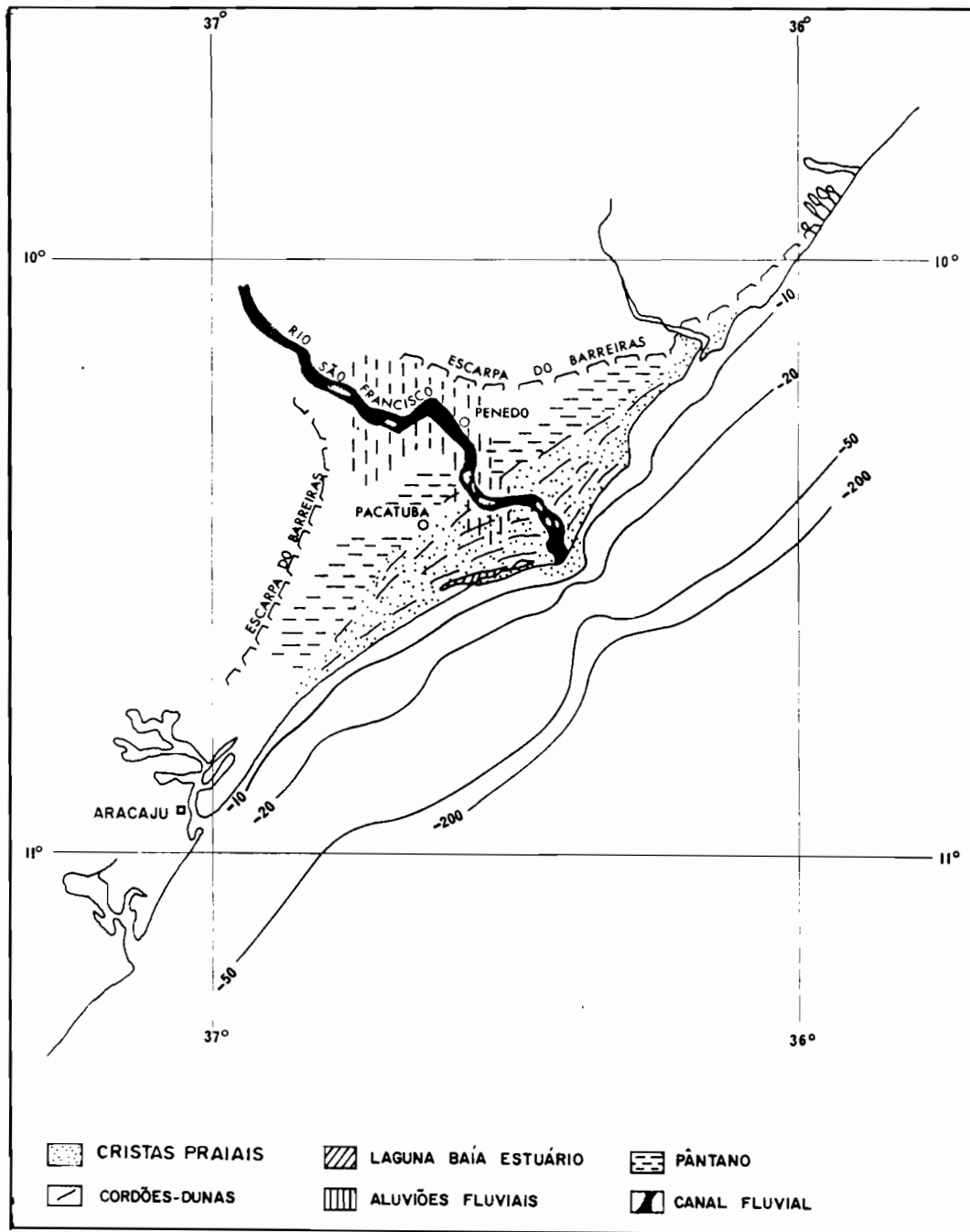
Figura 88 - Mapa geológico do "delta" do Rio São Francisco segundo BACOCOLI (1971).
