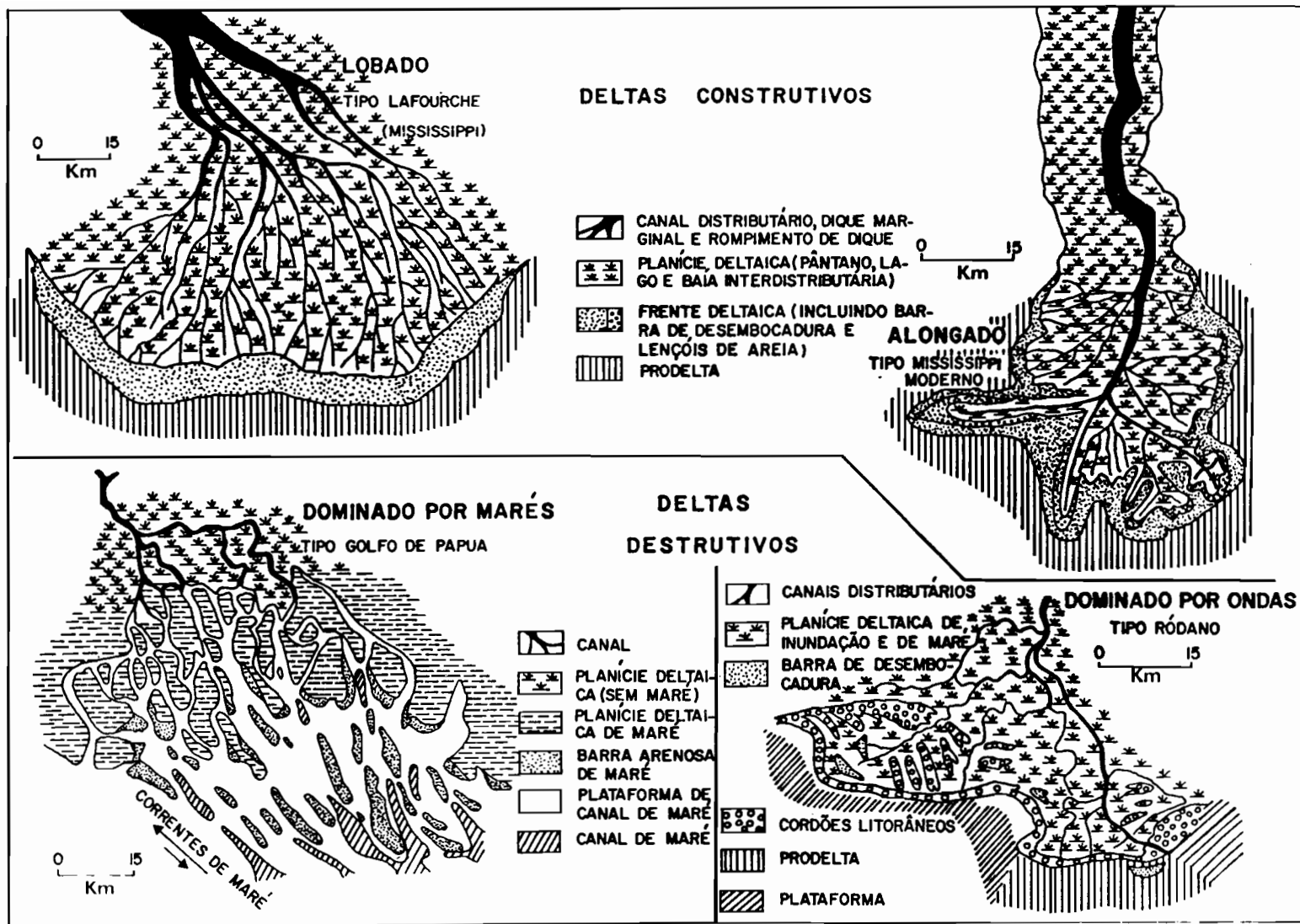
Figura 16 - Classificação genética de deltas marinhos ou oceânicos segundo a predominância de processos fluviais (deltas construtivos) ou marinhos (deltas destrutivos), cada um comportando uma subdivisão em dois subtipos (SCOTT & FISHER, 1969).
