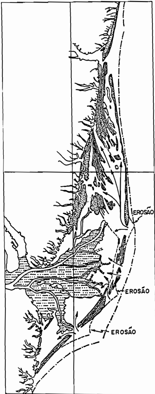
Figura 44 - Estádio D: Entre 3.900 e 3.600 anos A.P. - Submersão acompanhada de erosão ao redor das desembocaduras dos distributários.
