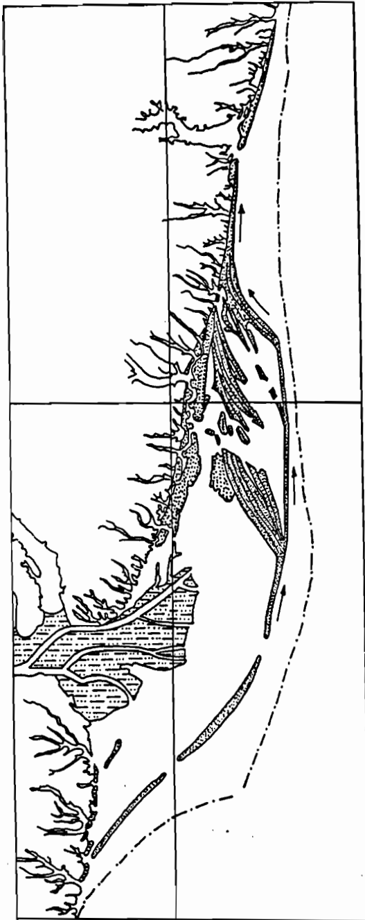
Figura 32 - Subestádio B-7: Quarta fase de construção do intervalo de tempo correspondente a 5.100-4.200 anos A.P.
