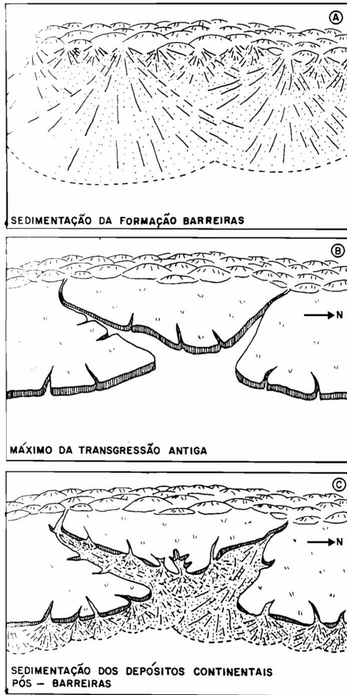
Figura 82 - Esquemas evolutivos da planície costeira do Rio Jequitinhonha do fim do Terciário (sedimentação de leques coalescentes da Formação Barreiras) até o Pleistoceno (antes de 123.000 anos A.P.) segundo DOMINGUEZ (1982).
