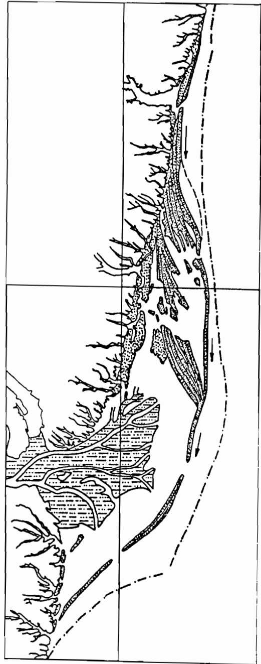
Figura 37 - Subestádio B-12: Sexta fase de erosão do intervalo de tempo correspondente a 5.100-4.200 anos A.P.
