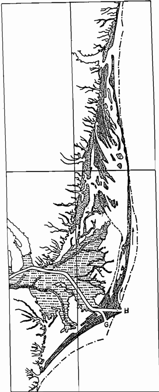
Figura 46 - Estádio E: Entre 3.600 e 2.700 ano A.P. - Progradação acompanhando a formação de duas novas desembocaduras (G e H).
