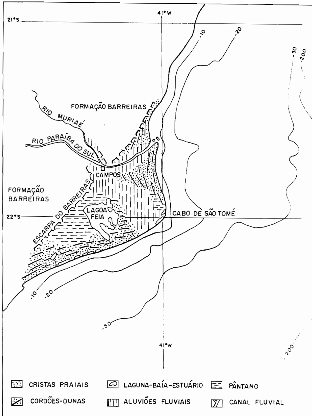
Figura 57 - Mapa geológico esquemático do "delta" do Rio Paraíba do Sul segundo BACOCOLI (1971).
