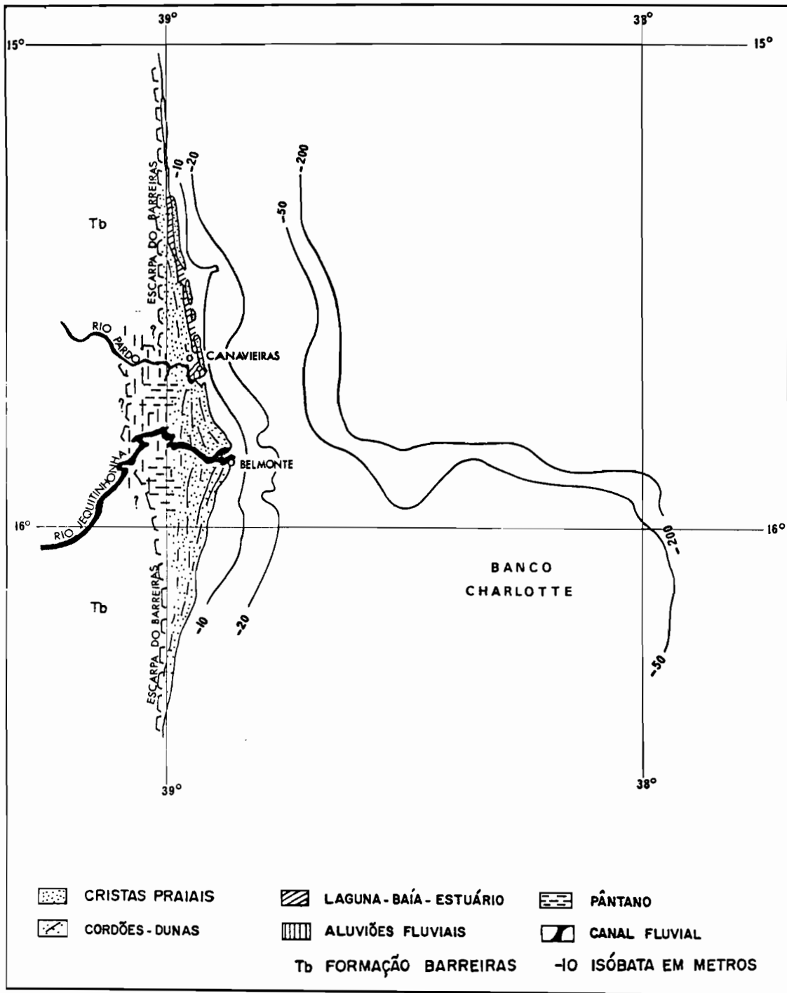
Figura 81 - Mapa geológico esquemático do "delta" do Rio Jequitinhonha segundo BACOCOLI (1971).
