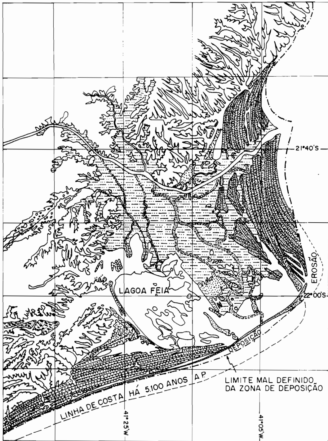
Figura 76 - Subestádio E-5: Fase de erosão acelerada no intervalo de tempo correspondente a 2.500 - 0 anos A.P.
