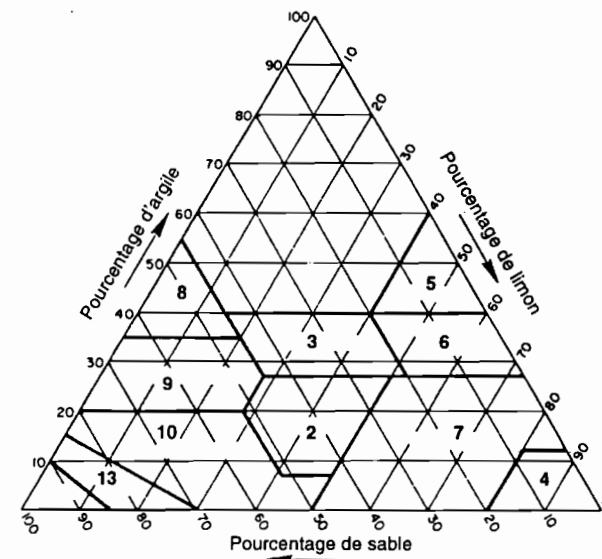
Fig. 2 Classes texturales
