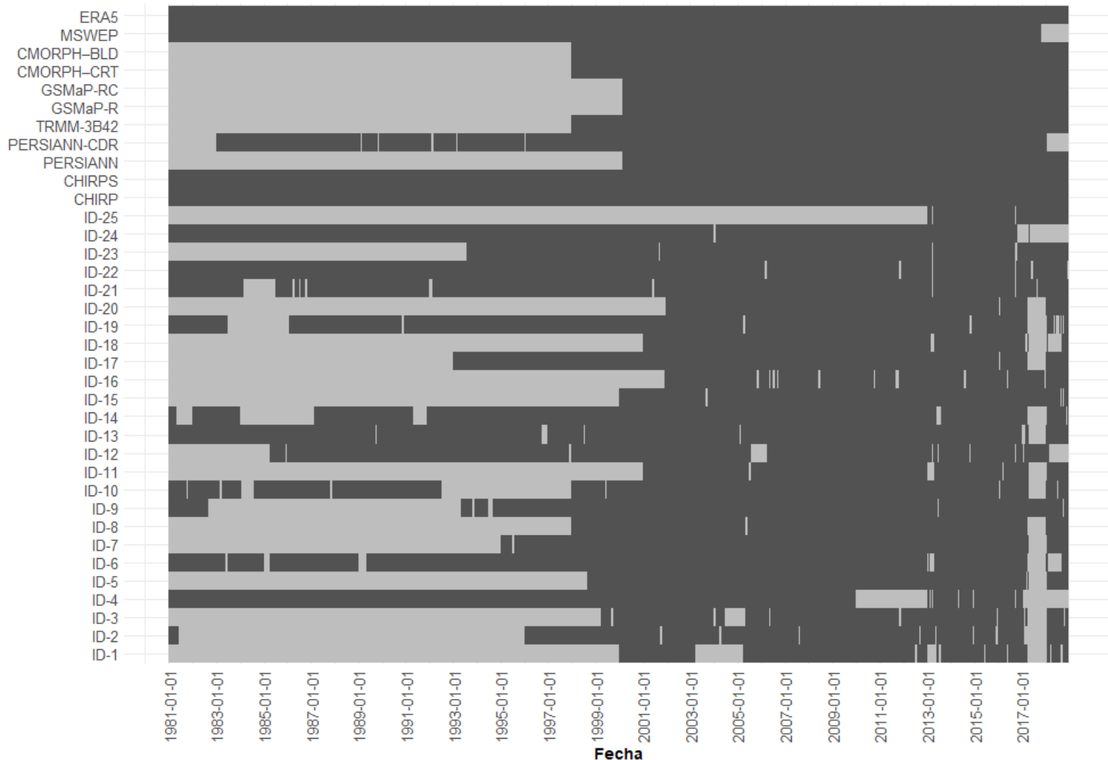
Figura 2. Disponibilidad de datos diarios en las 24 estaciones pluviométricas y en los PPEDsr (ERA5, MSWEP, CMORPH-BLD, CMORPH-CRT, GSMaP-RC, GSMaP-R, TRMM-3B42, PERSIANN-CDR, PERSIANN, CHIRPS, CHIRP). Gris oscuro: presencia de dato; gris claro: ausencia de dato.
