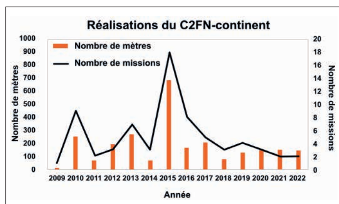
Figure A 2.2. Évolution des nombres de mètres de carottes et de missions réalisées par l'atelier de forage de la DT-INSU depuis la création du C2FN en 2009. Cette structure est devenue le cœur de l'instrument national CCF en 2022. Ces missions représentent une fraction infime de l'activité de carottage en domaine continental, mais ce sont les missions les plus ambitieuses, utilisant les matériels les plus lourds opérés par une équipe technique dédiée.
