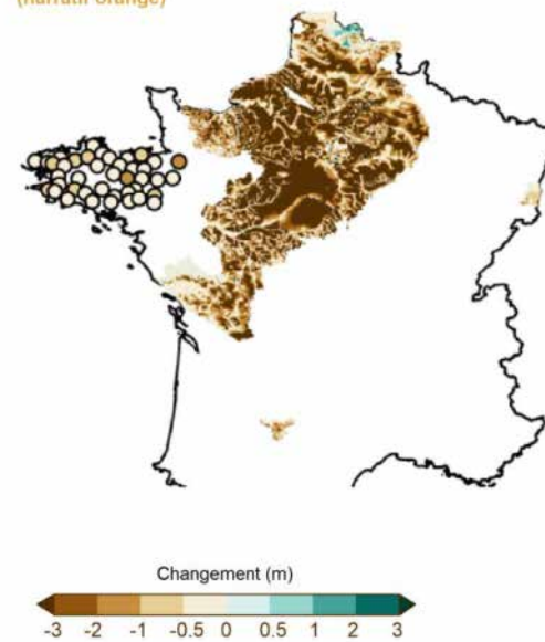
Fort réchauffement et fort assèchement en été (et en annuel) (narratif orange)
