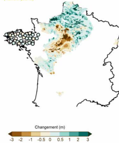
Changements futurs relativement peu marqués (narratif jaune)
