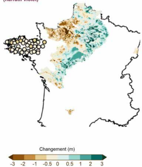
Fort réchauffement et forts contrastes saisonniers en précipitations (narratif violet)
