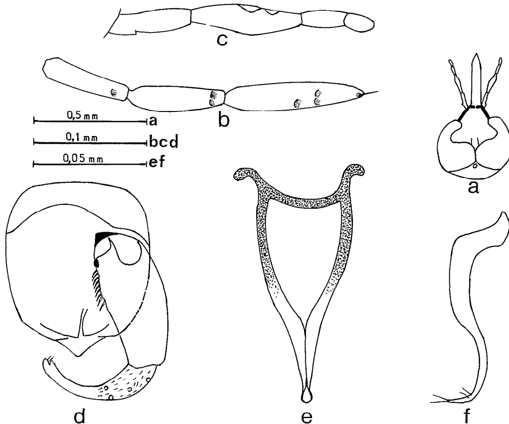
FIG. 1. — Culicoides nutshuruensis Goetghebuer. a : schéma de la tête femelle ; b : trois derniers articles de l'antenne femelle ; c : palpe femelle ; d : neuvième segment, coxite et style du mâle ; e : édage ; f : paramère
