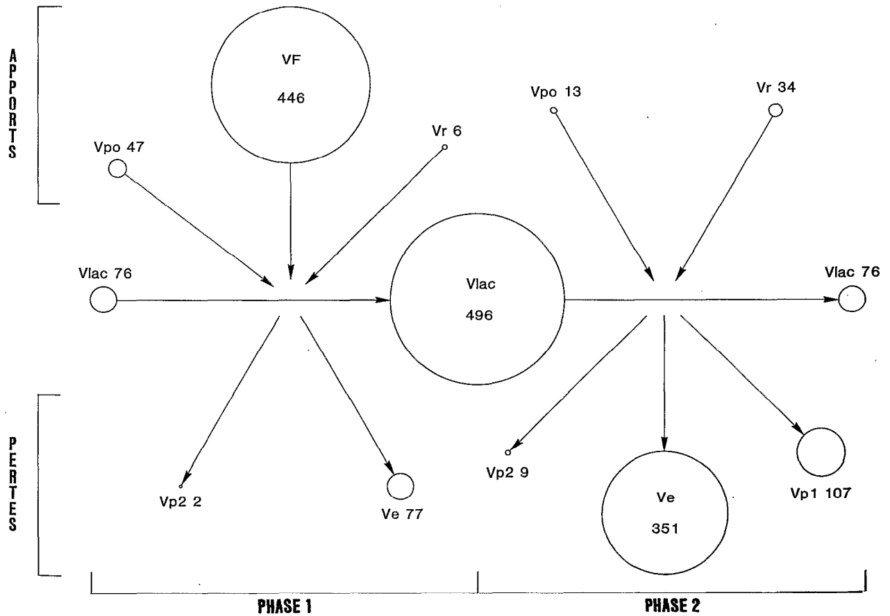
Fig. 3. — Bilan hydrologique moyen annuel par phase ( 10^6\text{m}^3 ) VF : Apports fluviaux — V_{p1} : Pompages CSS — Vr : Rejets CSS — V_{p2} : Pompages eau potable — Vpo : Pluviométrie — Ve : Évaporation — Vlac : Volume lacustre (en début et fin de phase de remplissage). Phase 1 : Remplissage — Phase 2 : Isolement.
