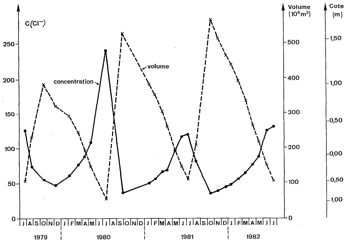
Fig. 5. — Évolution comparée des teneurs en Cl - (mg/l) du volume et de la cote du lac de juillet 1979 à juillet 1982.
