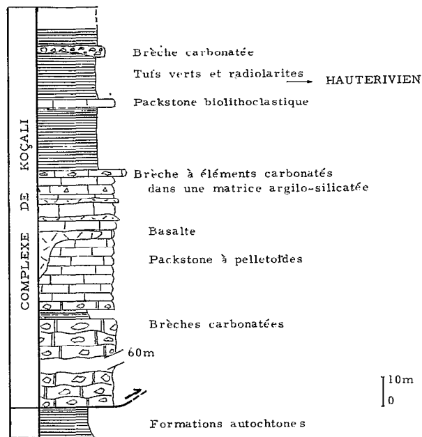
FIG. 5. — Coupe du complexe de Koçali (Ikiyaka-mounts Cilo)
