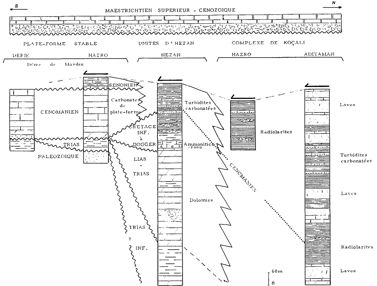
Fig. 9. --- Relations stratigraphiques et structurales entre la plate-forme arabe stable, sa bordure et le domaine océanique. Transversale nord-sud en Turquie du Sud-Est. Le complexe de Koçali s'étendant du Trias supérieur (?) au Sénonien
