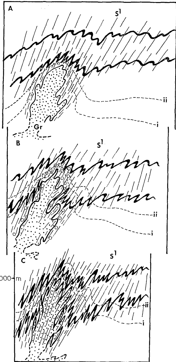
FIG. 9. — Mécanisme hypothétique de mise en place du granite syncinématique précoce à deux micas du Zongo-Yani. Stade A : début de l'intrusion granitique et du plissement sym-métamorphique ; Stade B : accentuation du processus de montée des isogrades (i et ii) en dôme autour du granite à deux micas et front de muscovitisation et de tourmalinisation périgranitique (o) ; Stade C : fin de la tectogenèse et orthogncissification mésozonale du granite à deux micas. On notera que le style de la déformation anisopaque est accentué à proximité immédiate du granite et que les isogrades forment une « hernie » autour du granite.
