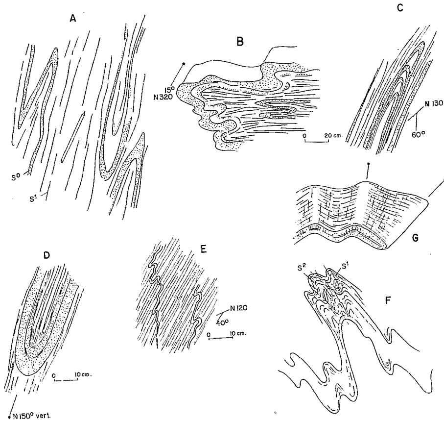
FIG. 3. — Structures mésoscopiques des phases I (A à G) et 2 (F et G) dans les métasédiments ordoviciens et siluriens du Zongo-Yani (So : stratification ; S 1 : schistosité de la phase 1 ; S 2 : schistosité de la phase 2).
