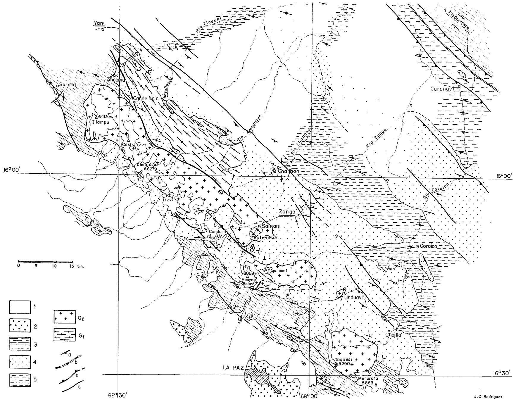
FIG. 2. — Carte géologique du Massif de Zongo-Yani (Cordillera Real, Bolivie) : 1. terrains récents ; 2. terrains andins ; 3. Siluro-Dévonien ; 4. Ordovicien supérieur ; 5. Ordovicien moyen ; G 1 , granites à deux micas hercyniens ; G 2 , granites andins ; a : schistosité ; b : front supérieur de schistosité ; c : failles inverses ; d : failles normales.
