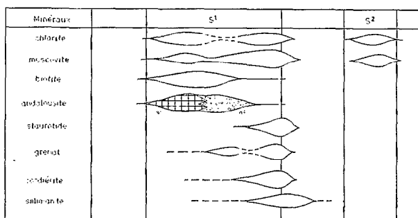
FIG. 5. — Ordre de cristallisation des minéraux du métamorphisme dans les métapelites du Zongo-Yani ( S^1 : schistosité de flux de la phase 1 (hercynien) ; S^2 : schistosité de fractures de la phase 2 (andin ou hercynien tardif?) - ( a^1 : andalousite « normale » ; a^2 : andalousite fortement poecilithique).
