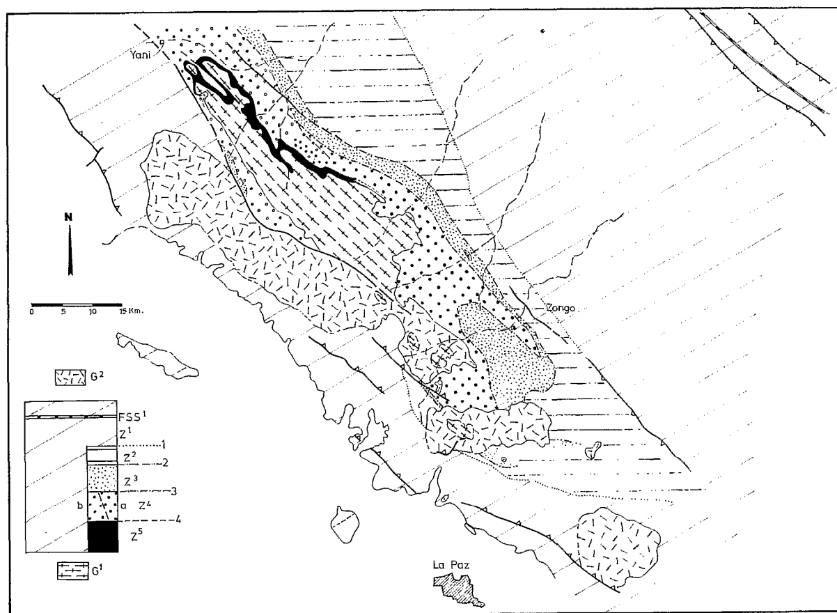
FIG. 6. — Carte zonéographique du Massif du Zongo-Yani ( Z^1 : métasédiments ordoviciens à siluriens épimétamorphiques ; Z^2 : zone de la biotite ; Z^3 : zone de l'andalousite ; Z^{4a} : zone de la sillimanite - 1 : isograde biotite (+) ; 2 : andalousite (+) ; 3 : staurotide ou cordiérite (+) ; 4 : sillimanite (+). G^1 : granite orthogneissifié à deux micas (hercynien) ; G^2 : granite calco-alcalin (andin) ; FSS^1 : front supérieur de la schistosité de flux hercynienne.
