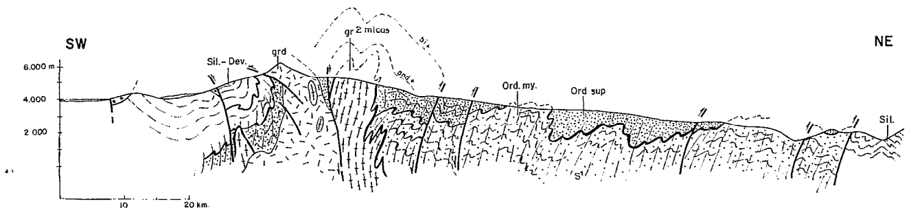
FIG. 7. — Coupe synthétique NE-SW du Massif du Zongo-Yani.
