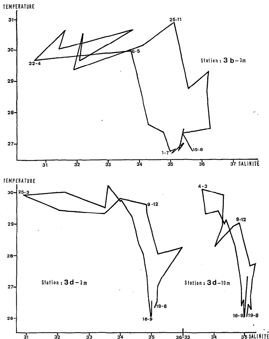
Fig. 4. — Diagrammes TS aux stations 3b et 3d.
