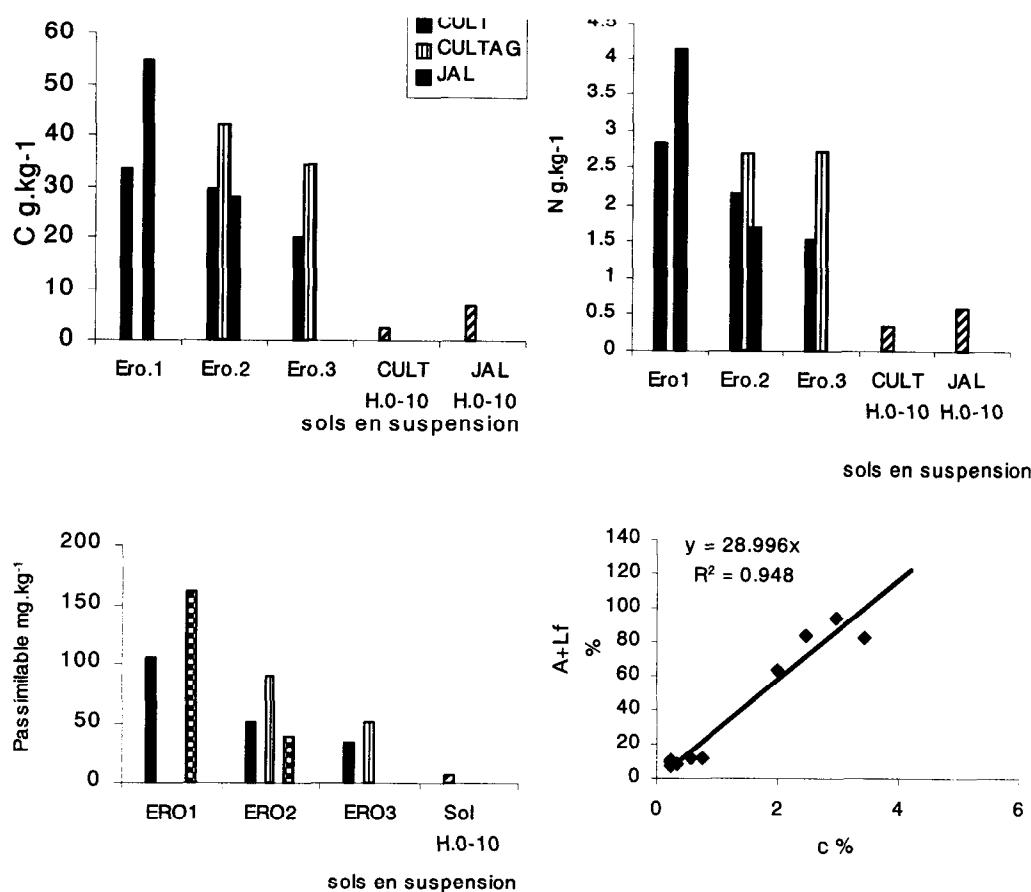
Figure 2 : Teneur en Pass, C et N des sols en suspension : teneurs en carbone (a), azote (b) et phosphore assimilable (c) regroupées en classe d'évènements érosifs Ero1 (érosion < 1\text{t.ha}^{-1} ), Ero2 ( 1\text{t.ha}^{-1} < \text{érosion} < 10\text{t.ha}^{-1} ), Ero3 (érosion > 10\text{t.ha}^{-1} ) et relation entre les éléments fins et le carbone total (d) dans la charge solide en tenant compte de l'horizon de surface 0-10 cm
