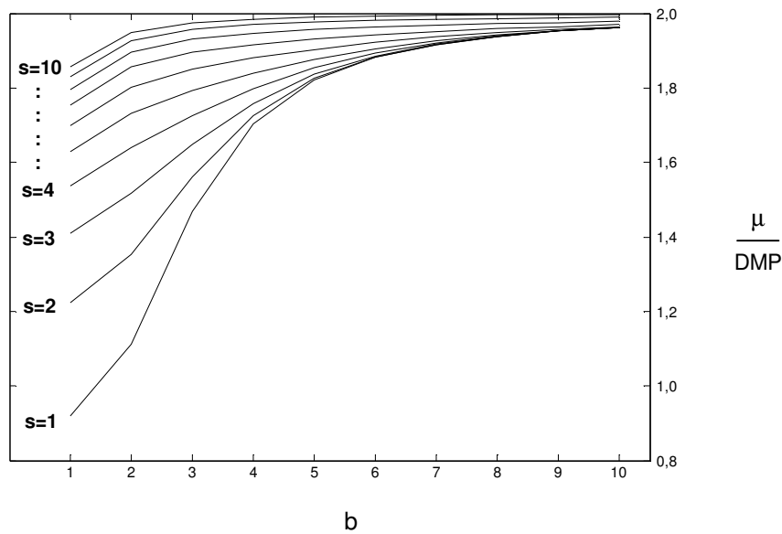
Figure II.20. Rapport \mu/DMP du modèle « Hazard-rate » pour des valeurs croissantes de s et b .
