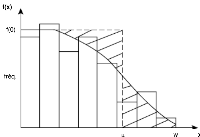
Figure II.4. Illustration graphique de la relation entre la largeur effective \mu et f(x) (d'après Thomas et al. 2002). La surface totale des barres de l'histogramme des fréquences d'observation est égale à 1. L'aire sous la courbe de f(x) s'ajustant à cette distribution est donc égale à 1. Par définition, les deux zones hachurées de part et d'autre de \mu ont une surface égale. L'aire du rectangle \mu \times f(0) est donc égale à 1, soit \mu = 1 / f(0) .
