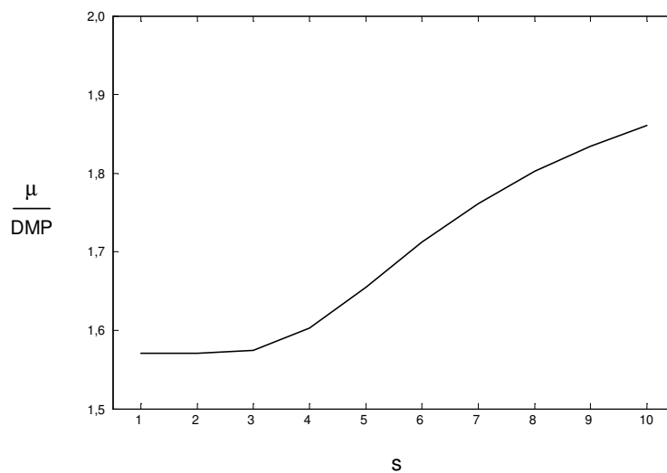
Figure II.18. Rapport \mu/DMP du modèle « Half-normal » pour des valeurs croissantes du paramètre s .
