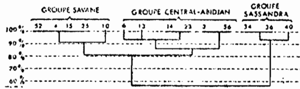
Figure 44 Dendrogramme après multiplication par graines
