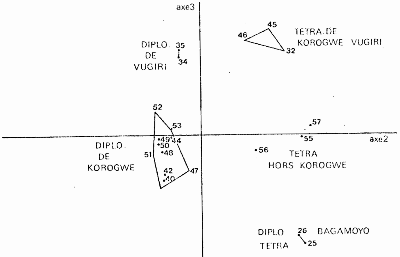
REPRESENTATION DES POPULATIONS DIPLOIDES ET TETRAPLOIDES VOISINES COMPOSANTES PRINCIPALES 2 ET 3
