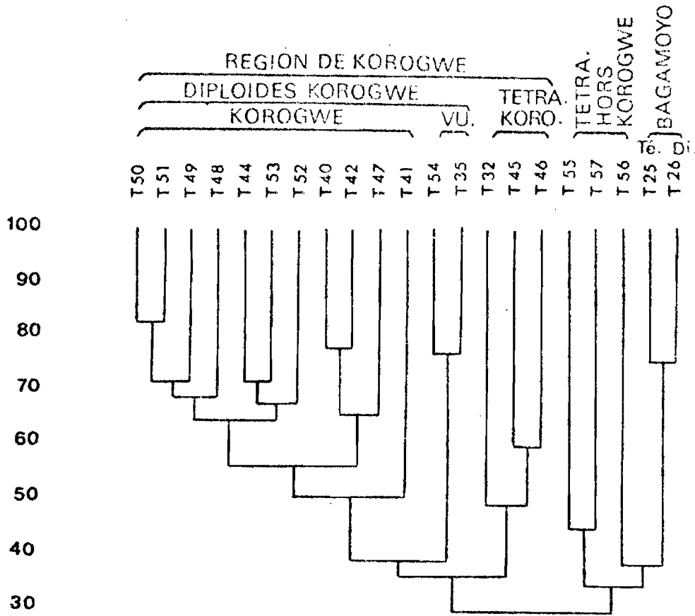
DENDROGRAMME DES POPULATIONS DIPLOIDES ET TETRAPLOIDES VOISINES
