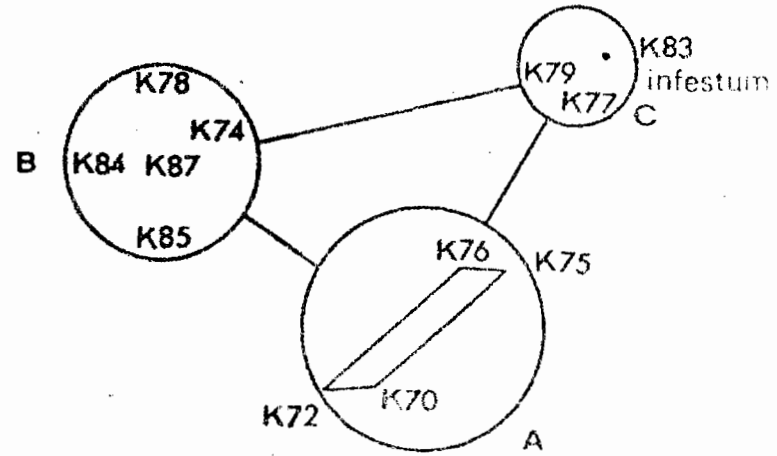
caractères indice ROGERS TANIMOTO (méthode nodale)
