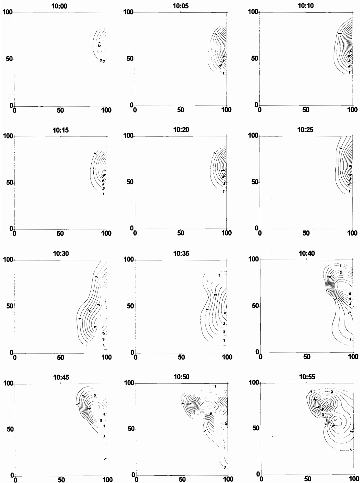
Figure 33: Isohyètes au pas de temps de 5 minutes du système précipitant du 9 juin.
