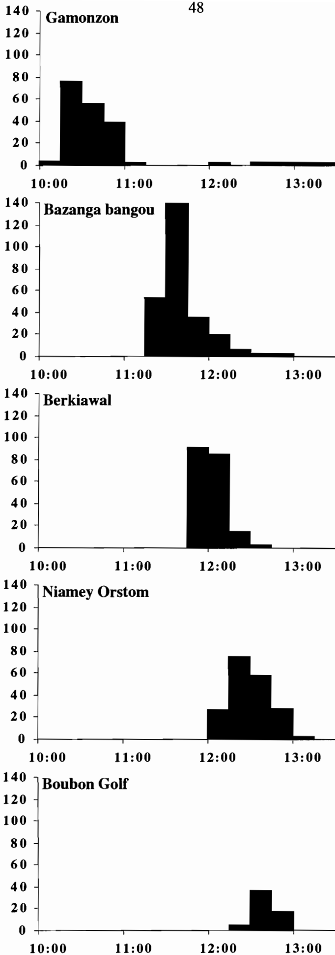
Figure 34: Hyétogramme de l'épisode du 9 juin 1996 pour 5 stations définissant un transect est-ouest.
