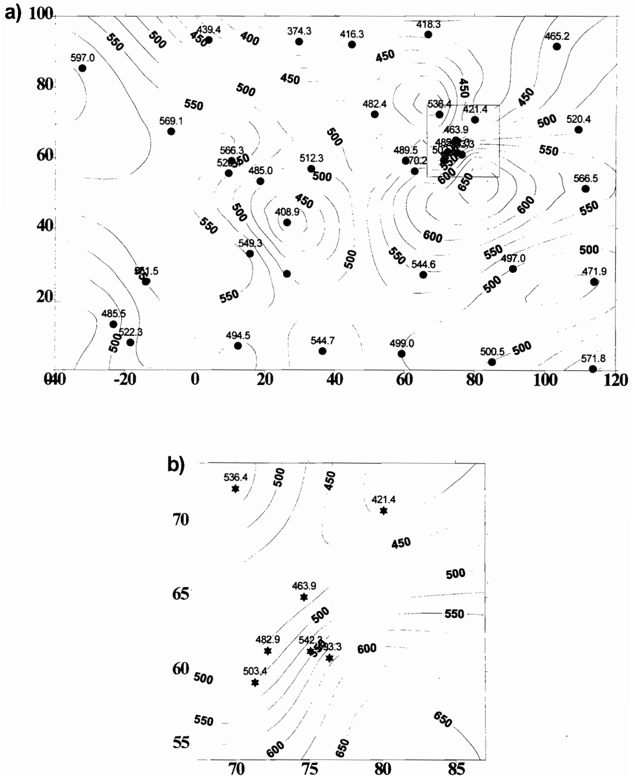
Figure 1: Isohyètes (mm) de la saison des pluies 1996 (15 avril 15 octobre) sur le degré carré de Niamey. 36 stations (cumuls seu). Coordonnées en km ; origine 2°E, 13°N. a) zone d'étude complète ; b) zoom sur le site central.
