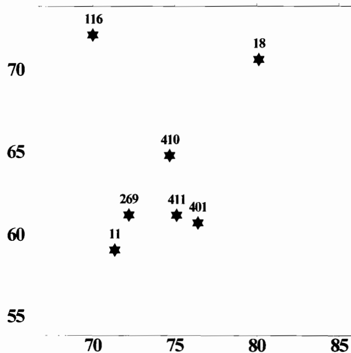
Figure 8: Dispositif de mesures durant la saison 1996. a) zone complète Coordonnées en km - Origine: 2°E, 13°N. b) site central
