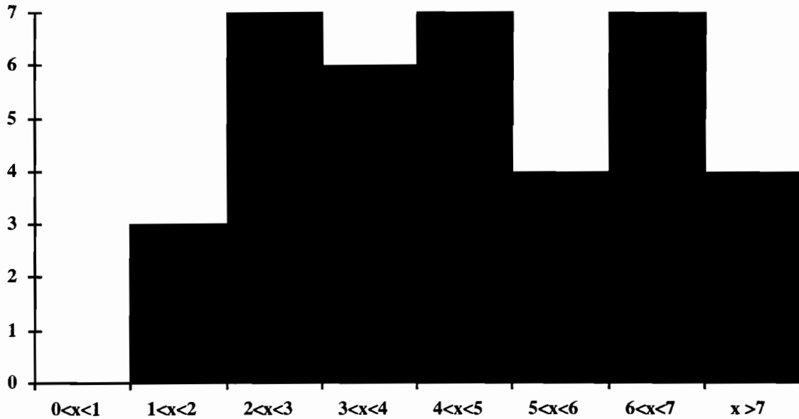
Figure 20: Histogramme de la durée en heure des épisodes spatiaux majeurs de la saison 1996.
