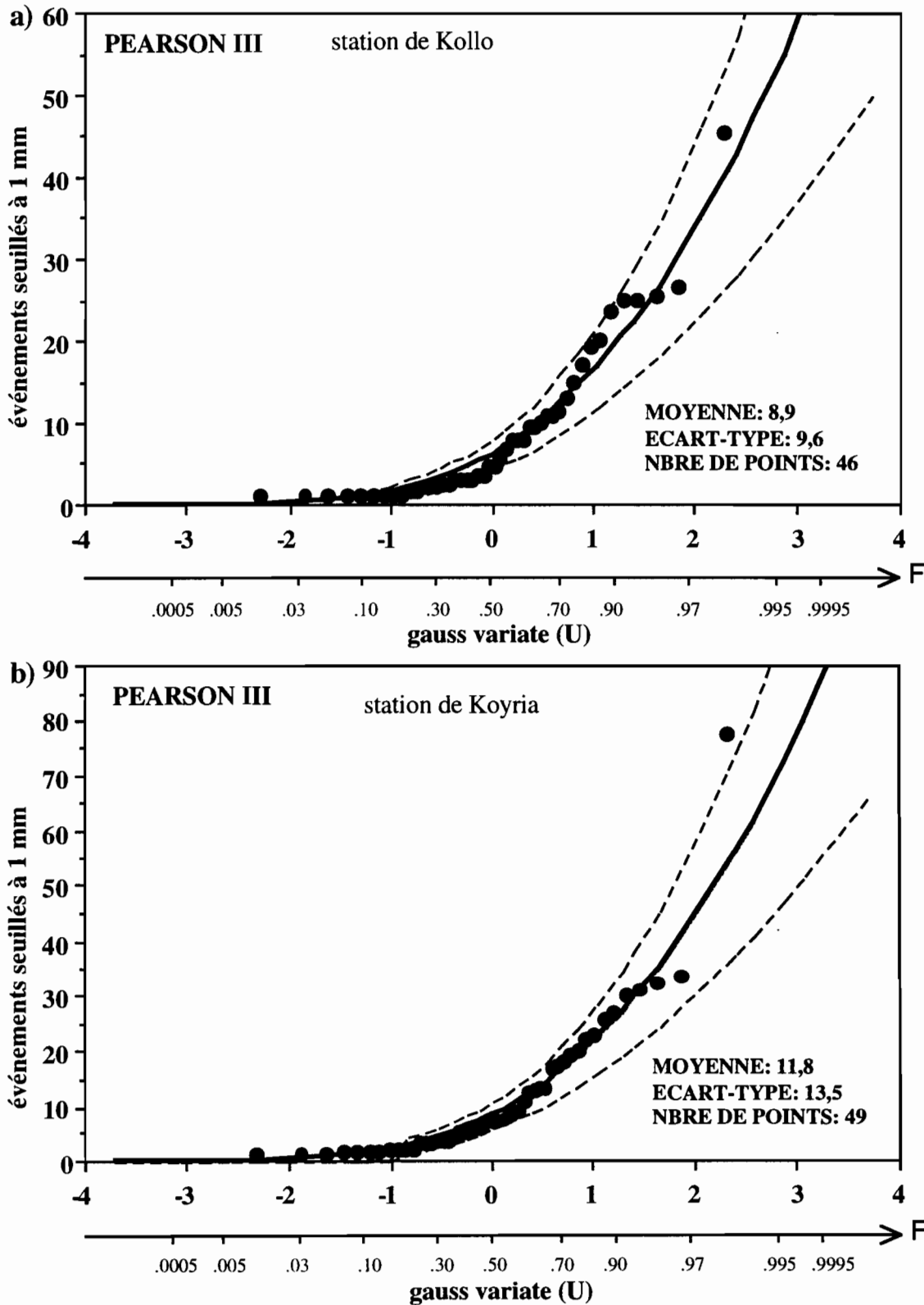
Figure 25: Loi de distribution des cumuls seuillés à 1 mm pour la station de Kollo (a) et de Koyria (b).
