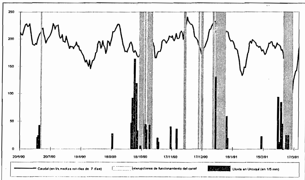
Figura 8 Evolución del caudal en el reservorio (medias móviles en 7 días, sin tener en cuenta los valores nulos debidos a las interrupciones de funcionamiento)
