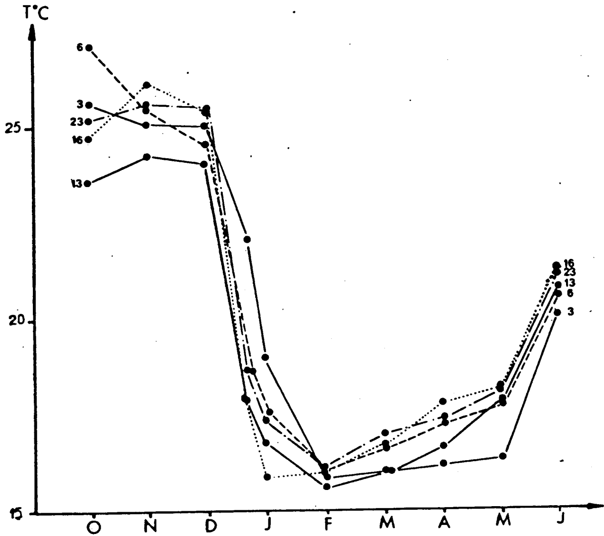
Fig.16 - Variation dans le temps de la température moyenne de la colonne d'eau aux stations 3,6,13,16 et 23.
