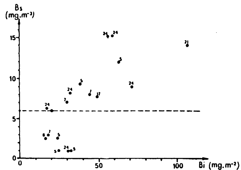
Fig. 53 - Rapport biomasse de surface (Bs)/biomasse intégrée (Bi). Les numéros indiquent les stations.
