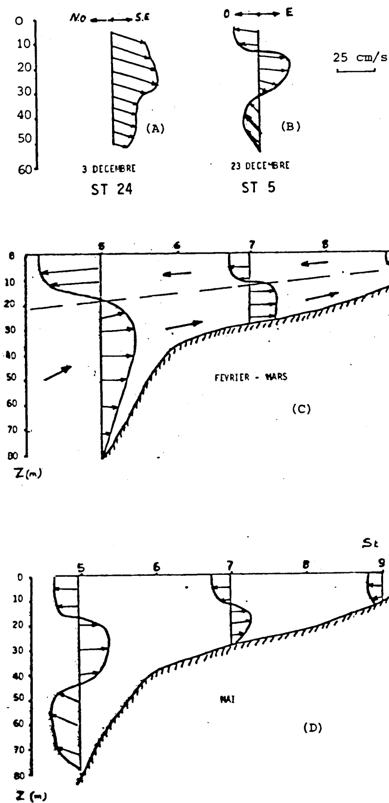
Fig.37 - Distribution verticale des vitesses de courant.
