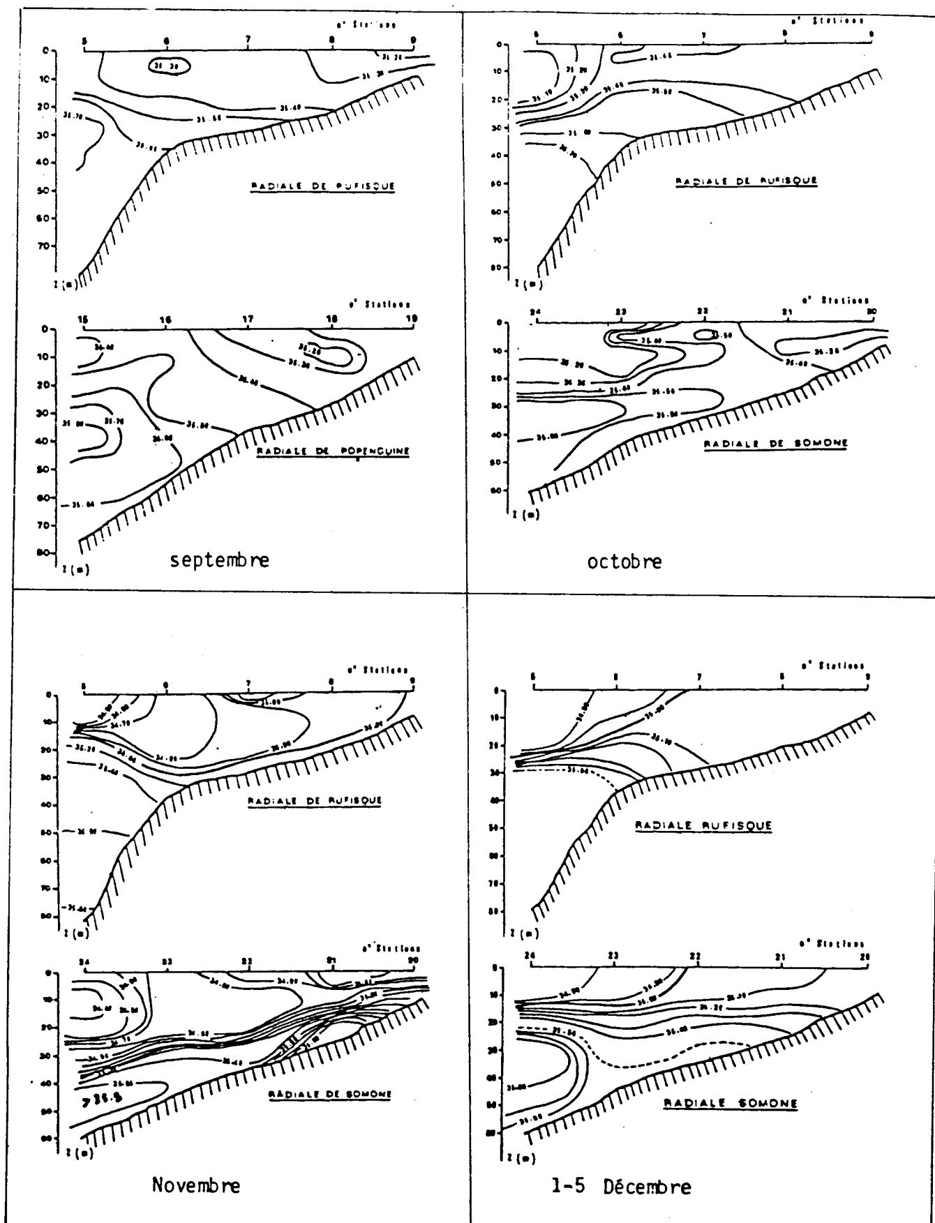
Distribution verticale de la salinité.
