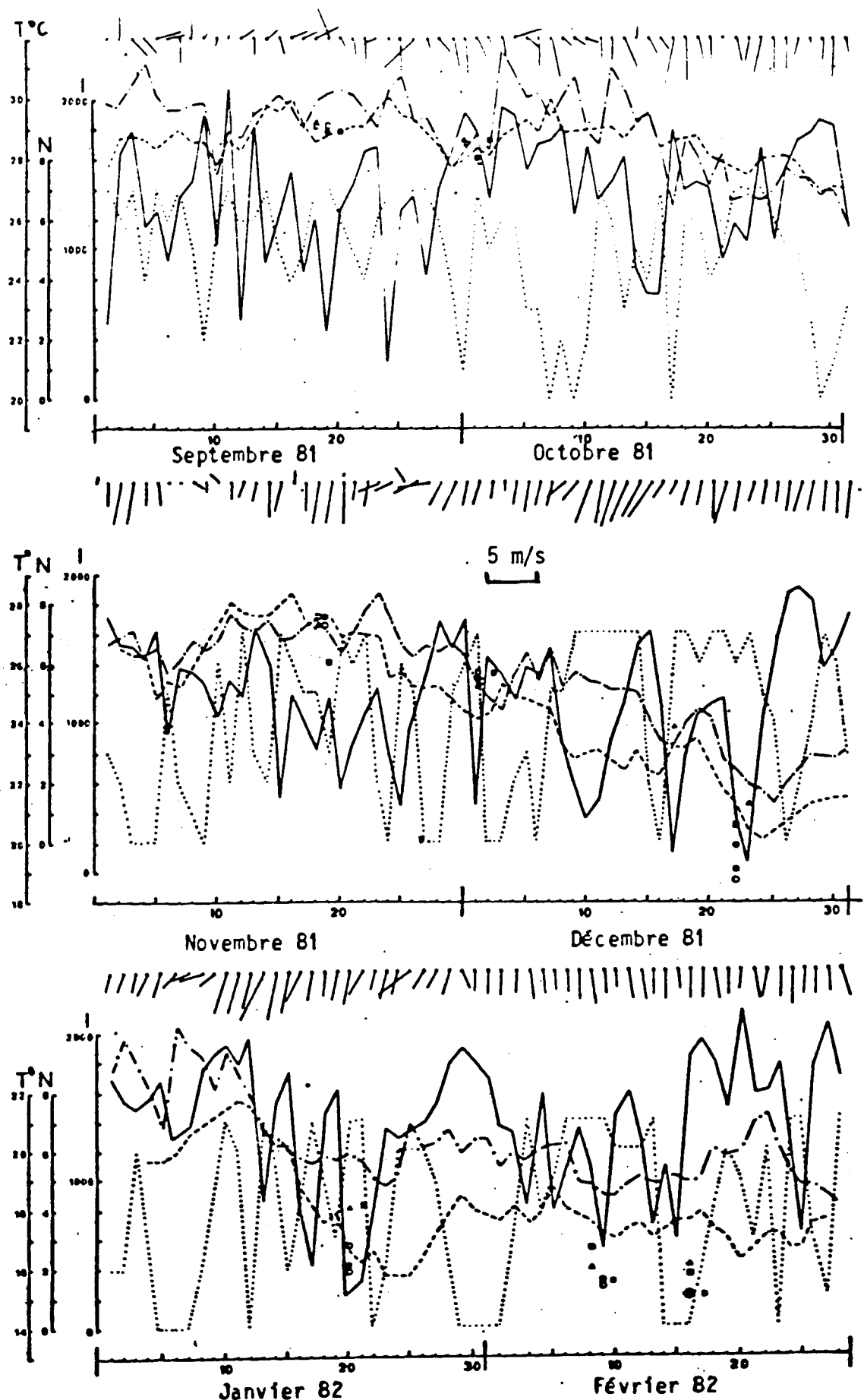
Fig.7a Variation temporelle de la température de l'air ( T_a ---), de la température de l'eau ( T_w ---), de la nébulosité ( N ....) et de l'insolation ( I —) aux stations côtières de Dakar-Yoff et Thiaroye/mer. Les valeurs de la température de surface à quelques stations du large ( \blacktriangle -st.2; \blacksquare -st.8; \bullet -st.9; \circ -st.10; \bullet -st.21) sont également indiquées.
