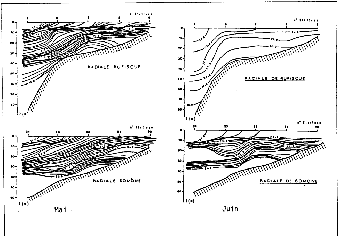
Distribution verticale de la température.
