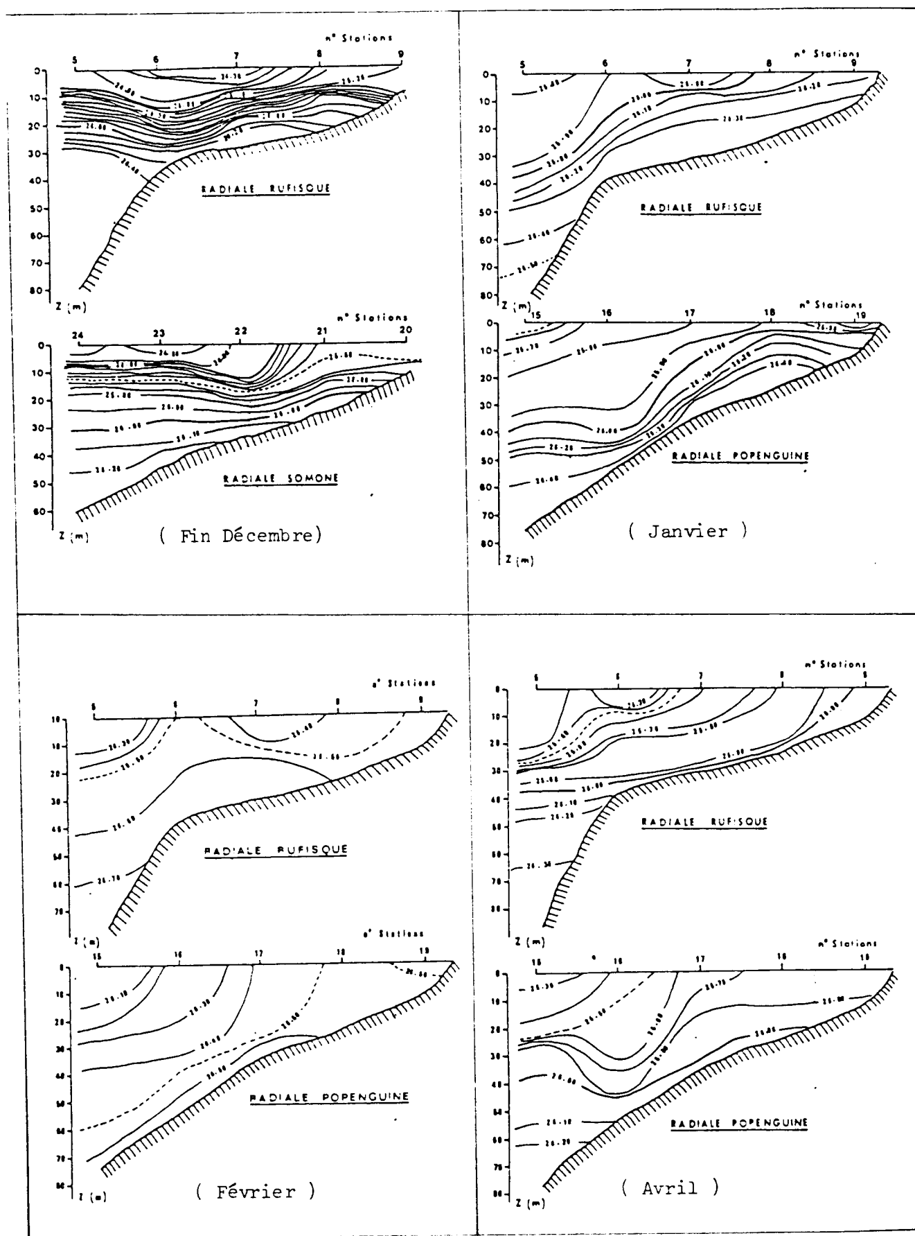
Fig. 14 - Répartition verticale de la densité.
