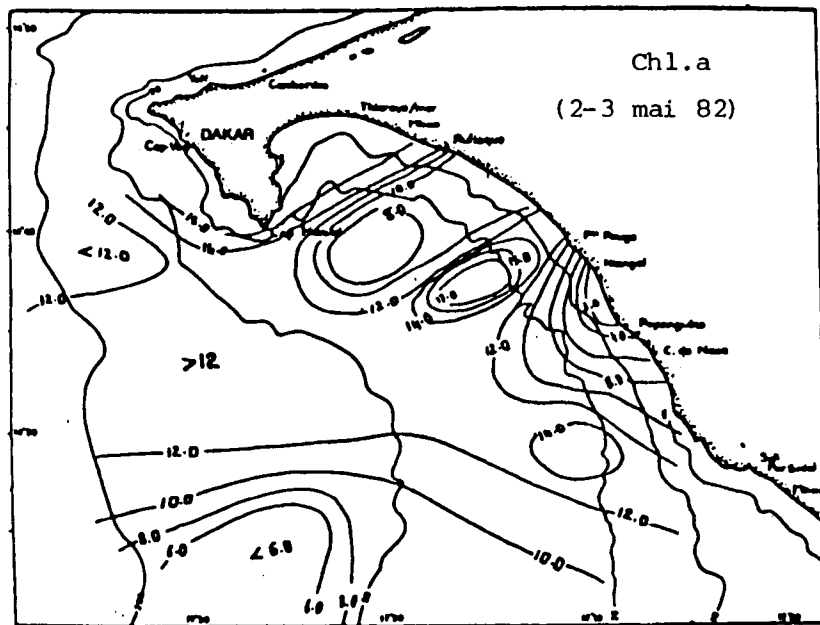
Fig. 46 - Distribution en surface des concentrations de chlorophylle a et du pourcentage de saturation en oxygène.
