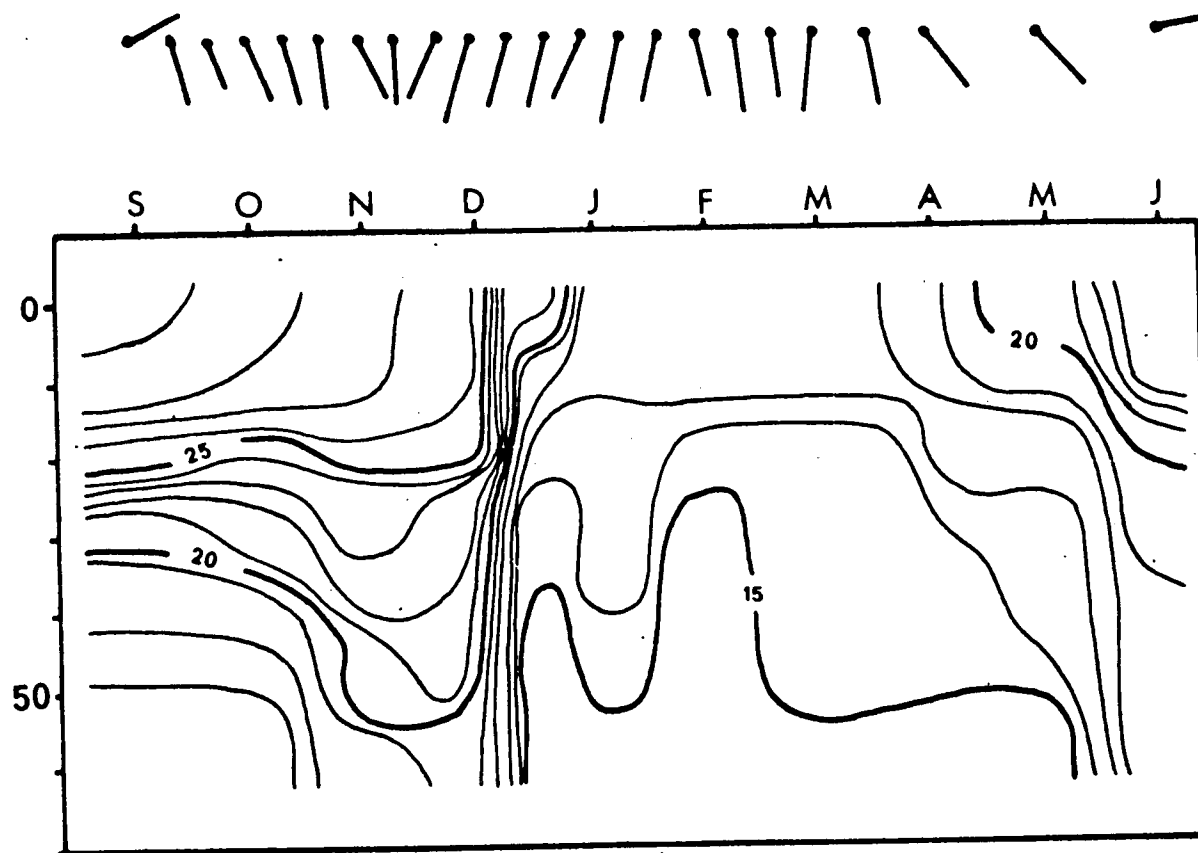
Fig. 10 - Variation dans le temps du profil de température à la station 5 en relation avec les moyennes décadaires des vents.
