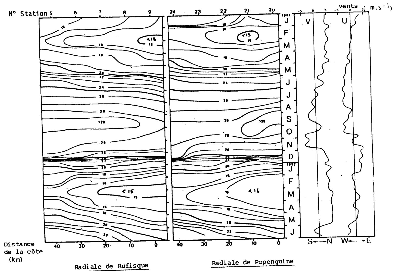
Fig. 8 - Variation dans le temps de la température de surface le long des radiales de Rufisque et de Popenguine-Somone en relation avec les composantes horizontales de la vitesse du vent.
