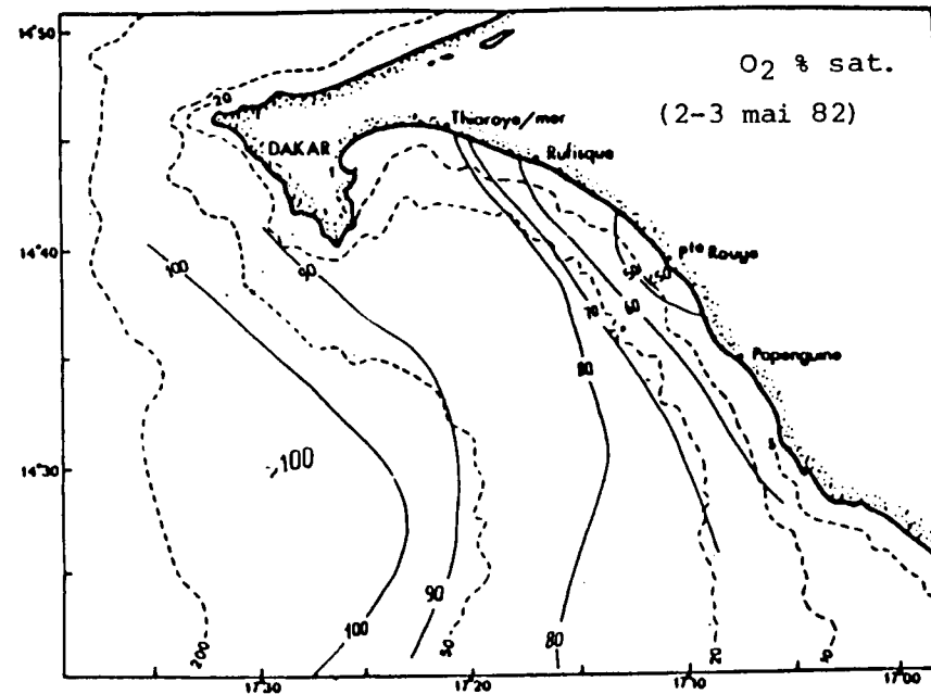
Fig. 46 - Distribution en surface des concentrations de chlorophylle a et du pourcentage de saturation en oxygène.
