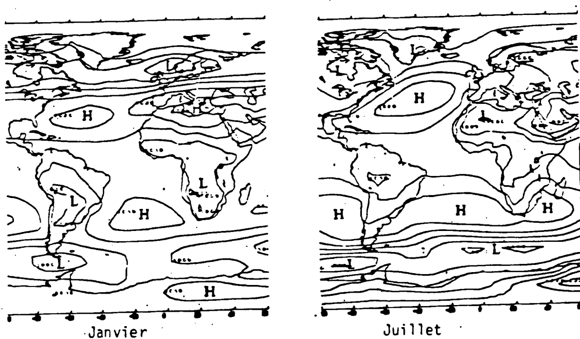
Fig. 4 - Champ de pression au niveau de la mer (D'après le rapport annuel du Laboratoire de Météorologie Dynamique de Palaiseau 1980)
