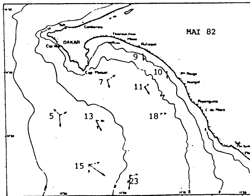
Fig.36 - Distribution horizontale des courants. Les numéros indiquent les stations.
