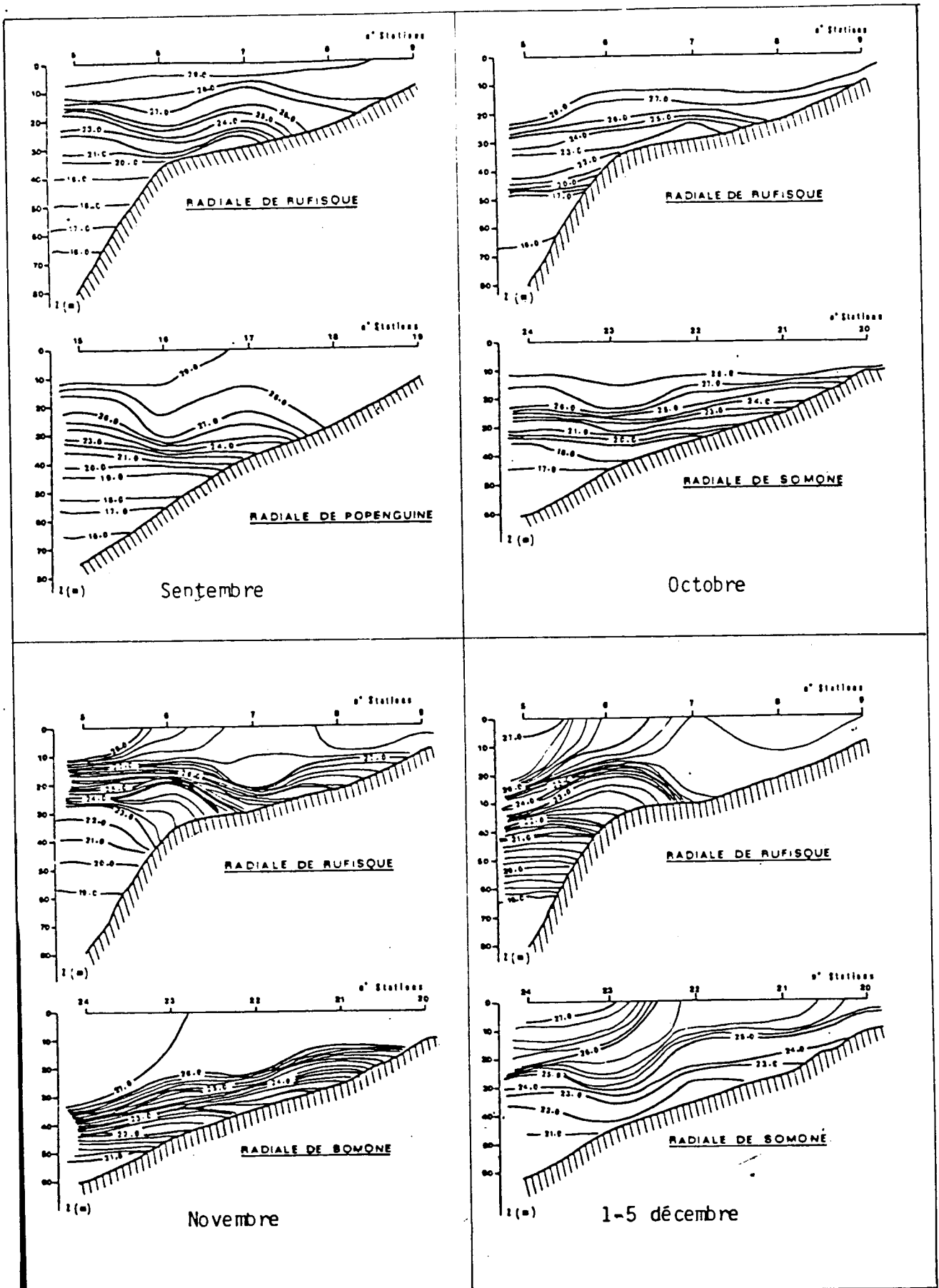
Distribution verticale de la température.
