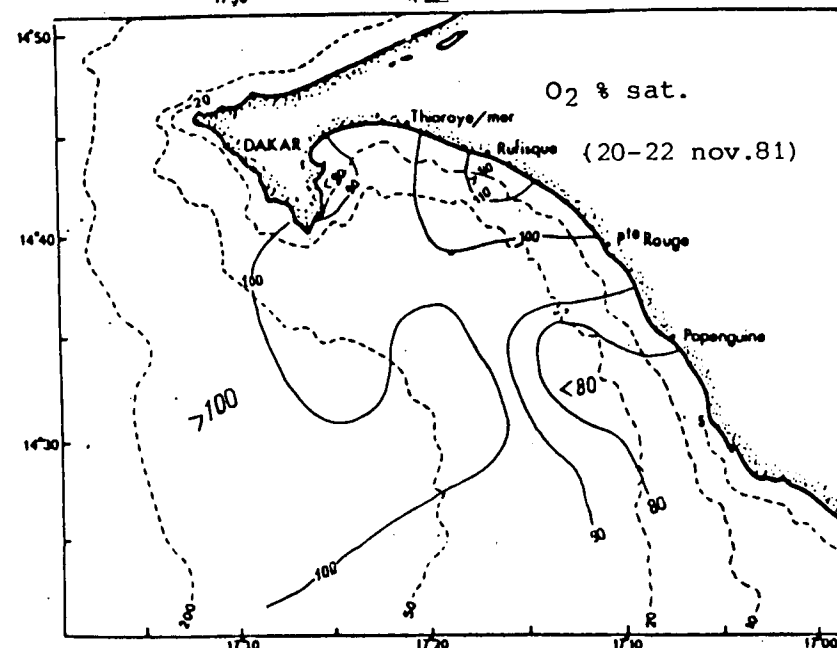
Fig. 44 - Distribution en surface des concentrations de chlorophylle a et du pourcentage de saturation en oxygène.
