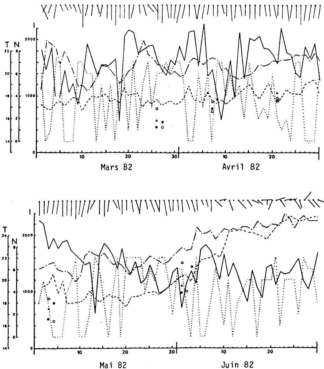
Fig. 7b - Variation temporelle de la température de l'air ( T_a - - -) de la température de l'eau ( T_w - · - ·), de la nébulosité ( N ...) et de l'insolation ( I —) aux stations côtières de Dakar-Yoff et Thiaroye/mer. Les valeurs de la température à quelques stations du large ( \blacktriangle - st.2; \square - st.8; \bullet - st.9; \circ - st.10; \blacksquare - st 21) sont également indiquées.
