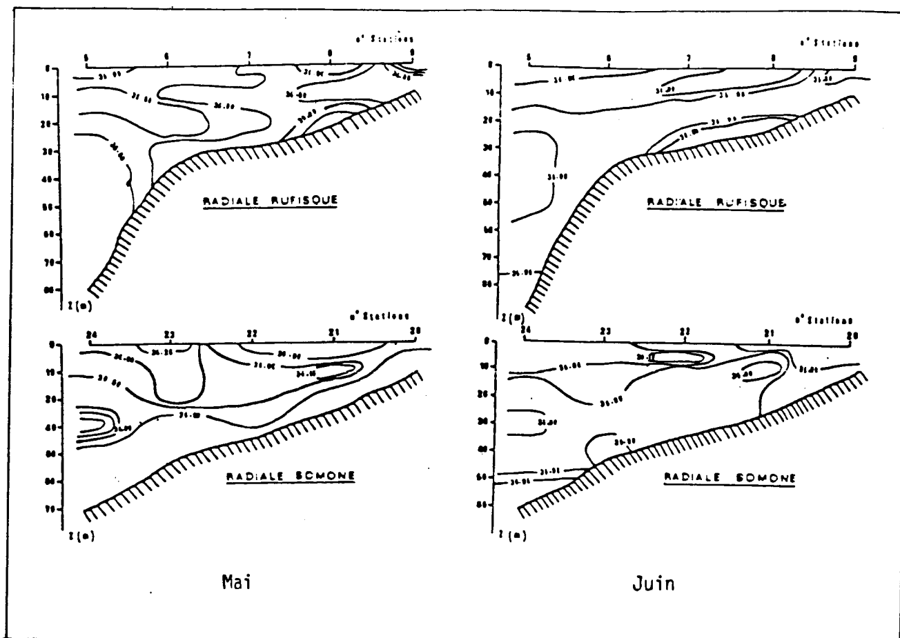
Distribution verticale de la salinité.
