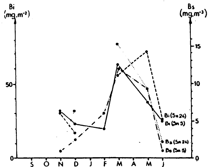
Fig. 52 - Variation temporelle de la chlorophylle intégrée (Bi) et de la biomasse de surface (Bs) aux stations 5 et 24.
