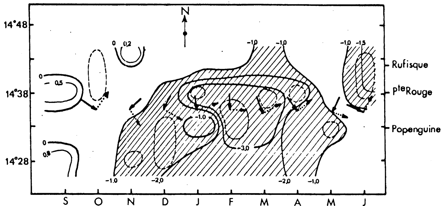
Fig. 27 -Variation mensuelle de l'écart de température entre les eaux de surface au dessus des fonds de 75 m et celles de la côte. Les valeurs négatives ( surfaces hachurées ) représentent une baisse de température des eaux superficielles côtières par rapport à celles du large alors que les positives indiquent le contraire. Les courants sont eux mesurés.
