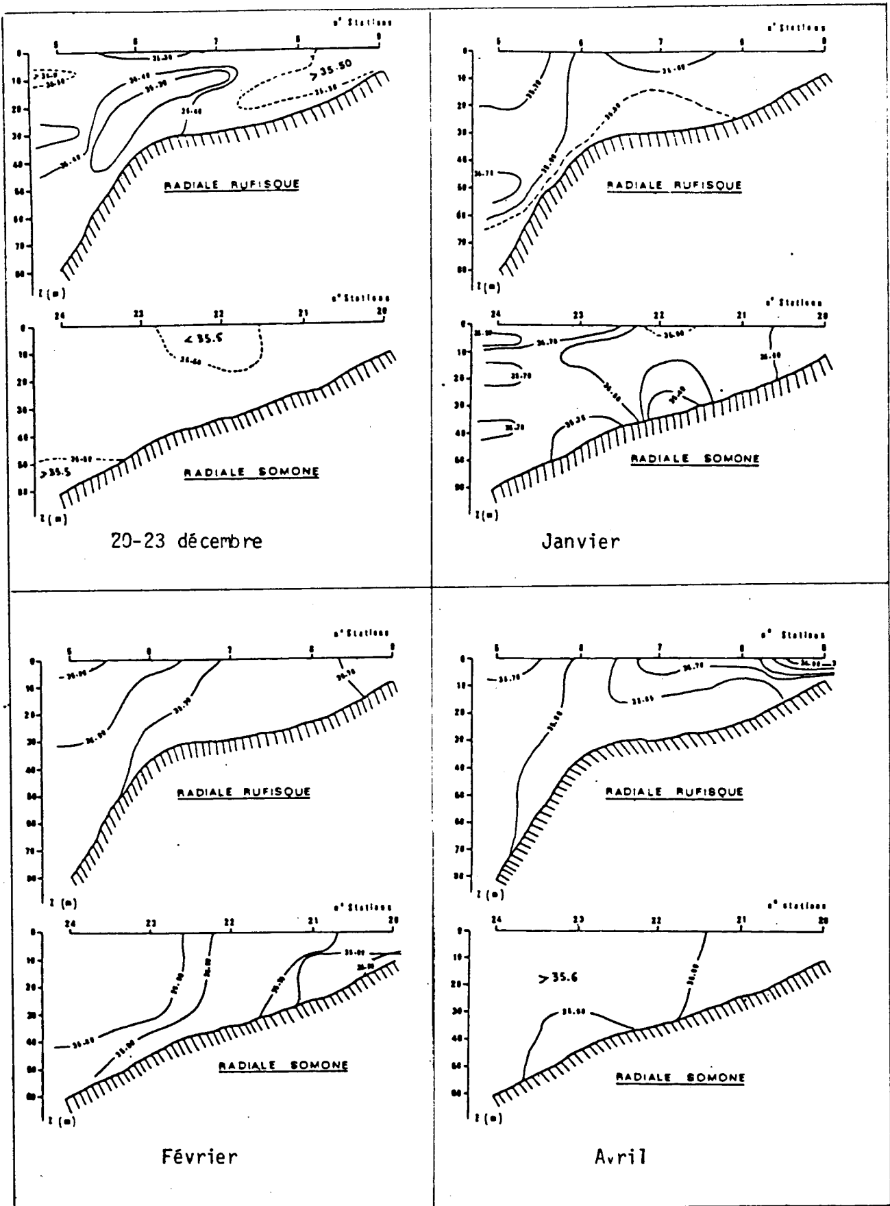
Distribution verticale de la salinité.
