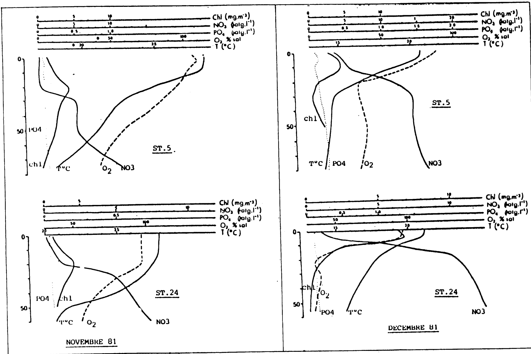
Fig.48 - Distribution verticale de la chlorophylle a , des phosphates, des nitrates, de la température et du pourcentage de saturation en oxygène.
