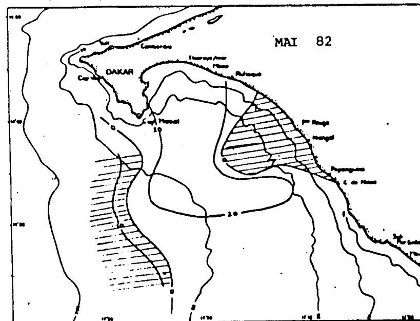
Fig.38 - Distribution en surface des vitesses verticales (W.en \text{cm/s } 10^{-4} ). Les valeurs négatives (surfaces hachurées) indiquent les mouvements verticaux ascendants.
