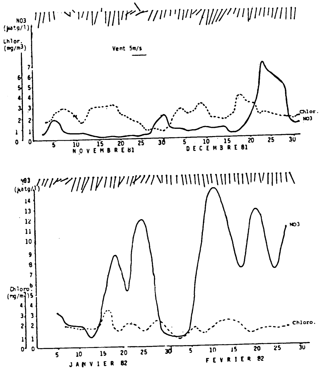
Fig. 51 - Distribution temporelle des valeurs moyennes lissées des concentrations de nitrates (—) et de la chlorophylle a (---) de surface à la station côtière de Thiarye en relation avec les vents journaliers de Dakar-Yoff.
