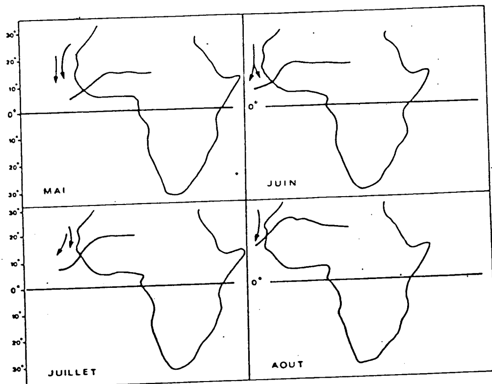
Fig. 3 Positions moyennes du Front Intertropical.
