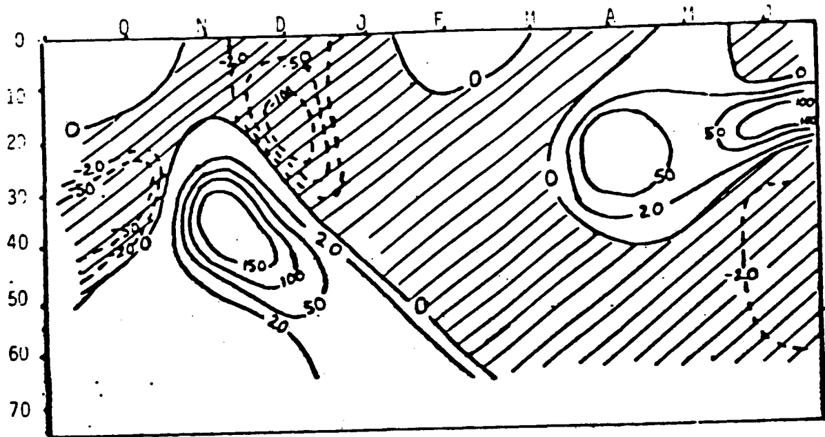
Fig.39 - Variation temporelle du profil des vitesses verticales à la station 5. Les valeurs négatives (surface hachurée) représentent les mouvements verticaux ascendants alors que les positives indiquent la descente des eaux. Les valeurs réelles ( \text{cm.s}^{-1} ) sont multipliées par 10^4 .
