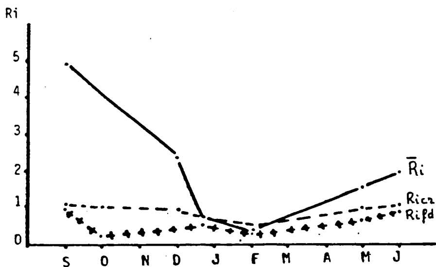
Fig. 42 - Variation temporelle à la station 5 du nombre de Richardson moyen de la colonne d'eau ( \bar{Ri} ), de la valeur critique de ce nombre ( Ricr ), et du nombre de Richardson de la couche profonde ( Rifd ).
