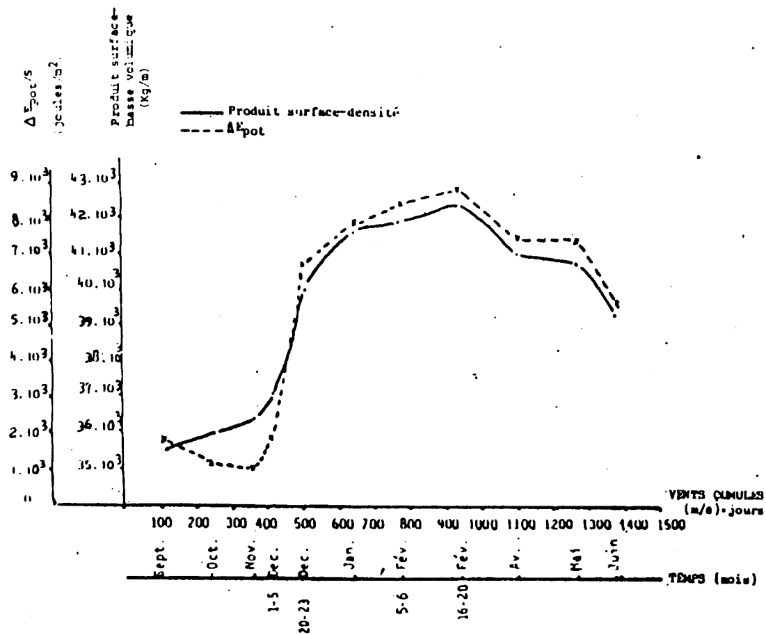
Fig. 41 - Variation simultanée dans le temps de l'énergie potentielle \Delta E_p et du produit surface- masse volumique en relation avec les vents cumulés.
