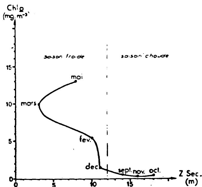
Fig. 43 - Relation entre les valeurs moyennes de la chlorophylle a dans la couche de surface (0-10m) et la profondeur de disparition du disque de Secchi ( Z_{sec.} ).
