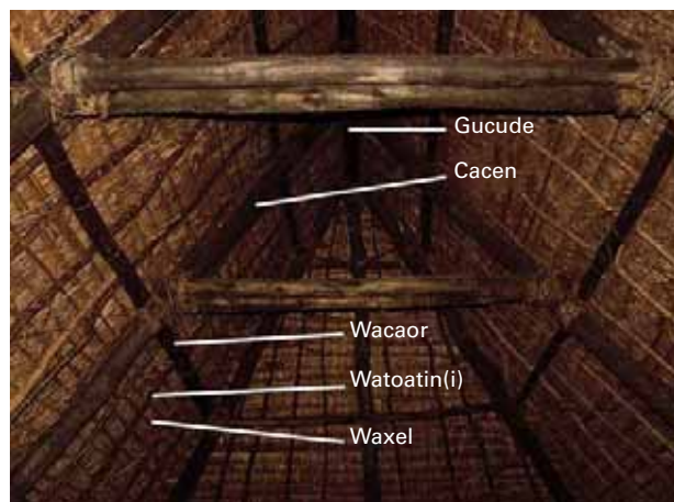
Charpente de mathaet (chez Pa Enare Bob, Nece).
