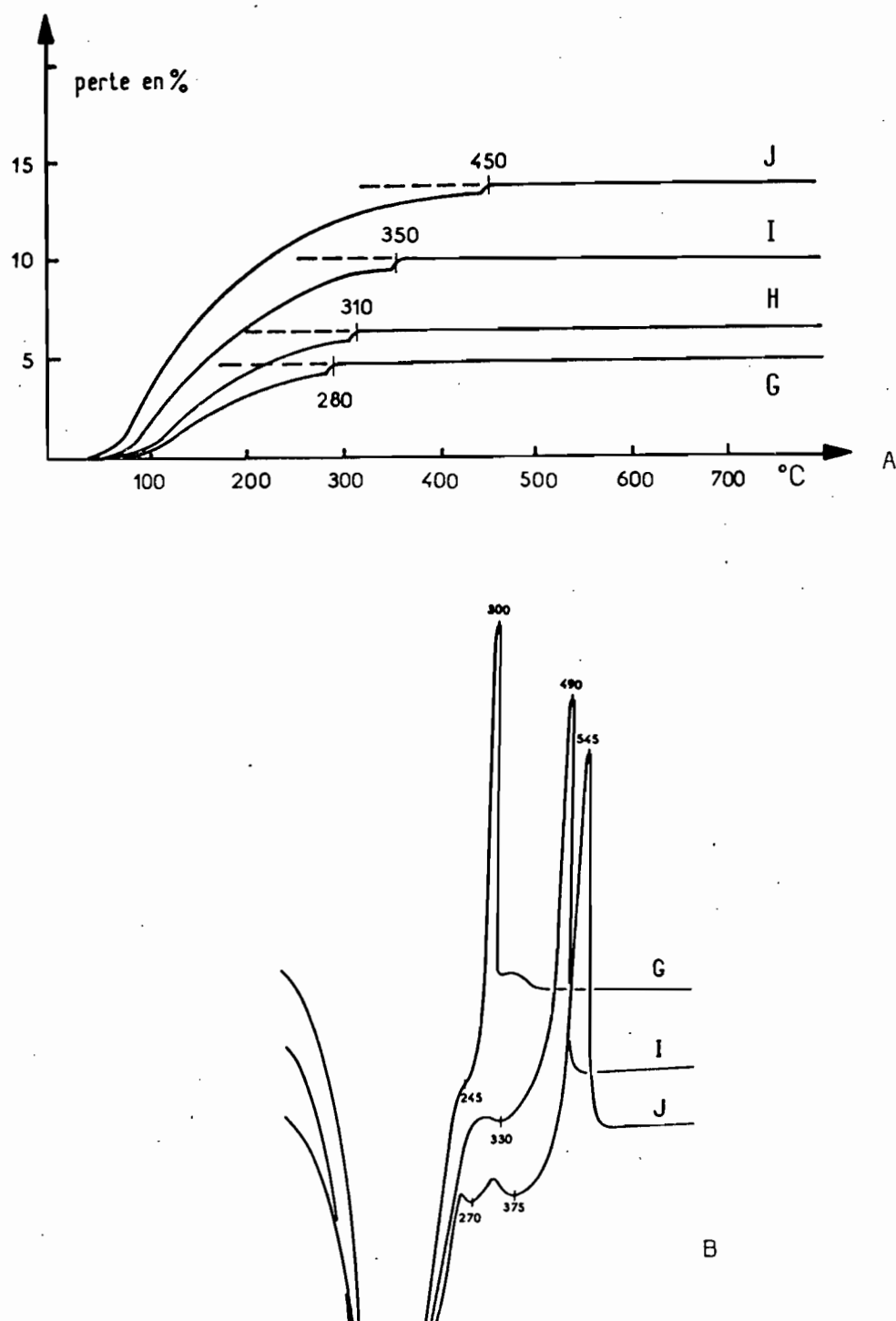
Fig. 35 - Résultats des échantillons obtenus pour une disponibilité en ions (OH)^- suffisante, puis lessivés pendant 100h , A : courbes thermo-pondérales des échantillons lessivés B : courbes d'analyse thermique différentielle des matériaux non lessivés .
