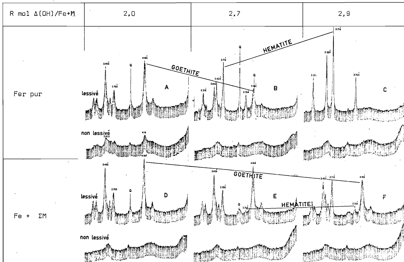
Fig. 31 - Diagrammes de rayons X des échantillons obtenus pour une disponibilité en ions (OH)^- limitée, puis lessivés pendant 100 h.
