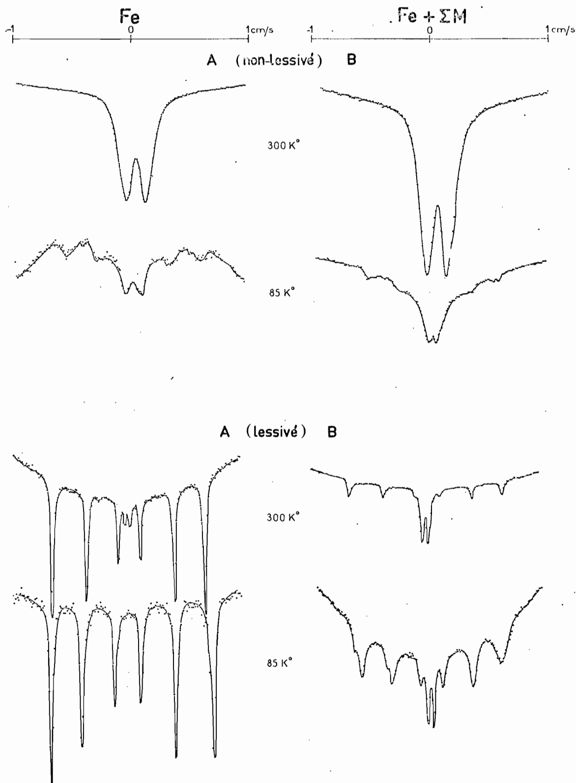
Fig. 37 - Spectres Mössbauer des échantillons obtenus pour une disponibilité en ions (OH)^- suffisante.
