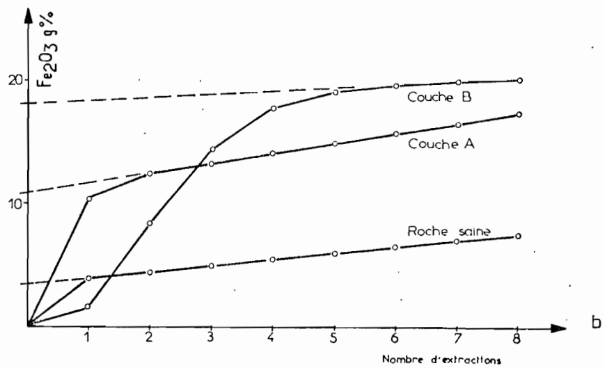
Fig. 2 - Caractéristiques de la roche R - 47 ; a : disposition des couches "pain d'épices", b : courbes cumulatives de la dissolution du fer au cours de l'attaque acido-basique.
