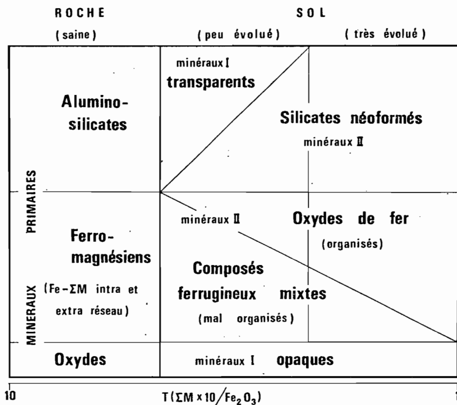
Fig. 40 - L'emplacement et la dynamique des éléments de transition au cours de la pédogenèse ; incidence sur la valeur du rapport T.
