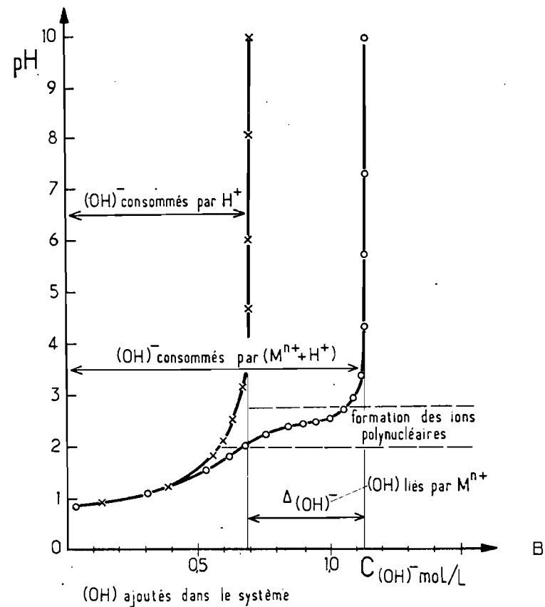
Fig. 13 - Courbes de titration pH/C_{(OH)^-} ; A : Système renfermant un ou deux ions simples ne formant pas d'espèces ioniques polynucléaires, B : Système composé de deux ions dont l'un donne des espèces ioniques polynucléaires.
