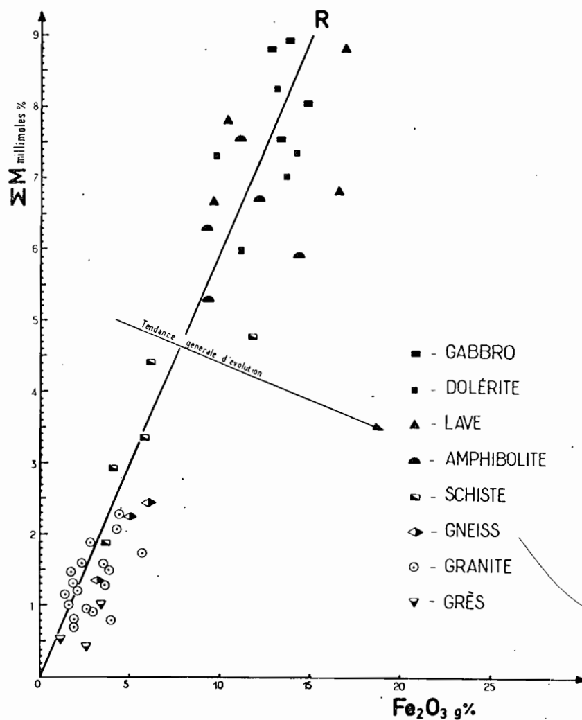
Fig. 3 - Répartition des roches saines en fonction de leurs teneurs en éléments du premier groupe de transition, (R représente le rapport T obtenu à partir de données existant dans la littérature).
