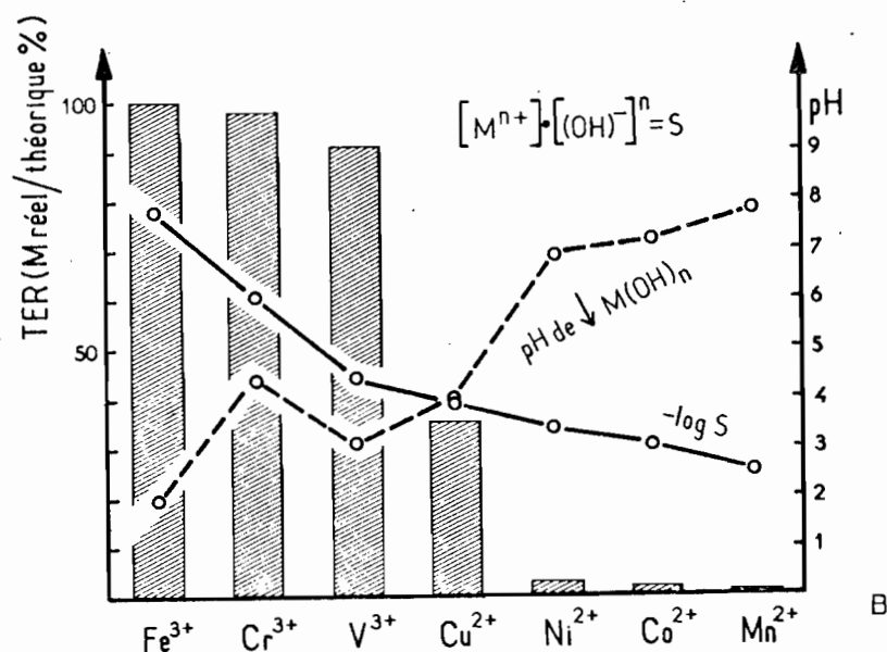
Fig. 36 - A : Variation du taux des éléments retenus (TER) à différents R \text{ mol } \Sigma M/Fe au départ. B : Corrélation entre TER, le produit de solubilité et le pH de l'apparition du précipité de l'hydroxyde des éléments de transition pour 10^{-2} \text{ M} en milieu chlorhydrique.
