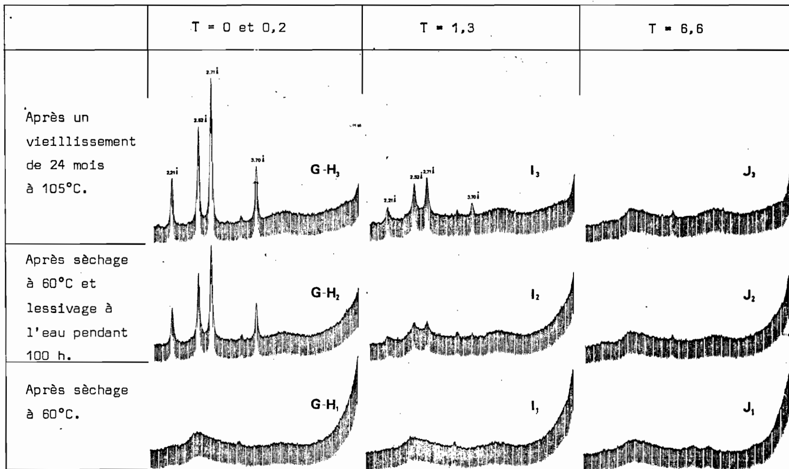
Fig. 34 - Diagrammes de rayons X des échantillons ayant un taux différent en éléments de \Sigma M obtenus pour une disponibilité en ions (OH)^- suffisante.
