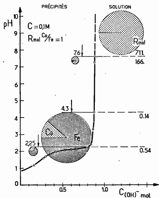
Fig. 20 - Courbes de titration pH/ C(OH)^- des systèmes binaires ( Fe^{3+} + M^{n+} ) ; composition des précipités et de la solution résiduelle.
