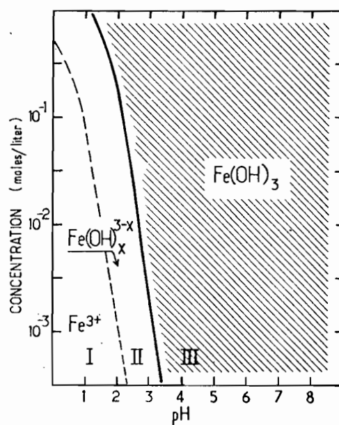
Fig. 15 - Domaine d'existence des différentes formes ioniques en équilibres avec l'hydroxyde \text{Fe(OH)}_3 pour des concentrations supérieures à 10^{-4} M et en présence de l'ion \text{Cl}^- . Les domaines I, II et III sont obtenus à partir des courbes \text{pH}/C_{(\text{OH})} (cf. Fig. 14).
