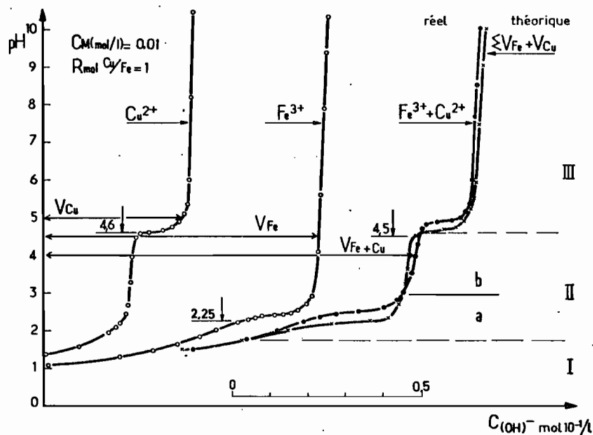
Fig. 21 - Courbes de titration \text{pH}/C_{(\text{OH})} des systèmes simples et binaires (réel et théorique) ; détermination graphique de la consommation en Ions (\text{OH})^- d'un système binaire.
