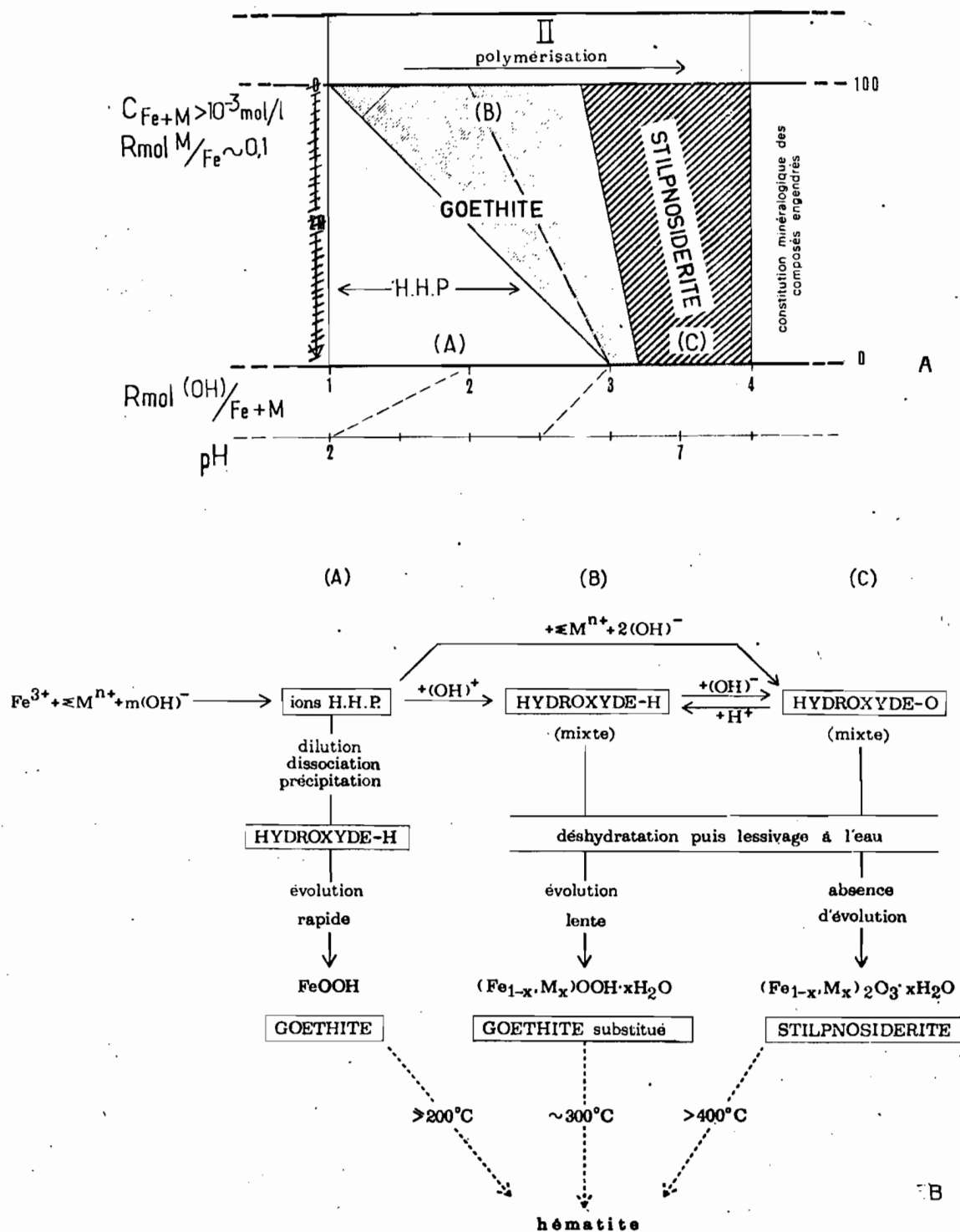
Fig. 39 - A : Domaine d'existence des différentes formes de composés mixtes en fonction de la disponibilité en ions (OH)^- du milieu. B : Relation entre les différentes formes sous lesquelles les composés mixtes se présentent.
