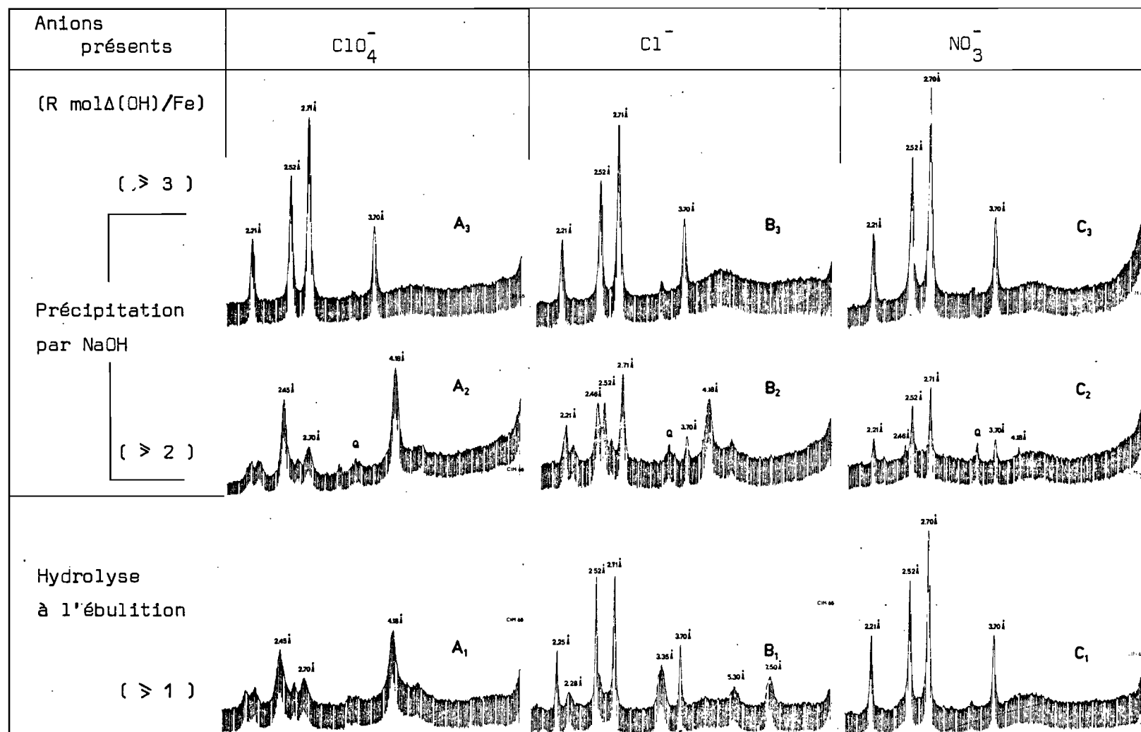
Fig. 28 - Diagrammes de rayons X des échantillons obtenus en présence de différents anions minéraux.
