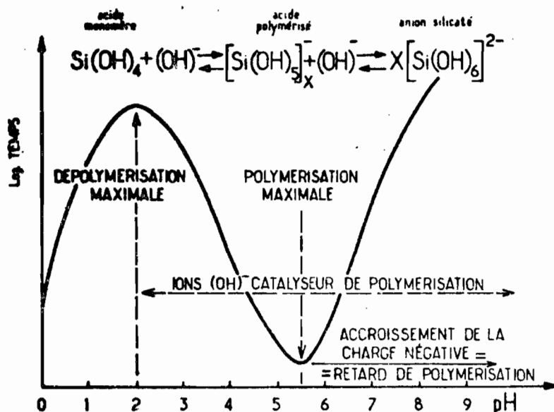
Figure 24 - Relation entre le pH d'une part et le degré et la vitesse de polymérisation d'autre part de l'anion silicate (d'après ILER - 1965).
