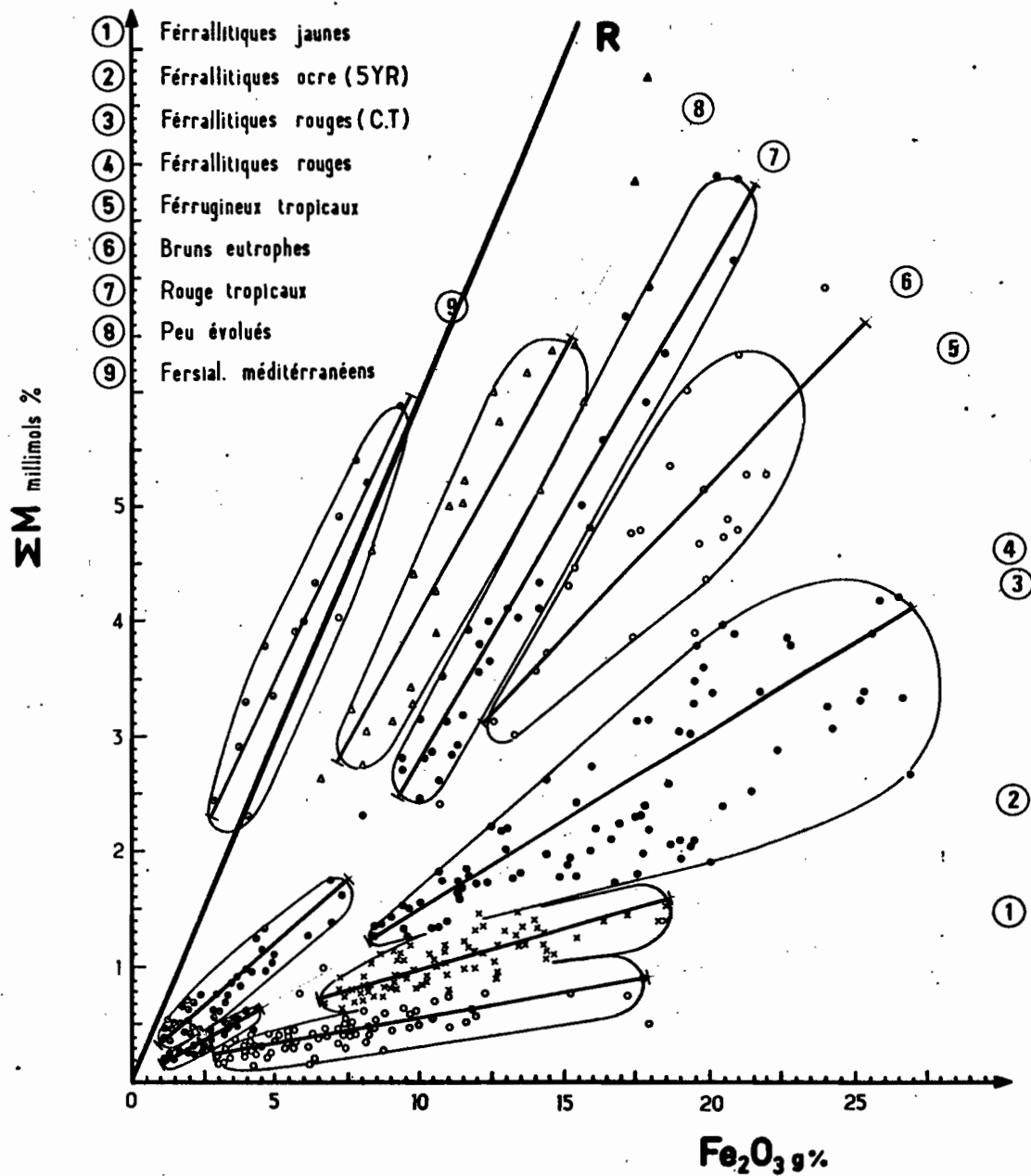
Fig. 41 - Les droites de régression de sols étudiés et les nuages des points correspondants.
