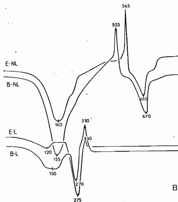
Fig. 32 - Résultats des échantillons obtenus pour une disponibilité en ions (OH)^- limitée, puis lessivés pendant 100h, A : courbes thermo-pondérales, B : courbes d'analyse thermique différentielle.
