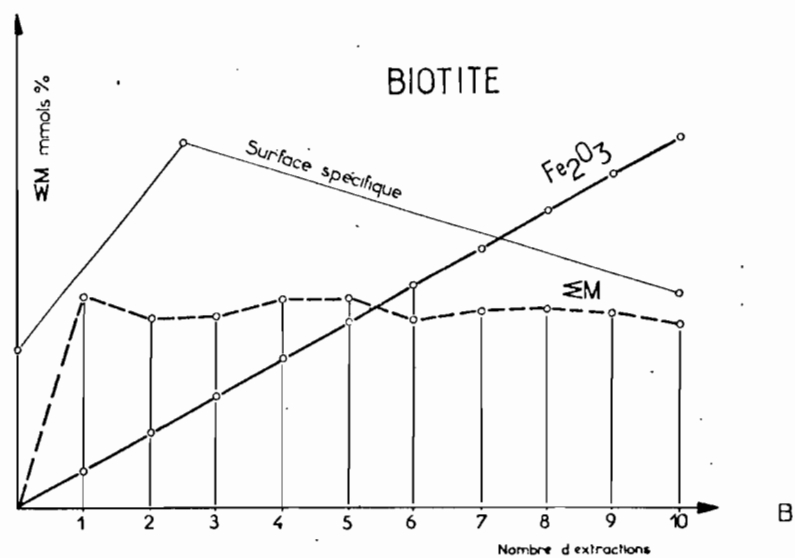
Fig. 1 - Comportement des éléments étudiés et de la surface spécifique au cours du traitement acido-basique des minéraux ferri-fères.
