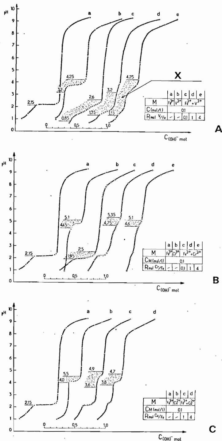
Fig. 18 - Courbes de titration pH/C (OH) des systèmes simples et binaires à différents R mol M/Fe ; (X = limites apparentes de la précipitation de l'hydroxyde).
