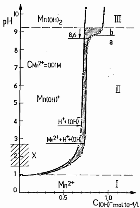
Fig. 16 - Courbes de titration pH/C (OH) des éléments traces de transition ; X = domaine d'existence des ions hydroxylés de fer (cf. Fig. 14).
