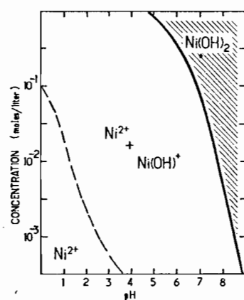
Fig. 17 - Domaine d'existence des différents formes ioniques des éléments traces de transition en équilibre avec leur hydroxyde M(OH)_n , en présence d'ion Cl^- .
