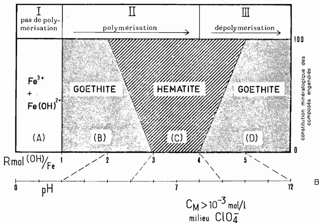
Fig. 38 - A : Equilibre entre les hydroxydes et les minéraux qui en résultent. B : Relation entre la composition minéralogique et la disponibilité en ions (OH) - du milieu.
