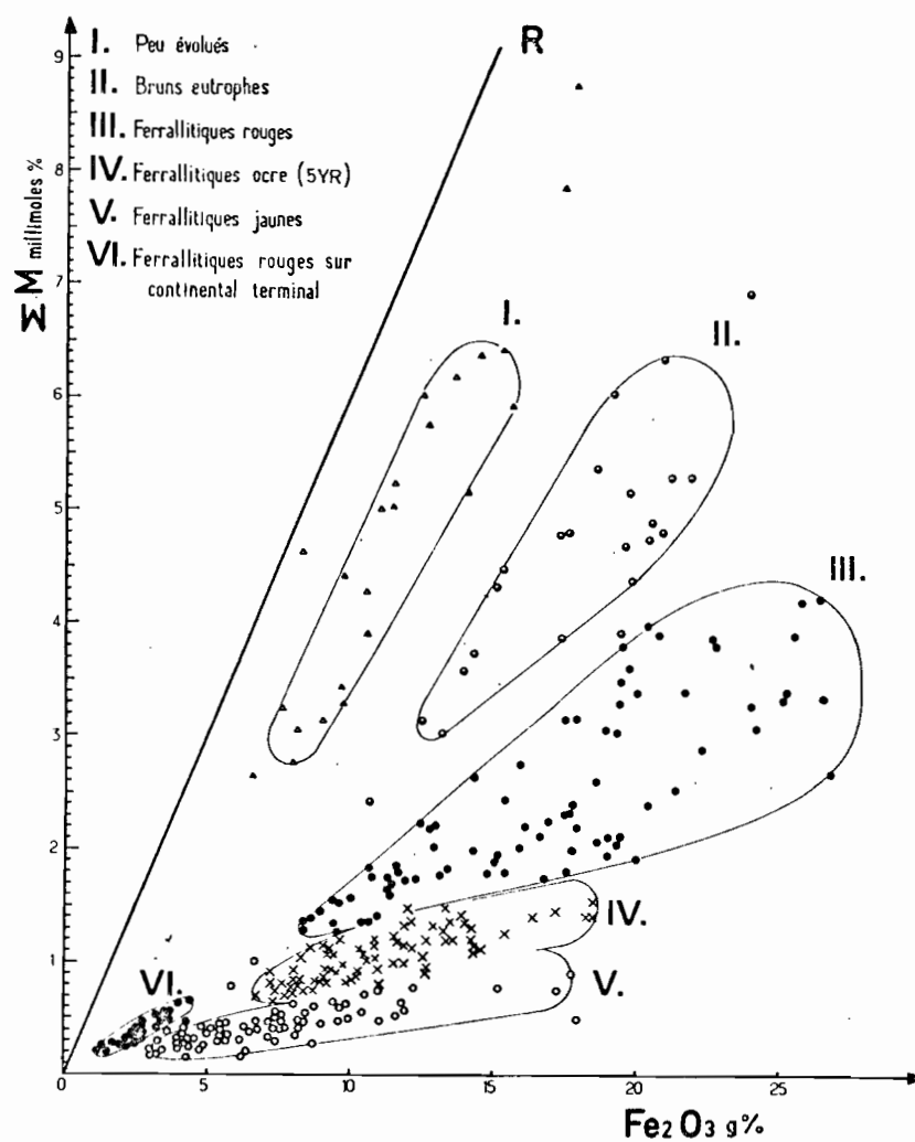
Fig. 6 - Répartition des sols des régions tropicales humides en fonction des paramètres \Sigma M et Fe_2O_3 .
