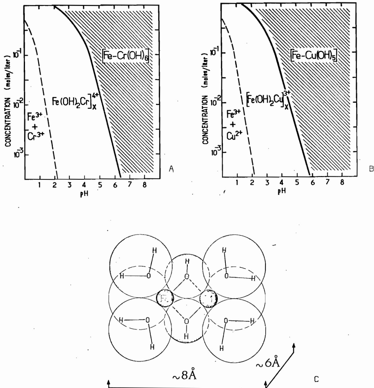
Fig. 23 - A et B : domaine d'existence des ions H.H.P., C : taille approximative d'un ion hydroxo- hétéro-dinucléaire des éléments de transition. (Pour la clarté du schéma, les deux molécules d'eau localisées à l'aplomb des cations métalliques n'ont pas été représentés).
