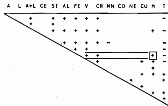
Fig. 9 - Corrélations de SPEARMAN pour les horizons B des sols ferrallitiques.
