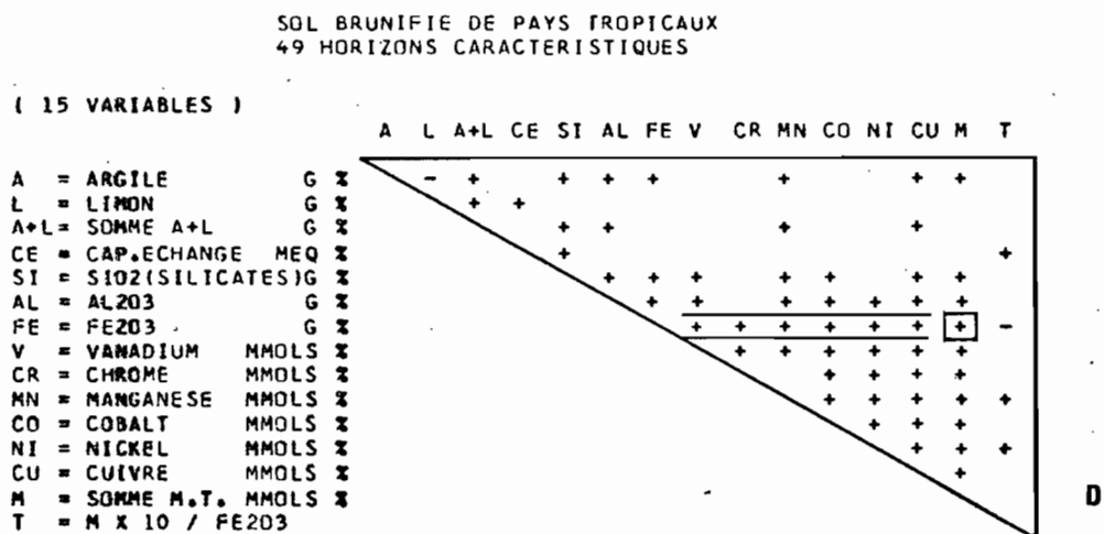
Fig. 8 - Corrélations de SPEARMAN pour les roches, les horizons d'altération ferrallitique et les horizons B des sols brunifiés de pays tropicaux.
