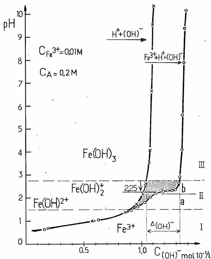
Fig. 14 - Courbes de titration \text{pH}/C_{(\text{OH})^-} d'un système \text{H}^+ et (\text{Fe}^{3+} + \text{H}^+) ; l'ion \text{Fe}^{3+} forme des espèces polynucléaires.
