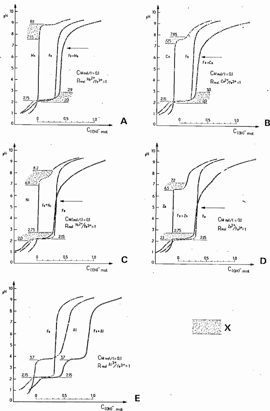
Fig. 19 - Courbes de titration pH/ C_{(OH)^-} des systèmes simples et binaires à différents R_{mol} M/Fe ; (X = limites apparentes de la précipitation de l'hydroxyde).
