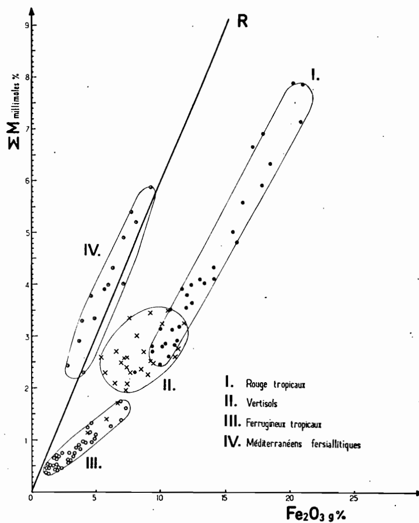
Fig. 7 - Répartition des sols des régions tropicales sèches et méditerranéennes en fonction des paramètres \Sigma M et Fe_2O_3 .
