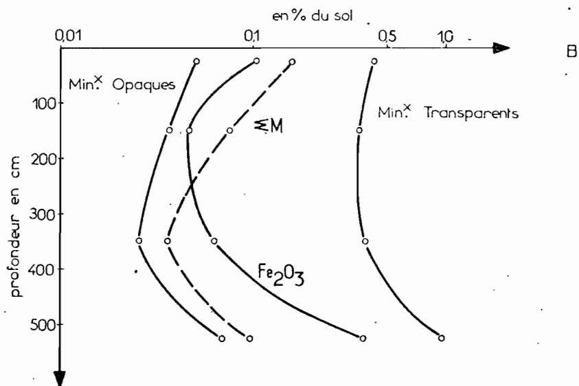
Fig. 4 - Teneur en minéraux primaires, en fer et en éléments traces de transition extraits de la fraction sable (> 50 μ) ; A : Sols ferrallitiques rouges (RM - 19), B : Sol ferrugineux tropical (TH - 7).
