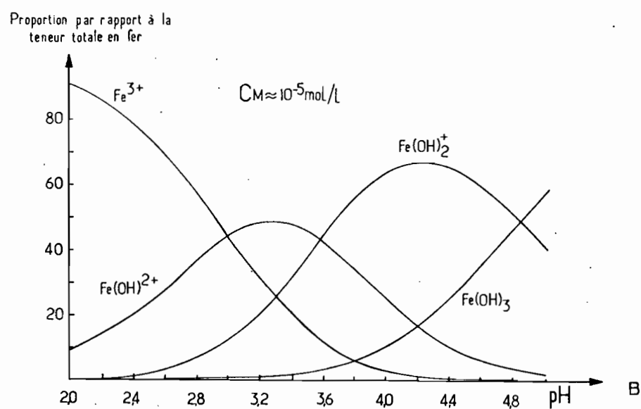
Fig. 12 - Domaine d'existence des différentes formes ioniques en équilibre avec l'hydroxyde \text{Fe(OH)}_3 ;
