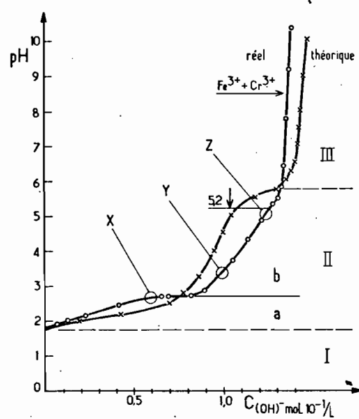
Fig. 22 - Situation des points d'arrêt au cours de la titration, auxquels la dilution est effectuée.
