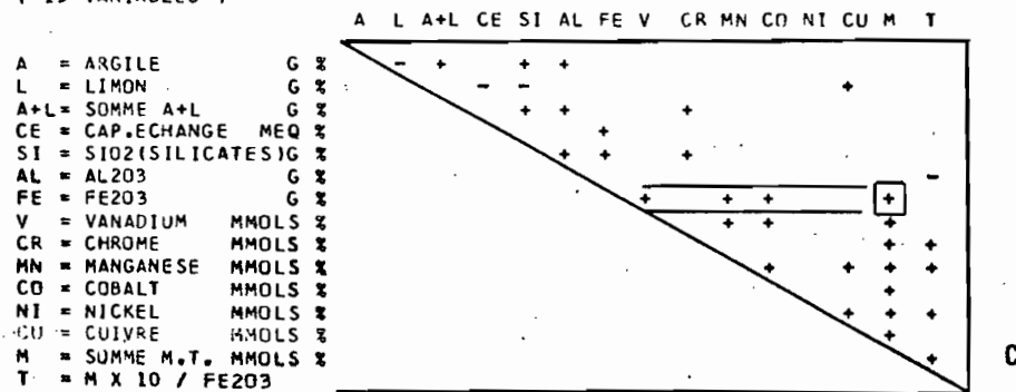
Fig. 10 - Corrélations de SPEARMAN pour les horizons B des autres sols des régions tropicales.
