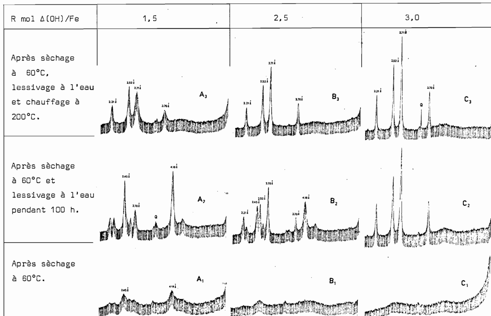
Fig. 27 - Diagrammes de rayons X des échantillons obtenus à différents R mol \Delta(\text{OH})/\text{Fe} .
