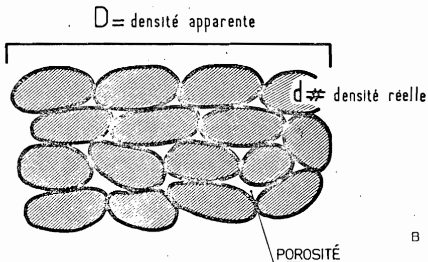
Fig. 30 - A : Variation de la taille moyenne des pores et de la porosité totale en cours du lessivage, B : Schéma de la macro-structure de l'hydroxyde de fer.
