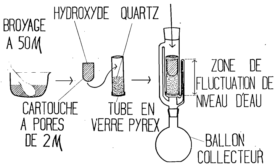
Fig. 25 - A : procédé utilisé lors de la préparation des échantillons étudiés, B : technique du lessivage à l'aide d'un extracteur "Soxhlet".
