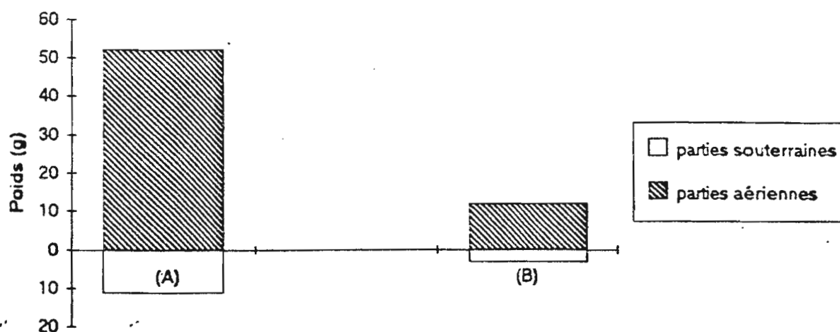
GRAPHIQUE 7 : Poids (g) des parties aériennes et souterraines de sorgho cultivé dans des seaux sur substrat prélevé sous F. albida (A) et hors de son couvert (B)
