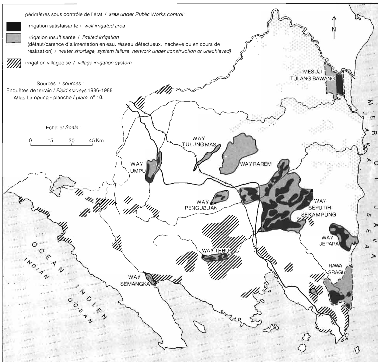
FIG. 20. RESEAUX D'IRRIGATION ET DE DRAINAGE - SITUATION EN 1987 IRRIGATION AND DRAINAGE NETWORKS - SITUATION IN 1987
