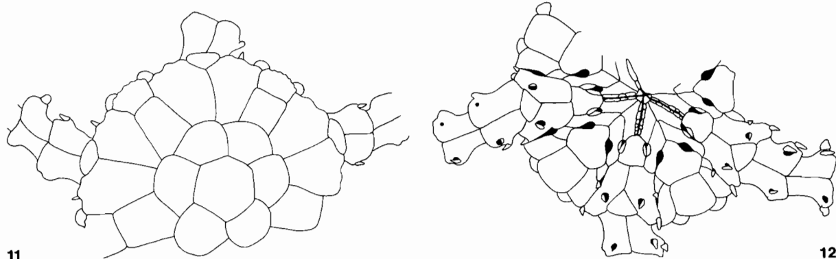
Fig. 11-12. — Anthophiura ingolfi Fasmer, BIOCAL, DW 46, d.d. = 3 mm
