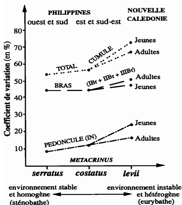
FIG. 5. — Variabilité des caractères morphologiques en fonction de l'hydrodynamisme chez Metacrinus serratus , M. costatus et M. levii . I N = nombre d'internodales par noditaxis ; IBr + IIBr + IIIBr = première, deuxième et troisième série brachiale.
