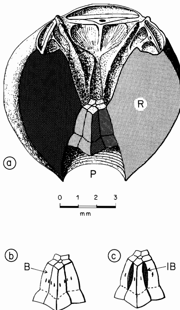
FIG. 8. — Architecture de la coupe dorsale de Caledonicrinus vaubani .
