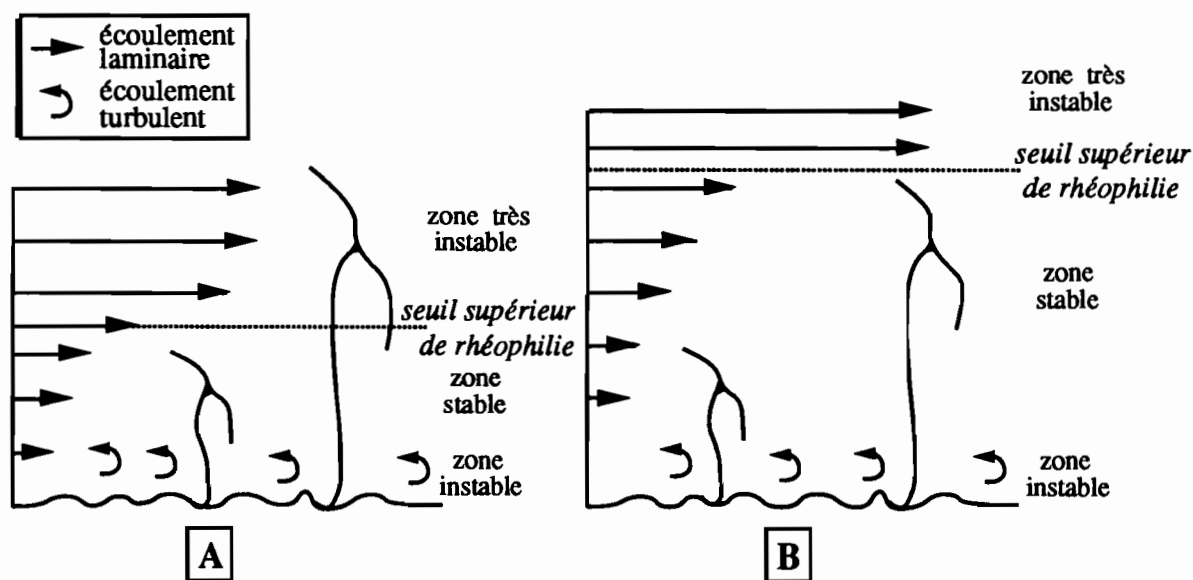
FIG. 4. — Modèle théorique liant la croissance des Metacrinus et l'hydrodynamisme.
