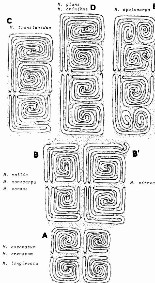
FIG. 35. — Les stades de complication des infundibula dans le genre Molguloides .
