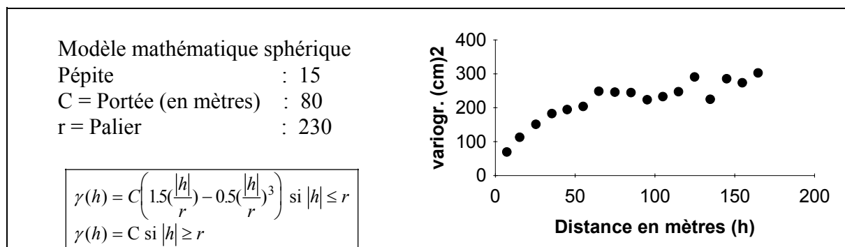
Figure VII-9. Variogramme omnidirectionnel de la hauteur des plants (1989). Groupe de parcelles 1.
