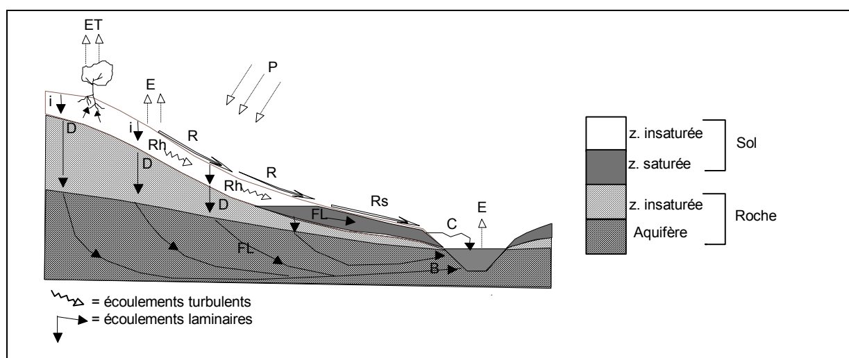
Figure I-11. Schéma qualitatif général de fonctionnement hydrodynamique d'un versant. D'après CHORLEY (1980), DUNNE (1980) et ATKINSON (1980).
