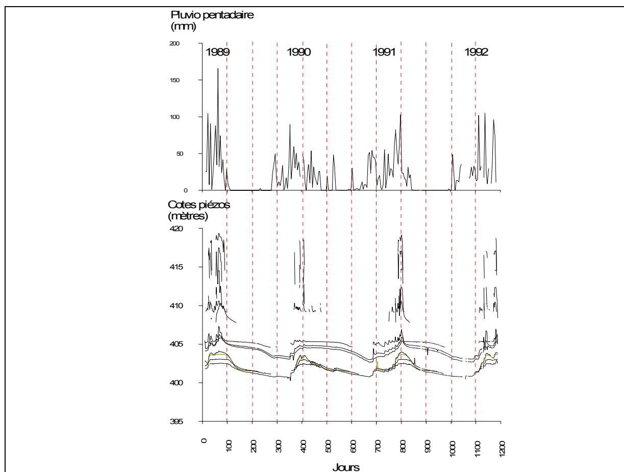
Figure V-6. Relevés piézométriques le long du transect et pluviométrie. Période 1989-1992
