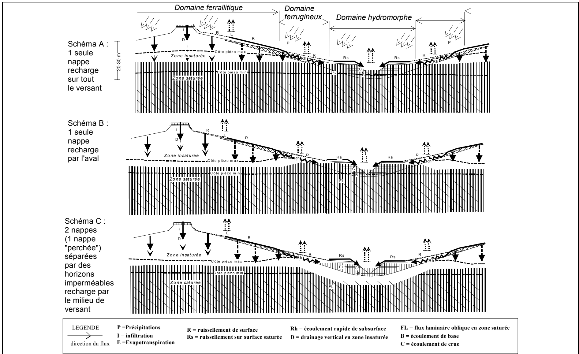
Figure I-12. Trois schémas possibles de fonctionnement hydrodynamique du versant-type.
