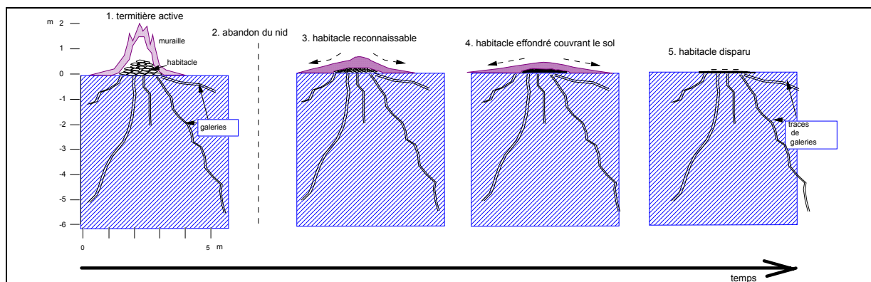
Figure III-19. Séquence d'évolution d'un nid de macrotermes créant une macroporosité tubulaire dans le sol.
