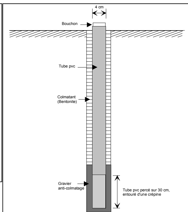
Figure V-5. Schéma d'un tube piézométrique.
