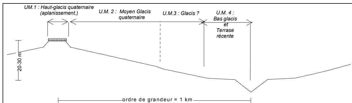
Figure I-7. Le modelé du versant-type
