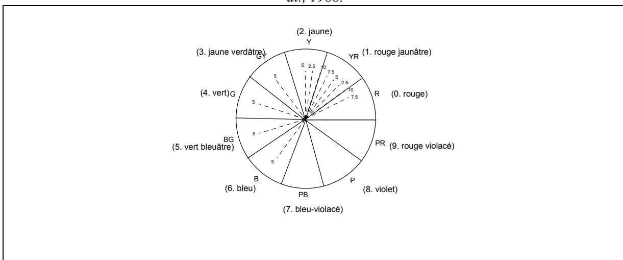
Figure A.7. Répartition des teintes Munsell sur le cercle colorimétrique.
