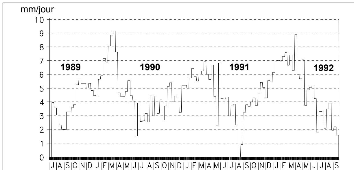
Figure III-4. Evaporation bac sur le site. Moyenne quotidienne par pentade. Période du 1.07.1989 au 31.09.1992.
