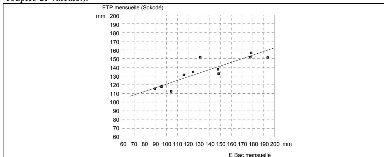
Figure III-5. Relation entre l'évaporation bac mesurée sur le site et l'ETP calculée à Sokodé.
