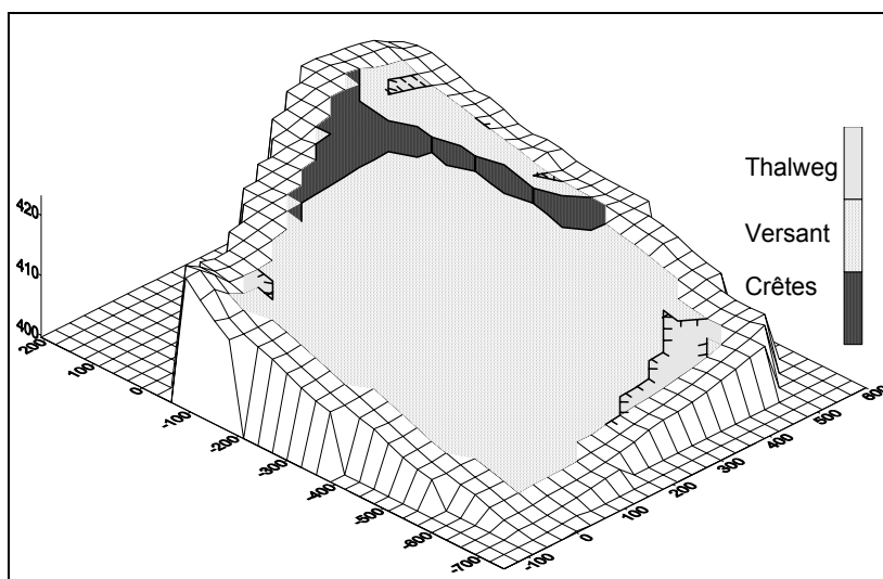
Figure III-10 : Bloc-diagramme des formes de terrain dérivées du modèle numérique de terrain.
