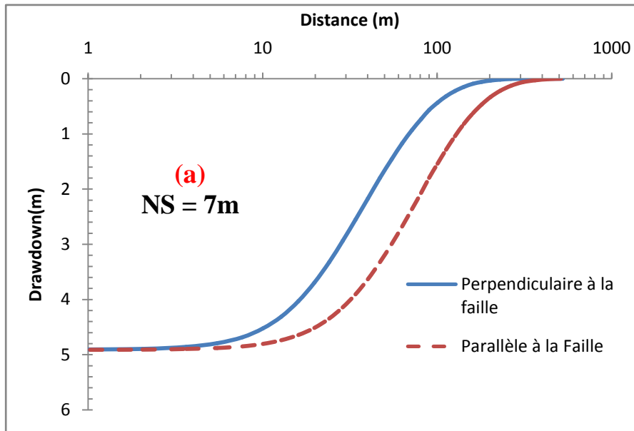
Figure 6.16 : Rabattement dans les altérites avec pompage dans la faille (cas 3) pour différents niveaux statiques. A gauche, niveau statique 7 m; à droite niveau statique 0 m (l'eau est sub - affleurante).
