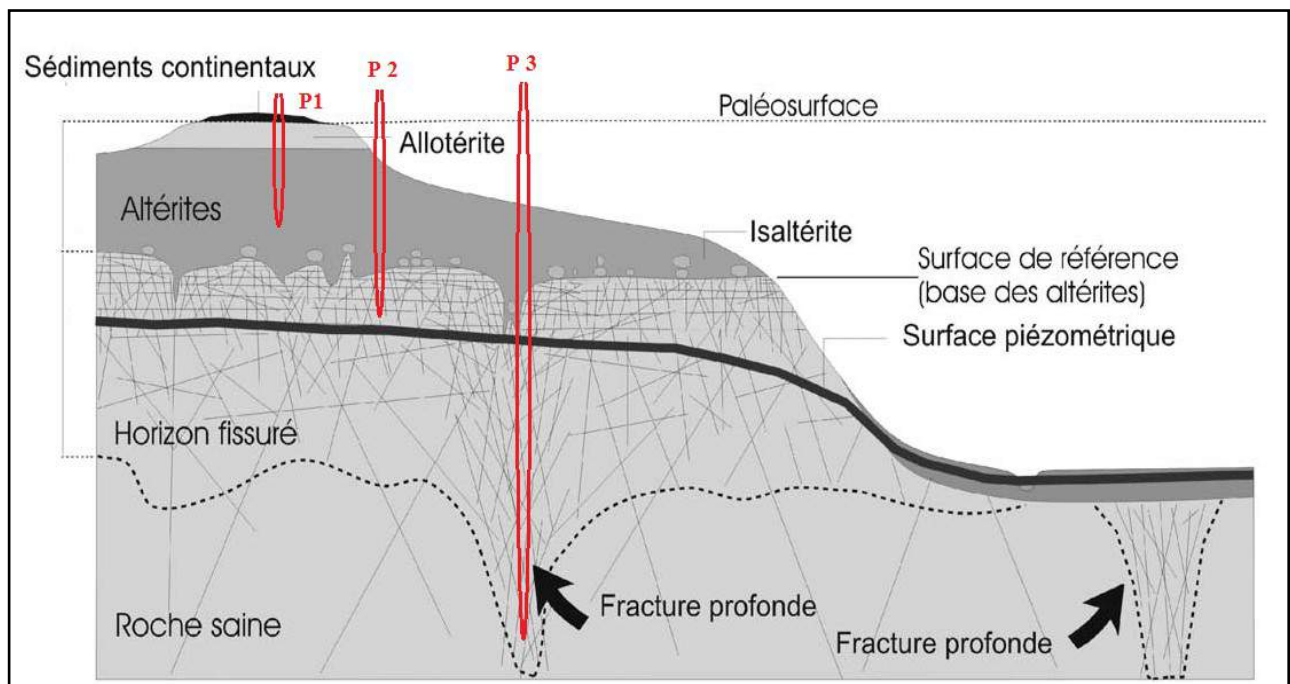
Figure 6. 3 : Illustration des 3 cas de pompage modélisés.
