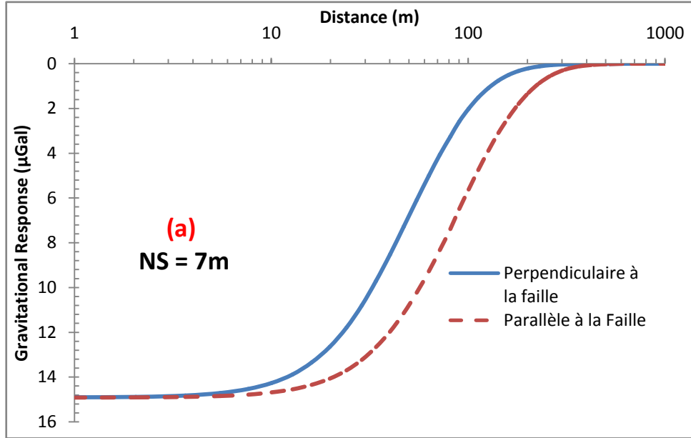
Figure 6. 17 : Courbes des signaux gravimétrique pour des pompages dans la faille avec différents niveaux statiques initiaux. A gauche, niveau statique 7 m; à droite niveau statique 0 m.
