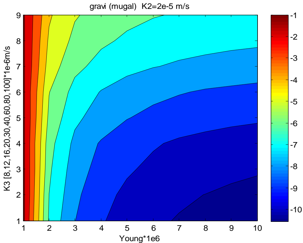
Figure 6.20 : Variation de la réponse gravitationnelle ( \mu\text{gal} ) en fonction de la conductivité K_3 et du module de Young en (Pa) pour une conductivité K_2 fixée.
