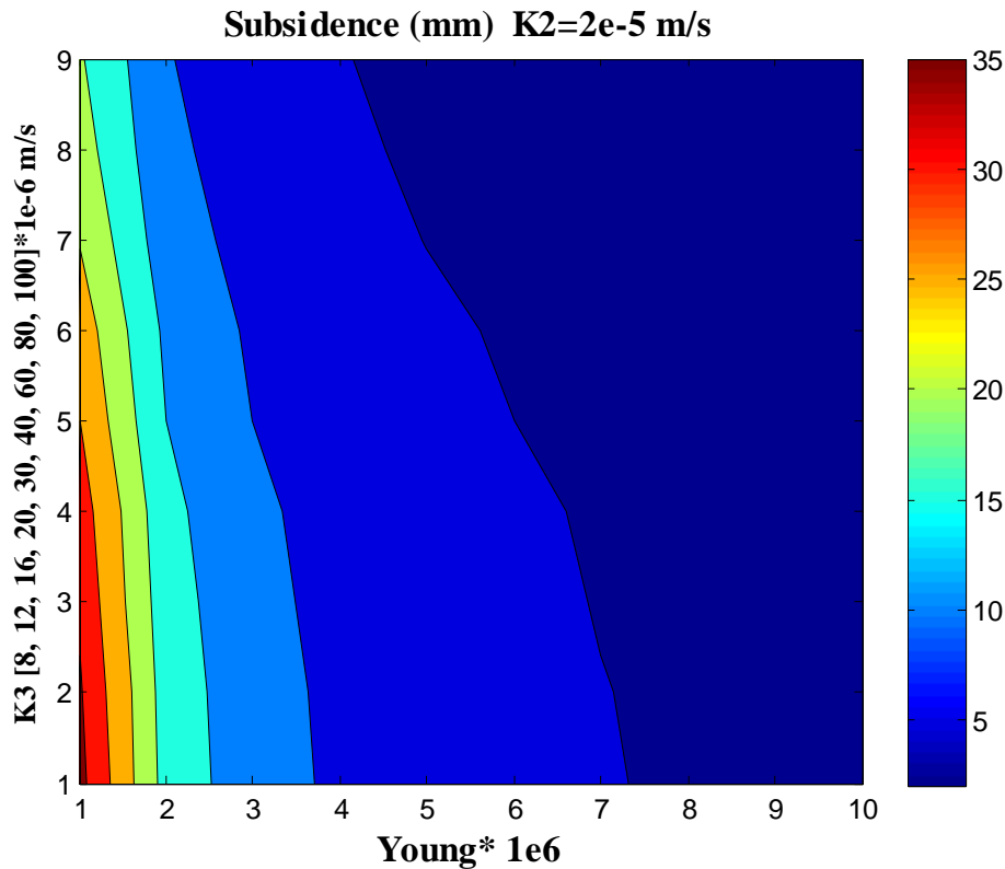
Figure 6.21 : Variation de la subsidence en (mm) en fonction du rapport K3 et du module d'Young en (Pa), pour une conductivité K2 fixée.
