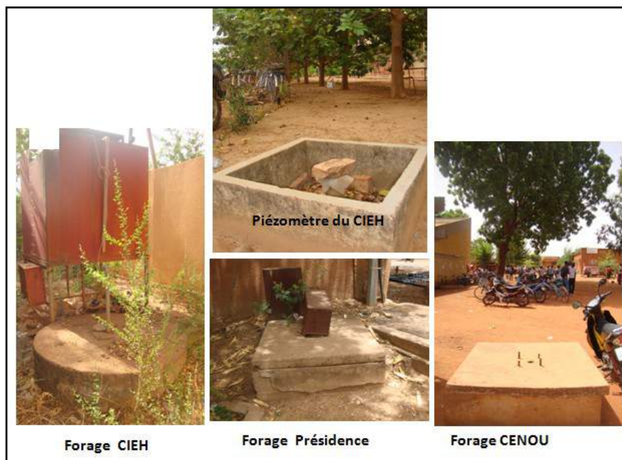
Figure 1. 13: Etat actuel des ouvrages piézométrique de l'université.
