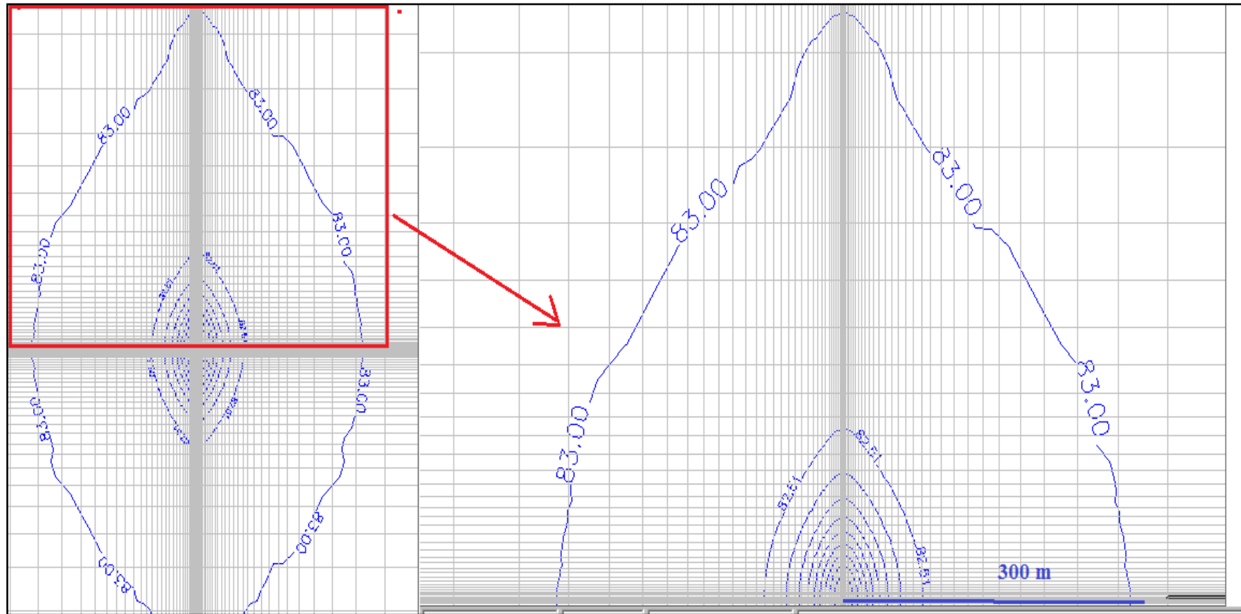
Figure 6. 15 : Anisotropie des isopièzes pour un pompage au sein d'une faille. L'allongement des isopièzes est suivant la direction de la faille.
