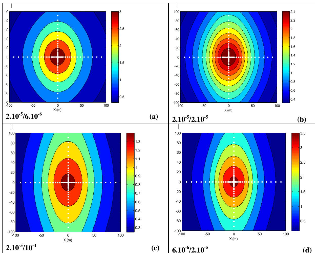
Figure 6. 18 : Rabattement en fonction du rapport ( K_2/K_3 ) des conductivités de la couche basale des altérites et celle de la faille. Les conductivités sont exprimées en m/s et le rabattement en m.
