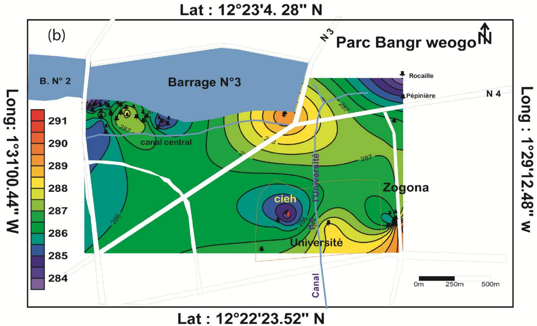
Figure 3. 9 : Cartes piézométriques de la zone d'étude à Ouagadougou: (a)Octobre 2013; (b) Avril 2014.
