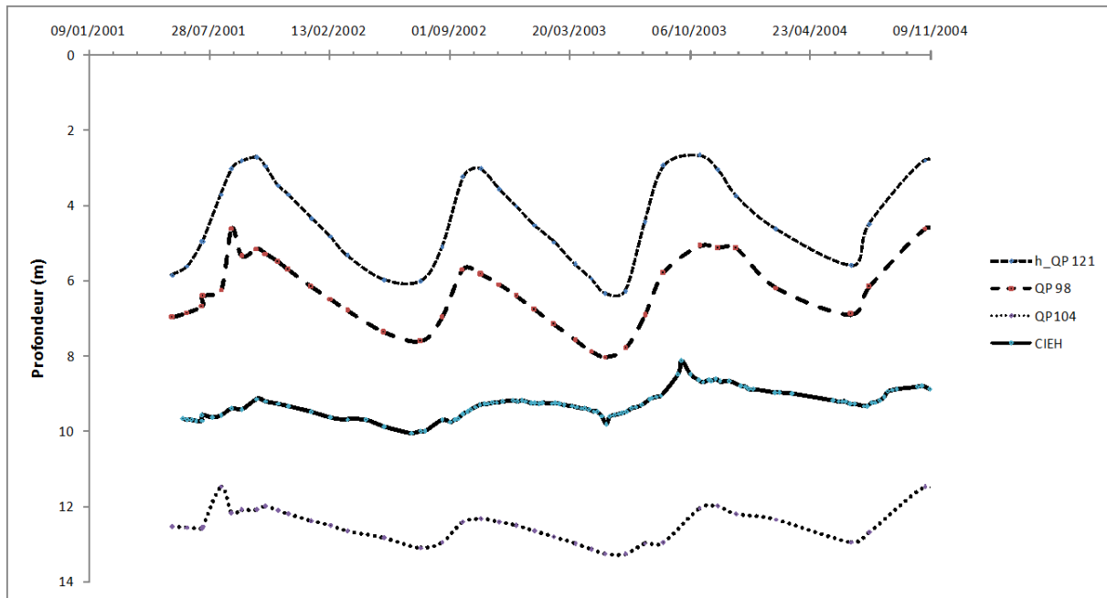
Figure 3. 8 : Variation des niveaux piézométriques des forages QP 98, 104 et 121 au sein de la ville de Ouagadougou entre de 2001 à 2004 (d'après Yameogo 2008) comparées à celles enregistrées au CIEH.
