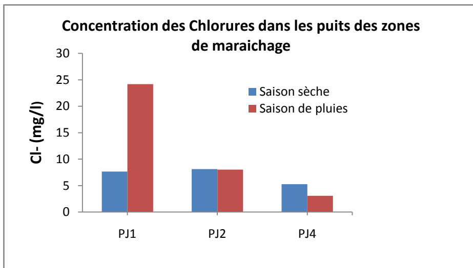
Figure 5. 6 : Représentation graphique des concentrations en chlorures dans les eaux des puits de la zone de maraîchage.
