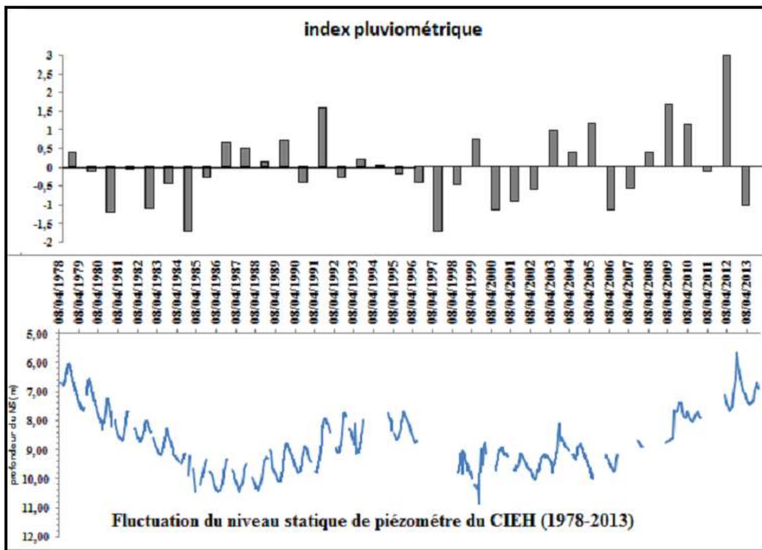
Figure 3. 6 : Variation du niveau statique du piézomètre du CIEH comparées avec l’index pluviométrique calculé sur la période 1978 – 2013.
