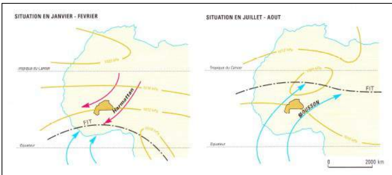
Figure 3. 5 : le déplacement du FIT en Afrique de l'Ouest (source : Laclavère 1993).
