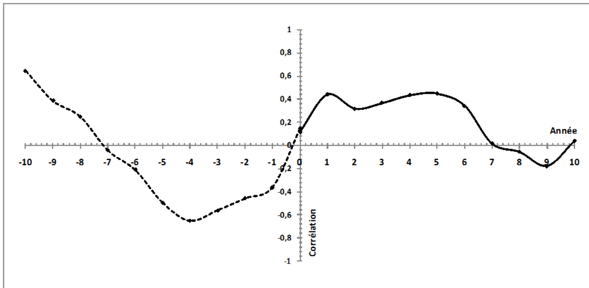
Figure 3. 12 : Corrélogramme croisé entre précipitation et niveau moyen du piézomètre du CIEH.
