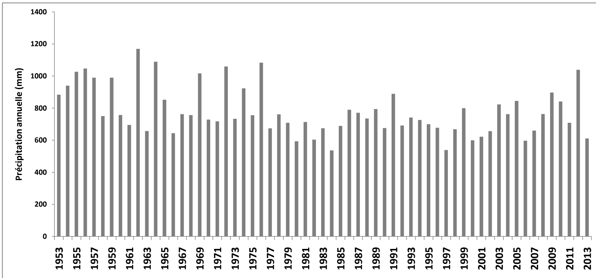
Figure 3. 2 : Précipitations annuelles à Ouagadougou (1953 – 2013).
