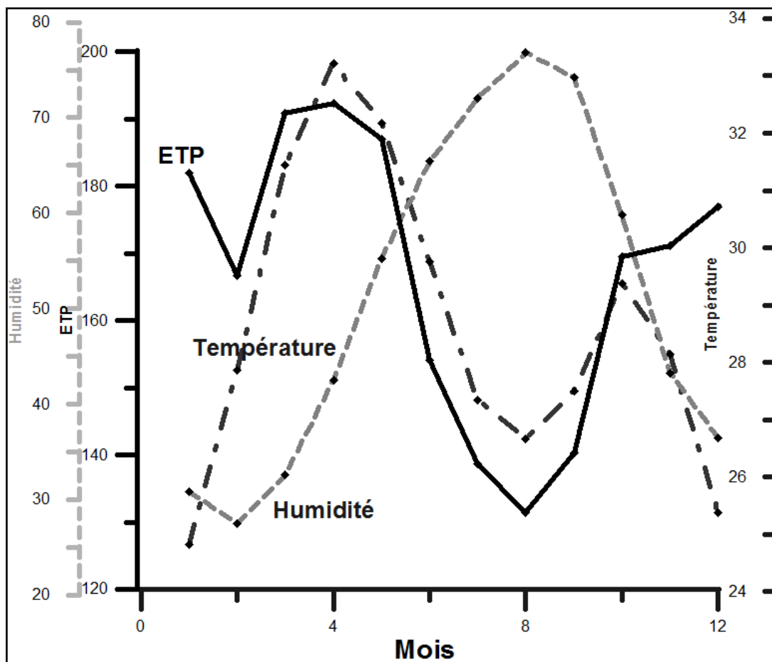
Figure 3. 4 : Variation mensuelle de la température (période : 1978 - 2012), de l'ETP (période : 1978 - 1990) et de l'humidité relative (période : 1961 - 1978) à Ouagadougou.
