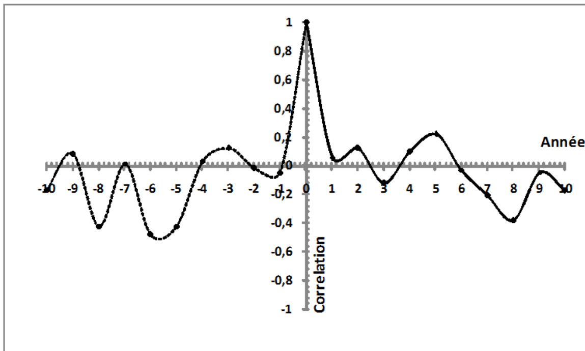
Figure 3.10: Autocorrélation des précipitations.
