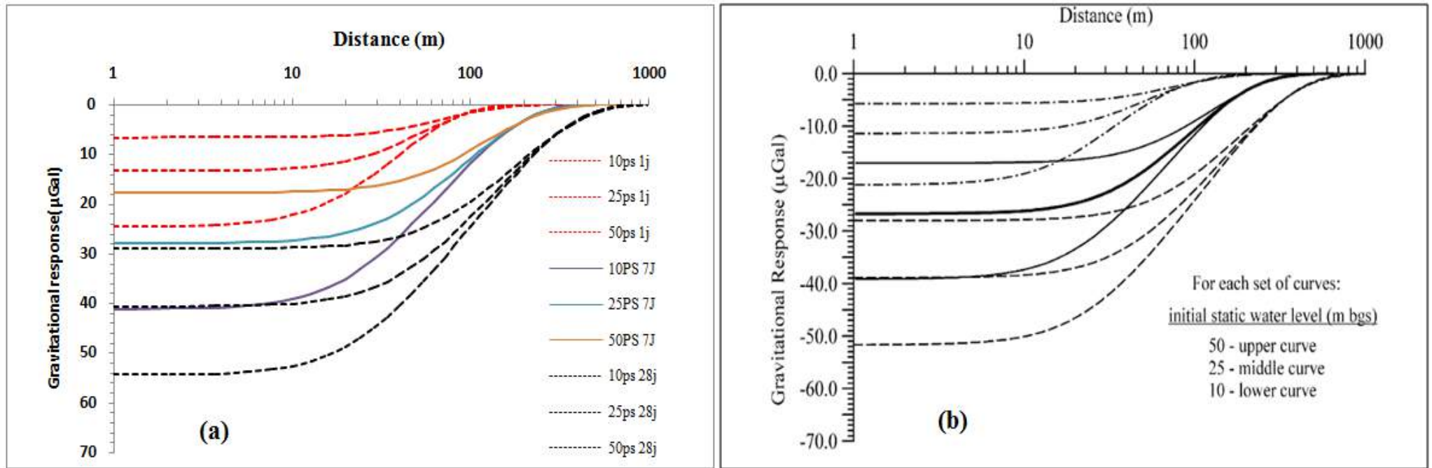
Figure 6. 9 : Comparaison des signaux gravimétriques obtenus Damiaty (2006) (b) et au cours de cette étude (a). Les trois séries de courbes correspondent à un pompage durant 1 jour, 7 jours et 28 jours, avec un niveau statique initial à 10 m 25 m et 50 m sous la surface du sol.
