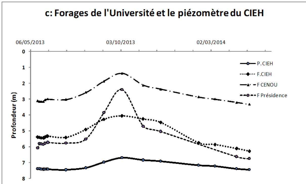
Figure 3.7 : Variations piézométriques sur l'année 2013 - 2014 dans trois parties de notre zone d'étude. a) la zone de Zogona : puits PP1,...PP7 ; b) le site de l'université : piézo CIEH, forage CIEH, forage Cenou et forage Présidence ; c) le parc Bangr Weogo: puits Rocaille et Pépinière. Pour chaque sous figure l'échelle verticale (hauteur piézométrique) est différente et le piézomètre du CIEH est figuré, à titre de comparaison.
