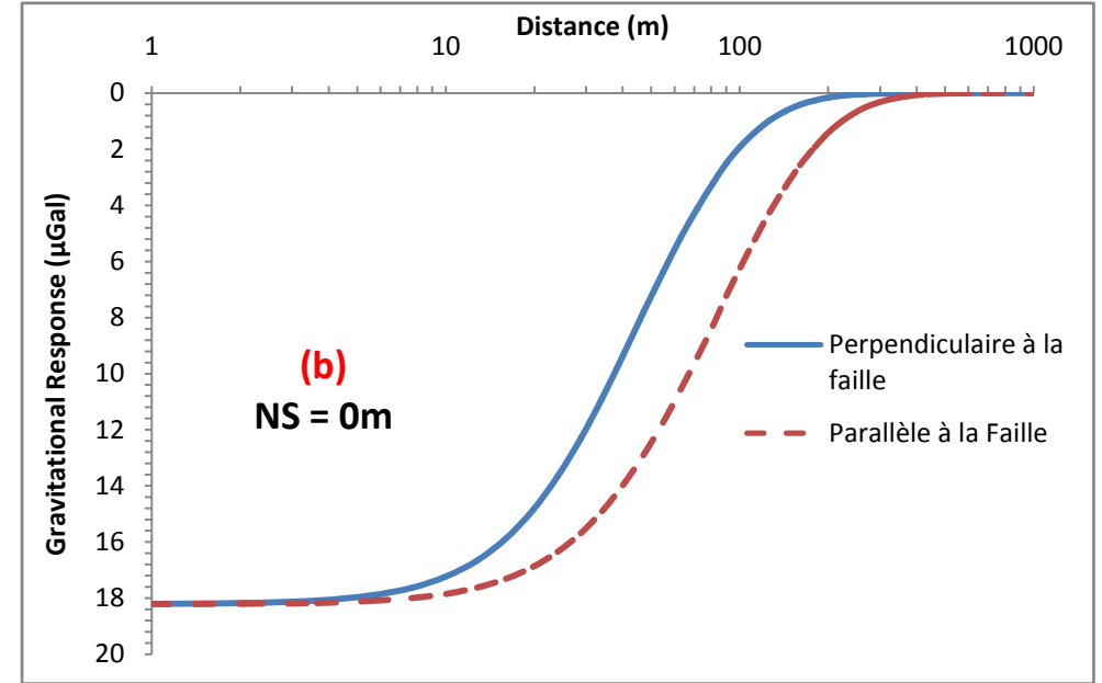
Figure 6. 17 : Courbes des signaux gravimétrique pour des pompages dans la faille avec différents niveaux statiques initiaux. A gauche, niveau statique 7 m; à droite niveau statique 0 m.
