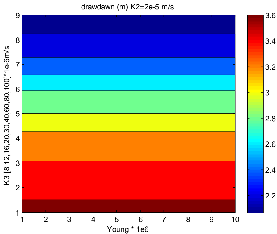
Figure 6. 19 : Variation du rabattement en fonction de K_3 , pour une valeur de K_2 fixée. Le rabattement est en mètres.
