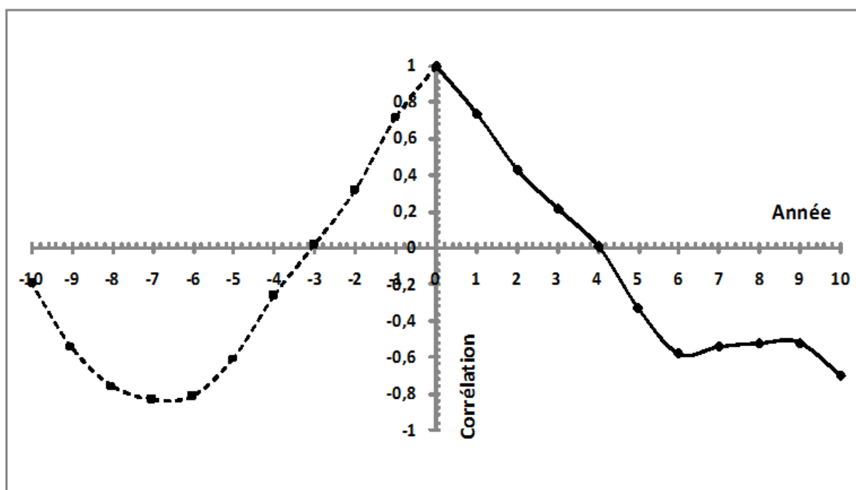
Figure 3.11 : Autocorrélation du niveau moyen du piézomètre du CIEH.
