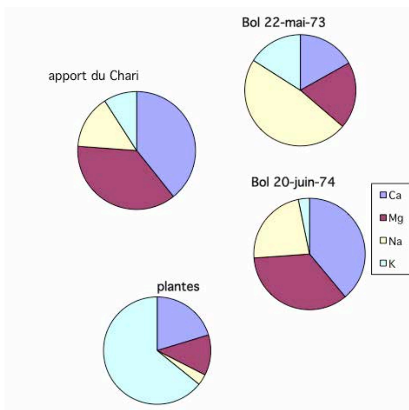
Figure 1 – Composition en ions majeurs (mg/L) de l'apport moyen du Chari, de l'eau du Lac en phase de Moyen Tchad (exemple de Bol, 22 mai 1973, conductivité 400 microSiemens) et en phase de Petit Tchad (Bol, 20 juin 1974, conductivité 400 microSiemens) en présence d'une forte densité de plantes aquatiques dont la composition est indiquée dans le graphique plantes (données Lemoalle).
