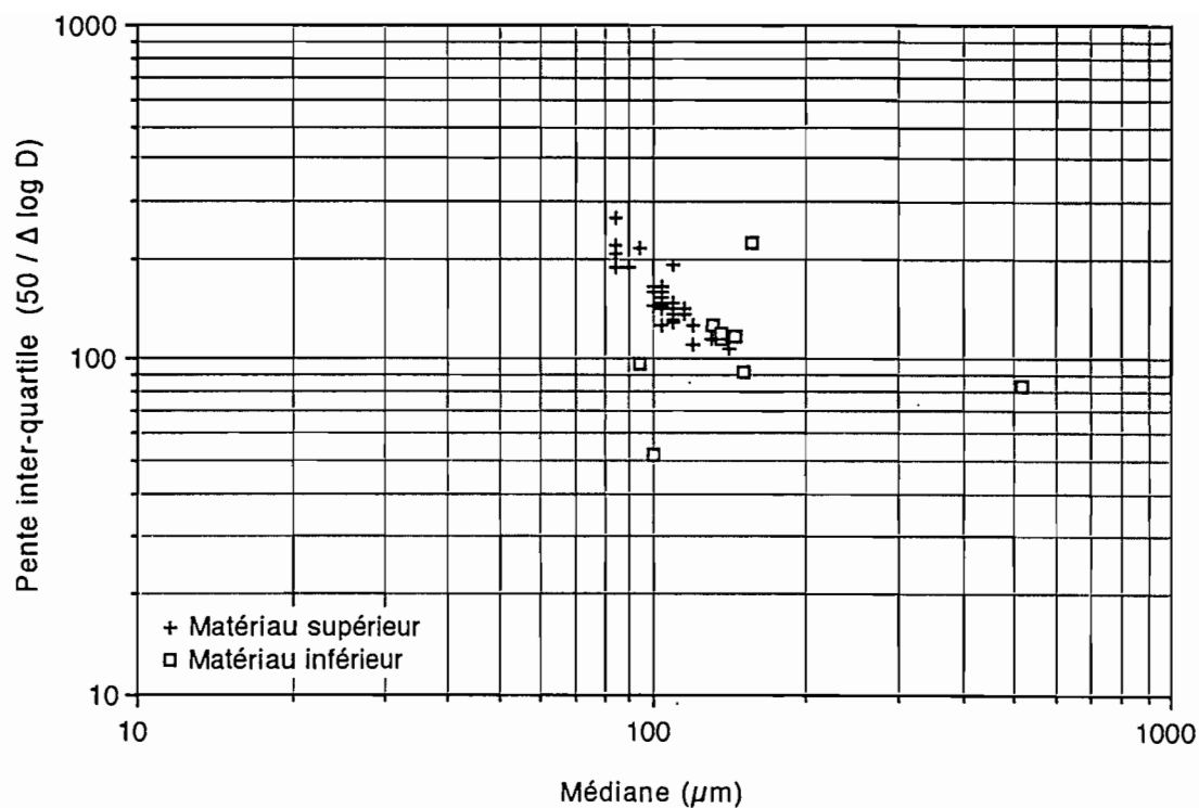
Figure VI.8 Caractérisation des matériaux sédimentaires. Variation de la médiane et de la pente inter-quartile pour les particules supérieures à 50 \mu\text{m}
