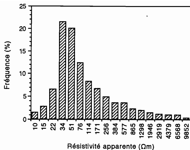
Figure V.8 Distribution des valeurs de résistivité apparente pour l'ensemble des mesures en 1 m, 2 m, 4 m et 8 m
