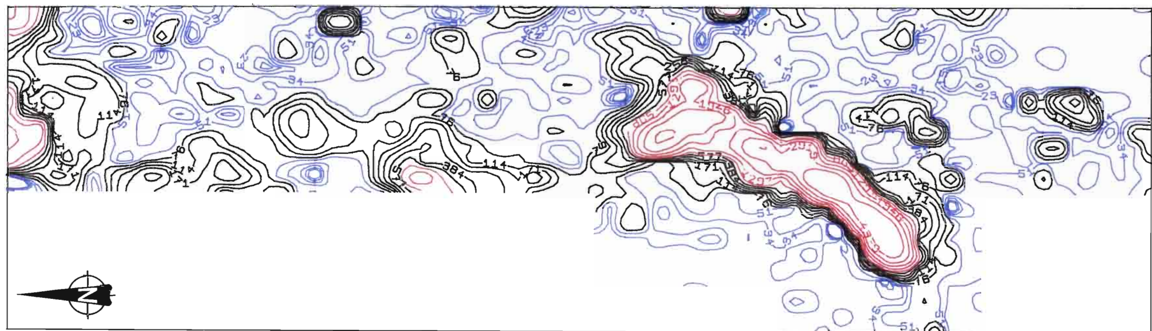
Carte de résistivité apparente en a = 2 m
