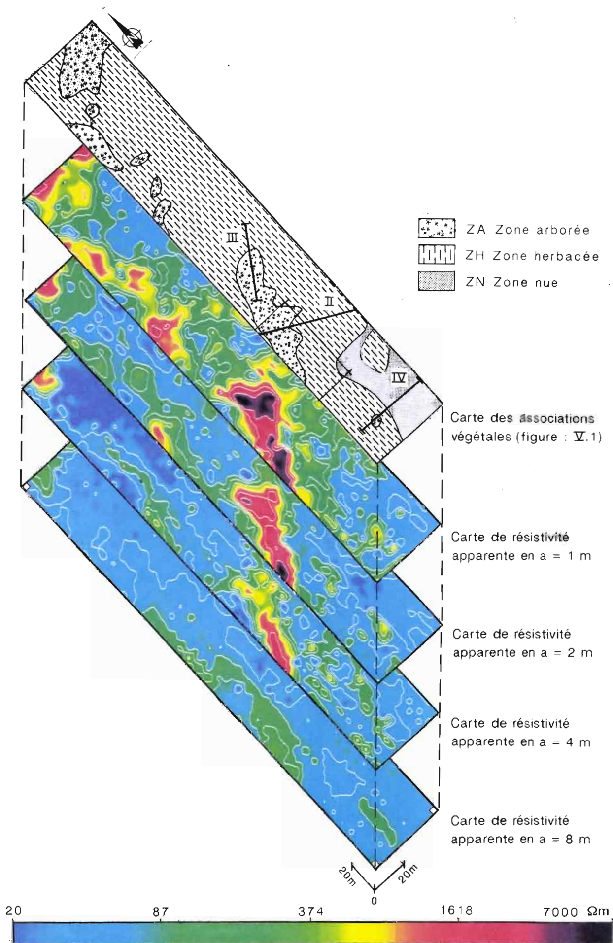
Figure V.10 Cartes de résistivité apparente en 1 m, 2 m, 4 m et 8 m et localisation des séquences II, III et IV sur un extrait de la carte des associations végétales (figure V.1)
