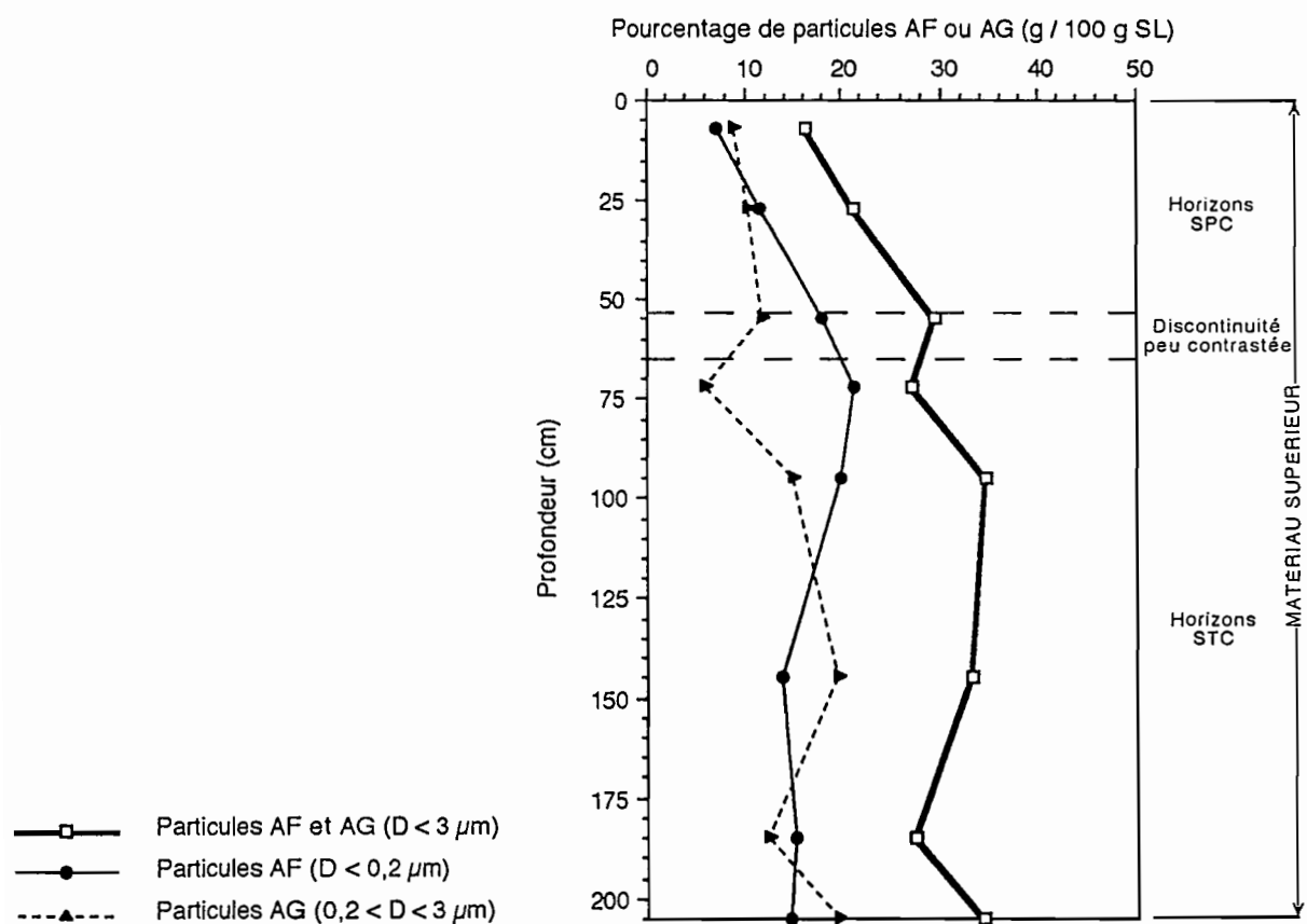
Figure VI.13 Variation de la teneur en AF ( D < 0,2 \mu\text{m} ) et en AG ( 0,2 < D < 3 \mu\text{m} ) rapportée à 100 g de SL ( 3 < D < 500 \mu\text{m} ). Cas d'un sol à discontinuité de cohésion peu contrastée (fosse B, localisation sur la figure VI.2)
