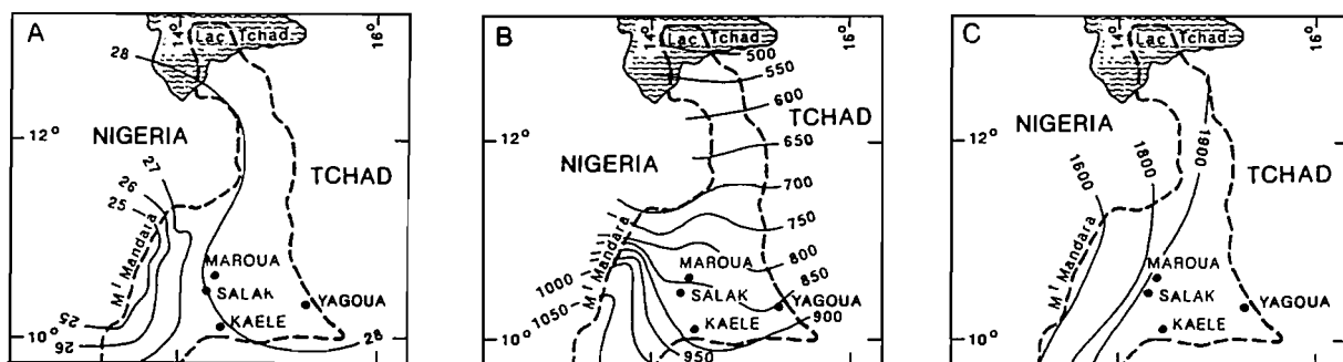
Figure 1.7 Variations géographiques (A) de la température moyenne annuelle (d'après SUCHEL, 1988), (B) de la pluviosité moyenne annuelle (d'après BRABANT et GAVAUD, 1985) et (C) de l'évapotranspiration ETc [TURC] (d'après JEGADEN-SANTIAGO et SUCHEL, 1990)
