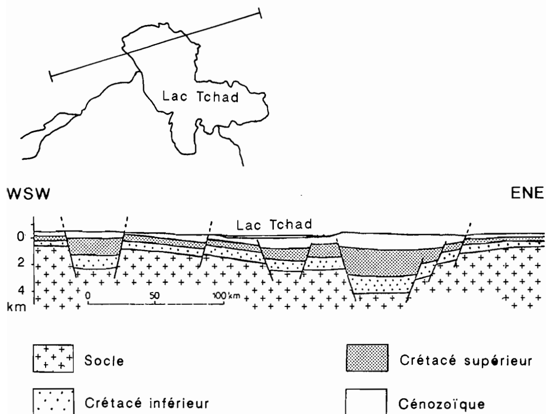
Figure I.9 Coupe montrant la structure du bassin tchadien (d'après POUCKET et DURAND, 1984)
