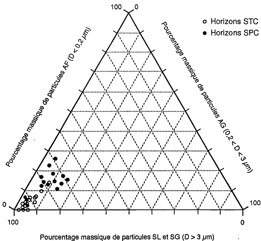
Figure VI.11 Constitution granulométrique des horizons SPC et STC développés au sein du matériau supérieur
