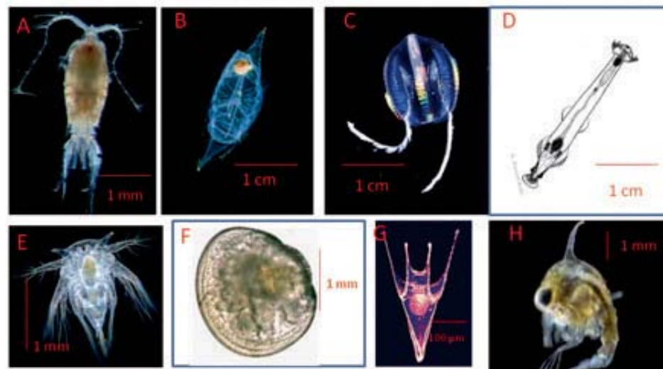
Quelques exemples d'organismes du métazooplancton. En haut holoplancton : (A) copépodes ( Rhincalanus sp.), (B) salpe ( Salpa fusiformis ), (C) Pleurobrachia pilaueus (groseille de mer), (D) Chaetognathes ( Sagitta sp.). En bas méroplancton (larves du plancton) : (E) nauplius de balane, (F) larve de bivalve, (G) larve pluteus d'oursin, (H) larve zoé de crabe
