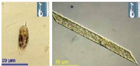
De gauche à droite, de haut en bas : Amphidinium longum , Oxytoxum sp., Prorocentrum gracile , Rhizosolenia imbricata . © Benoit Véron Université de Caen Basse Normandie
